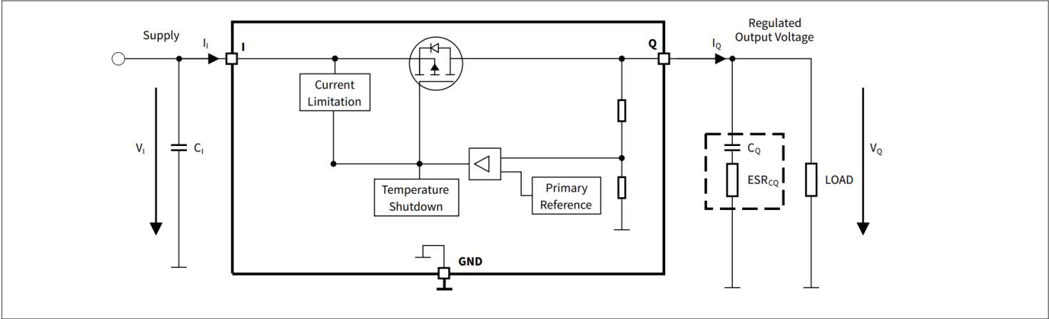
图 3 稳压器电路的功能框图
