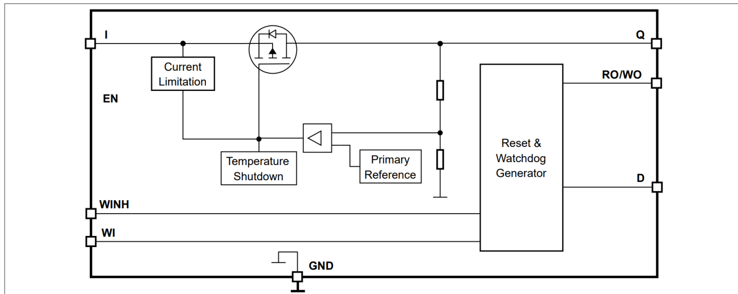
图 1 框图
