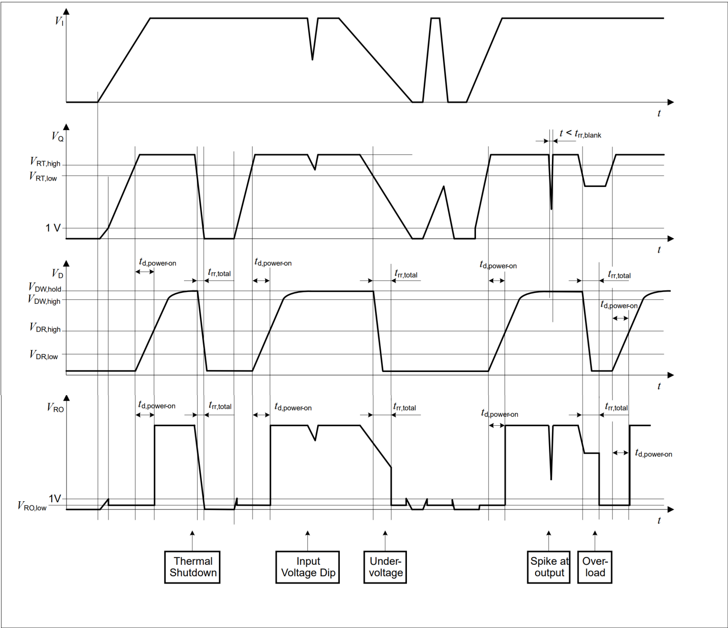
图 6 复位时序图
