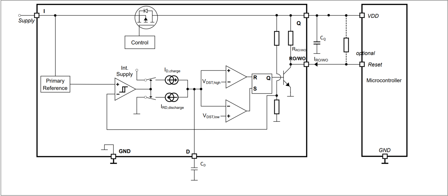
图 7 复位功能框图
