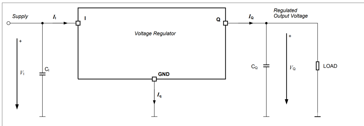
图 5 参数定义
