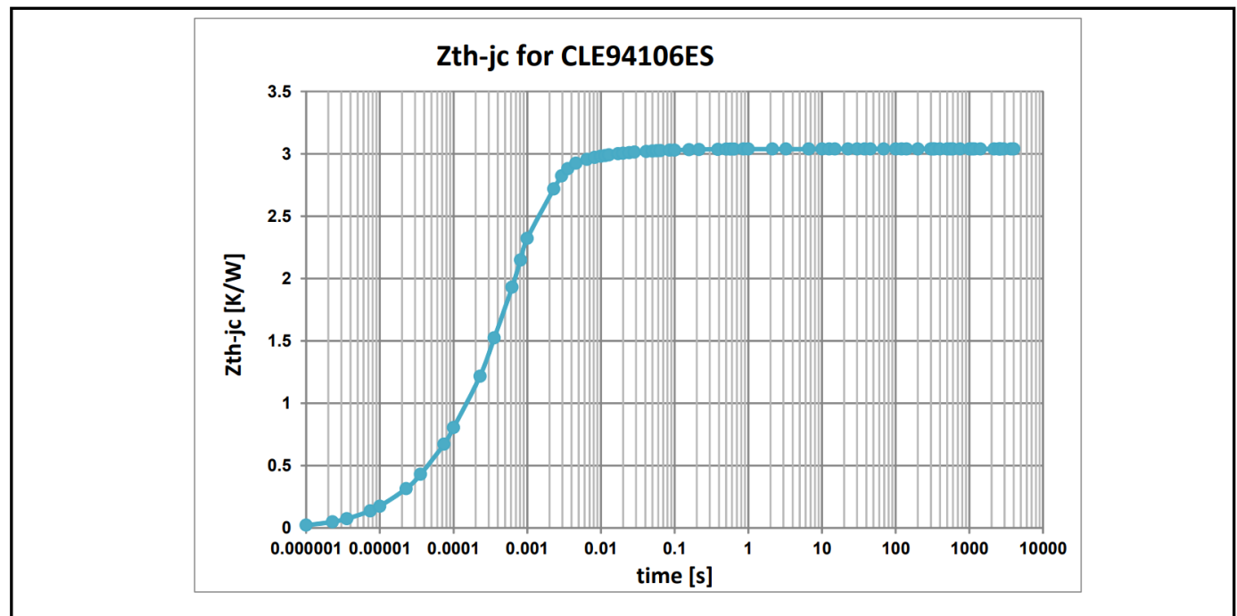
图 30 ZthJC 曲线
