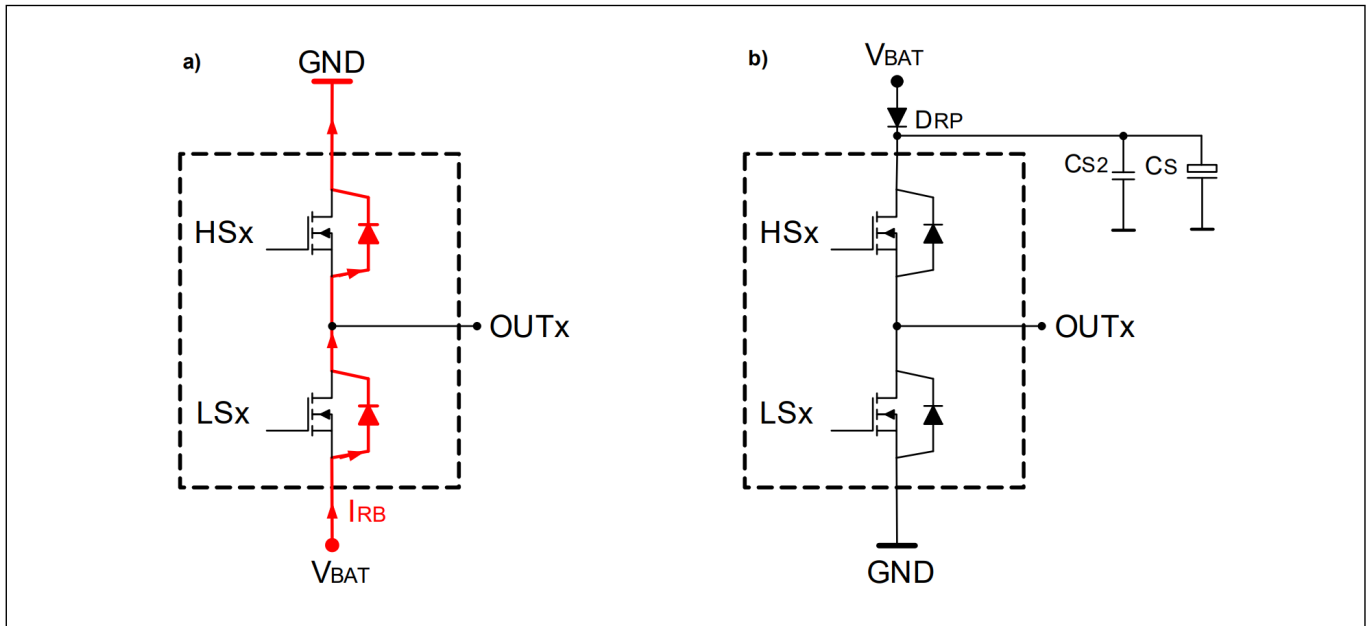
图 4 反极性保护
