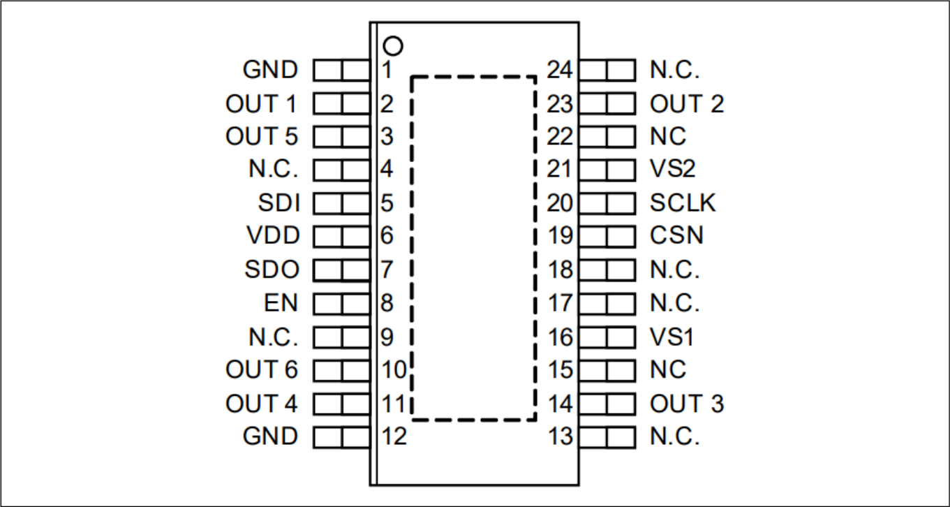
图 1 CLE94106ES 引脚配置
