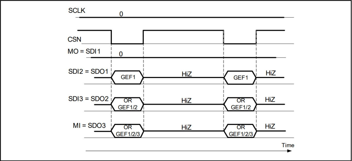
图 22 仅由 CLE941xy 器件组成的菊花链中具有零 SCLK 时钟周期的全局错误标志
