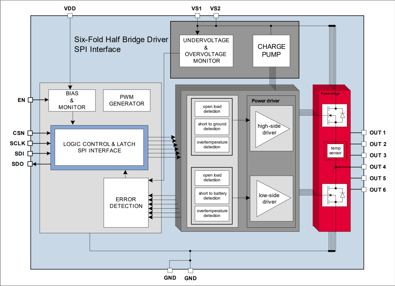
图2 CLE94106ES框图（SPI接口）
