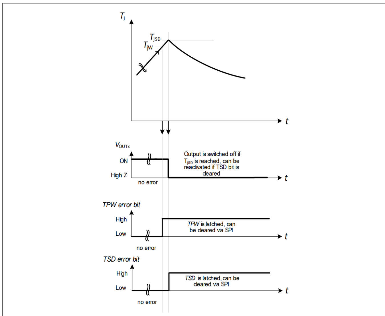
图 11 过温行为
