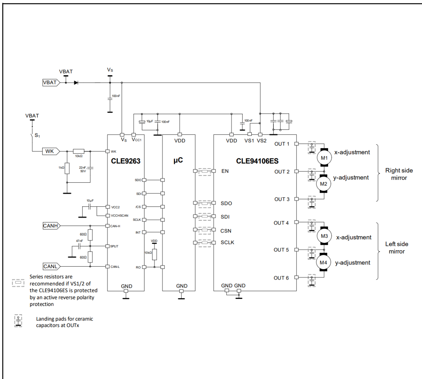
图 28 侧后视镜控制的应用示例
