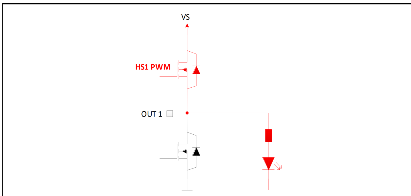
图 6 OUT 1 上的 PWM 操作
