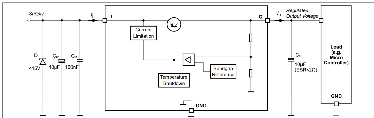
图3 应用框图
