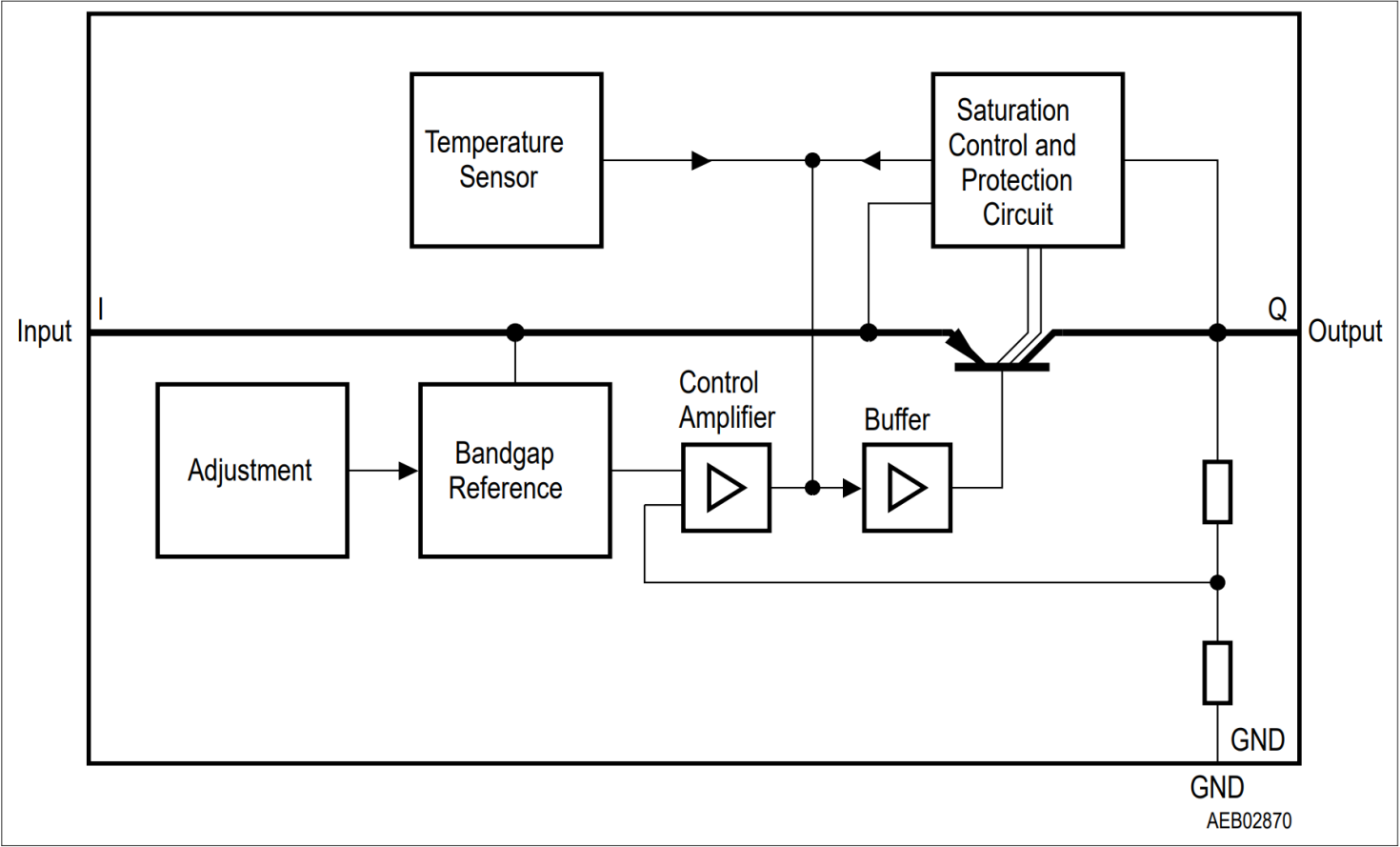
图 1 框图
