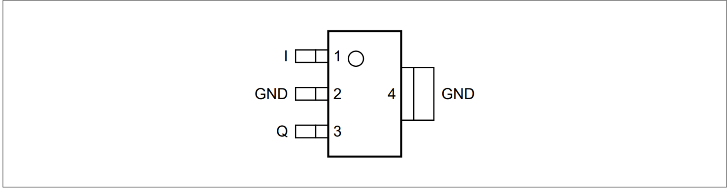
图 2 引脚分配
