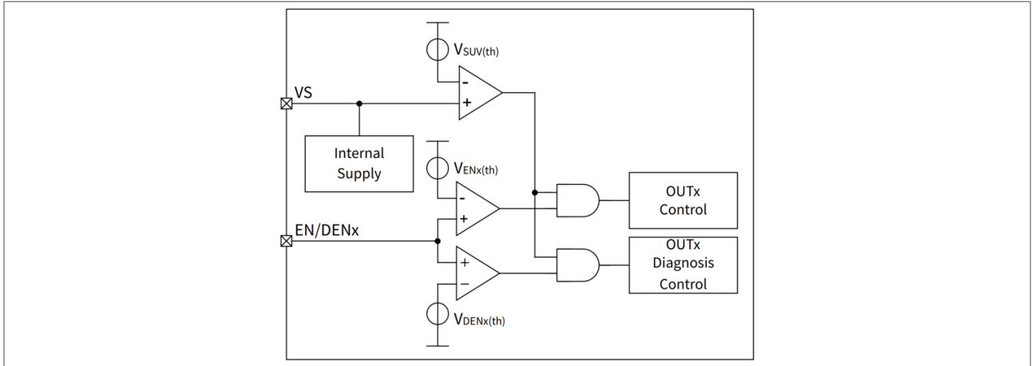
图 12 EN/DEN 框图
