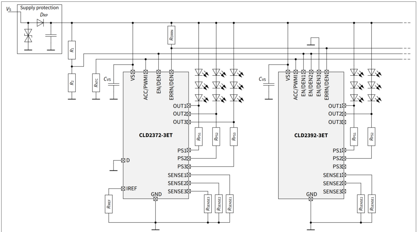
图 20 共享网络中 5 通道照明功能的应用图示例，具有“一错全开”故障管理和中央热降额功能
