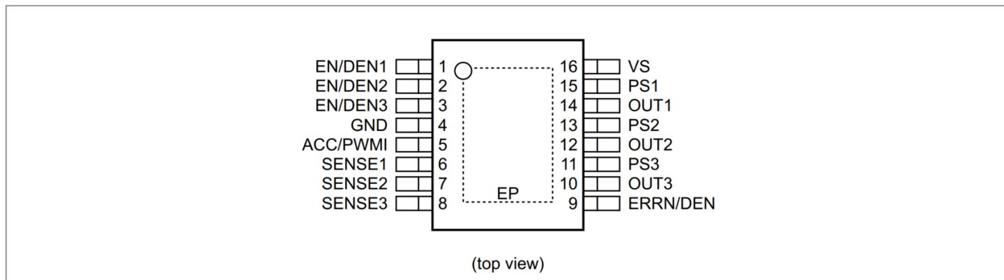
图3 PG-TFDSO-16 引脚配置
