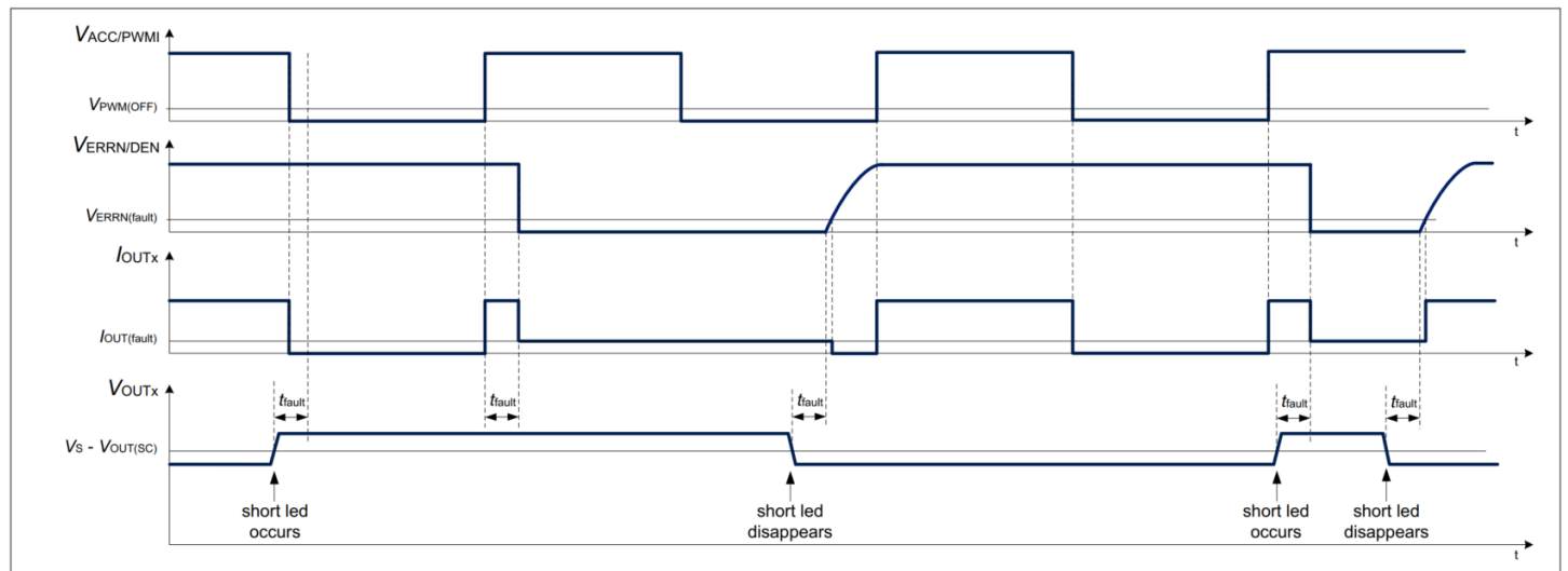
图 16 1-fail-all-ON 配置中的输出短路电源条件时序图示例
