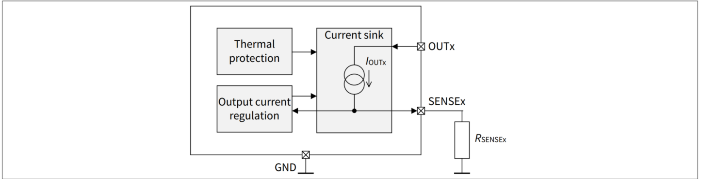
图 5 功率级框图
