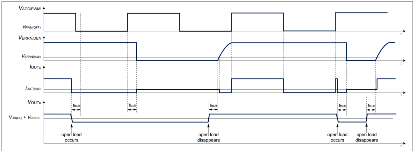
图 14 1-fail-all-ON 配置中的负载开路条件时序图示例
