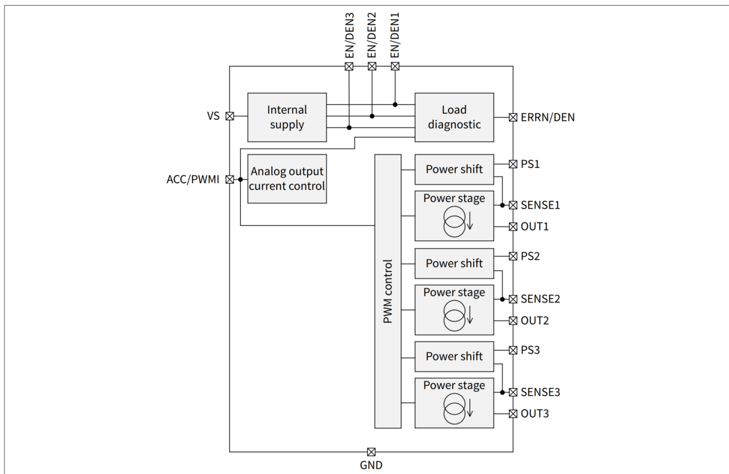
图2 CLD2392-3ET 框图
