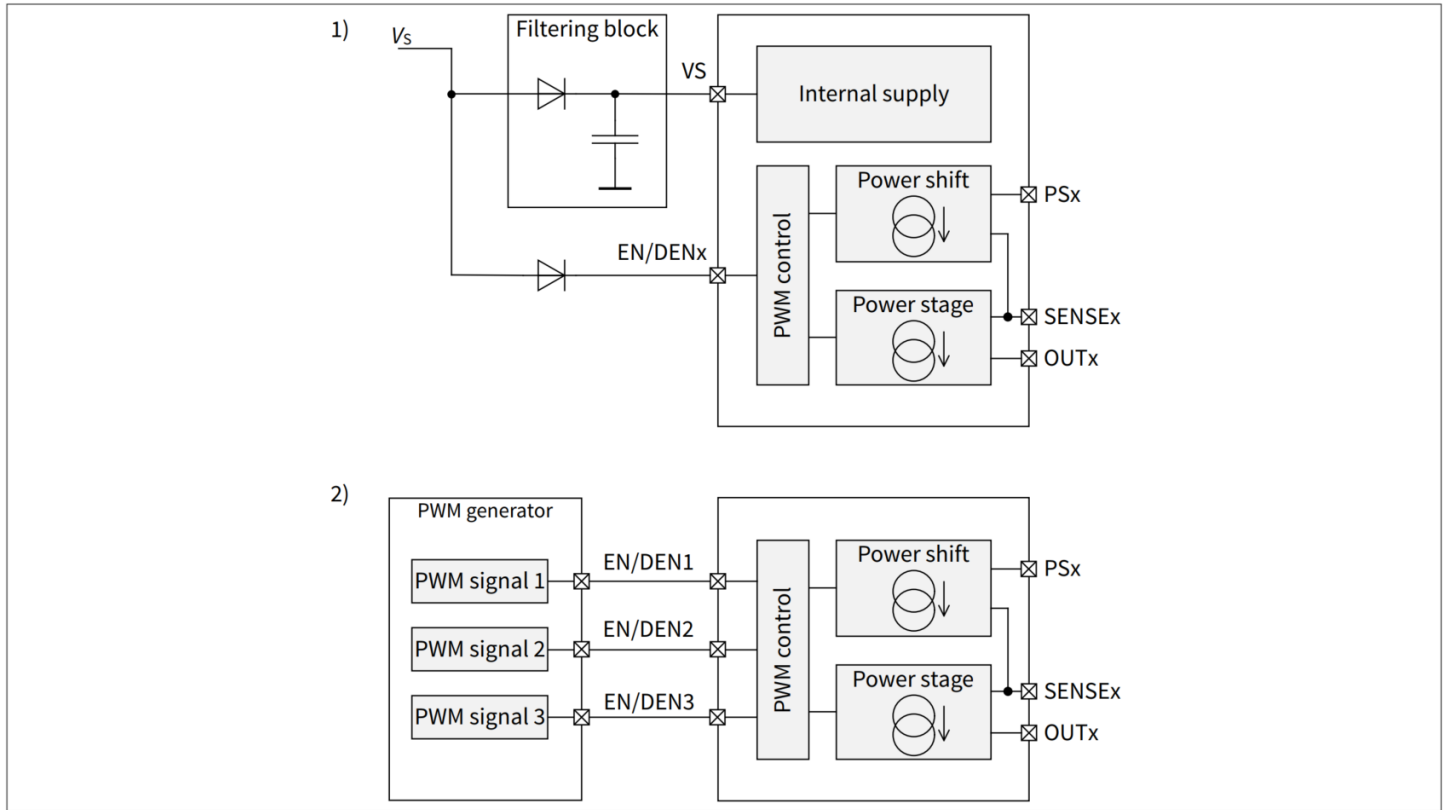
图 8 通过 EN/DENx 输入引脚进行 PWM 控制
