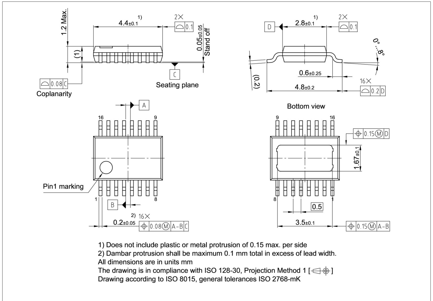
图 22 PG-TFDSO-16 封装外形 png
