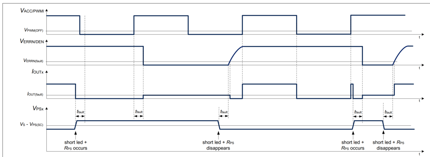
图 18 1-fail-all-ON 配置中的功率转移短路到供电条件时序图示例
