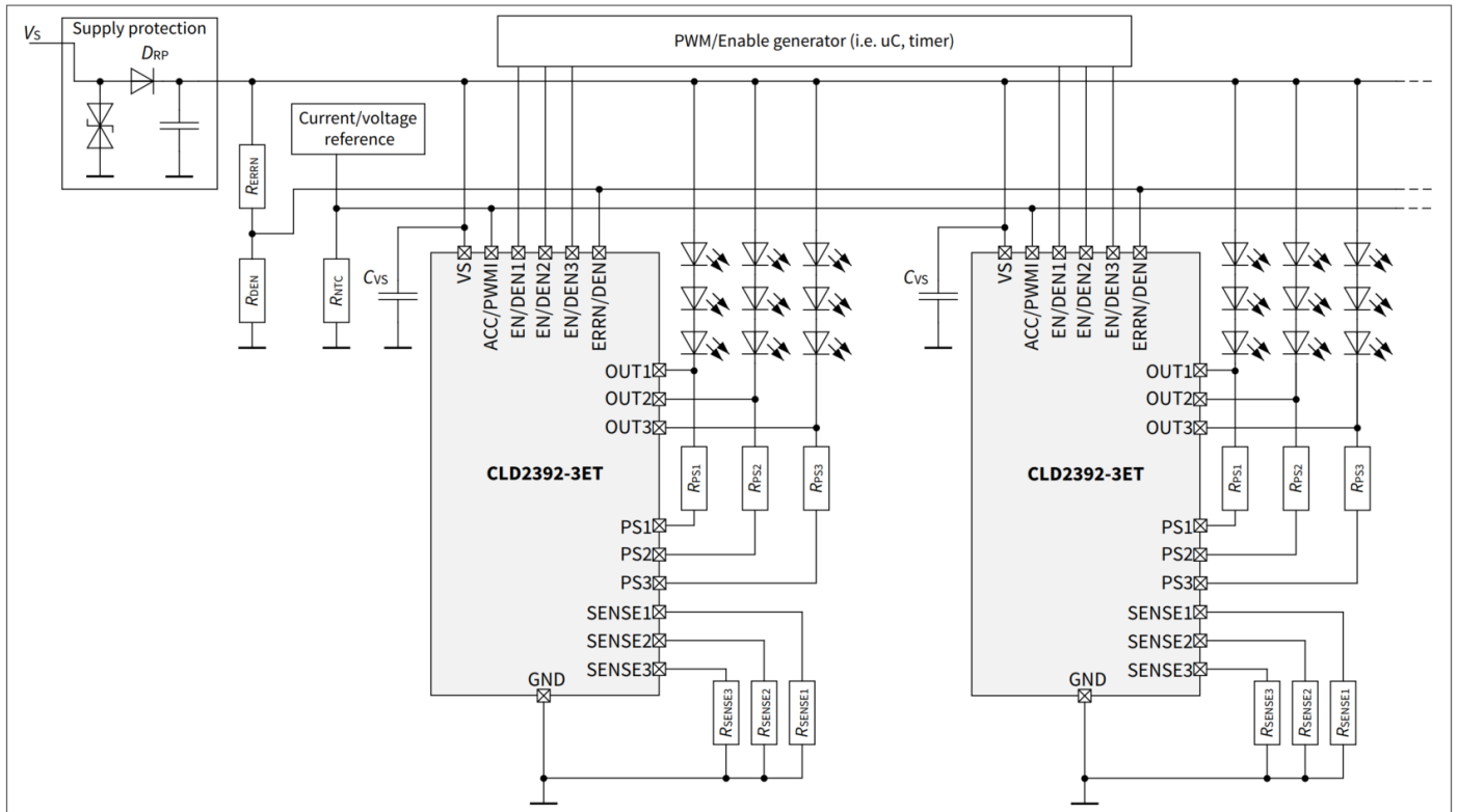
图 21 共享网络中动态照明功能的应用图示例，具有“一错全开”故障管理和中央热降额功能
