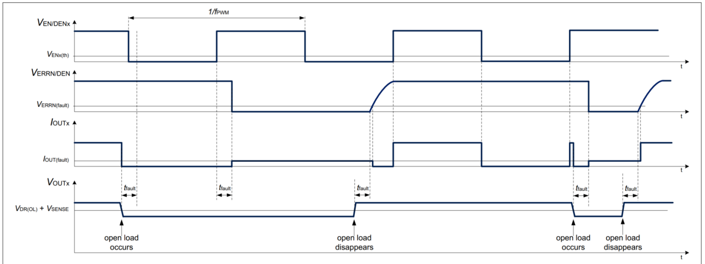
图 15 1-fail-all-ON 配置中的负载开路条件时序图示例，在 EN/DENx 引脚上应用数字调光
