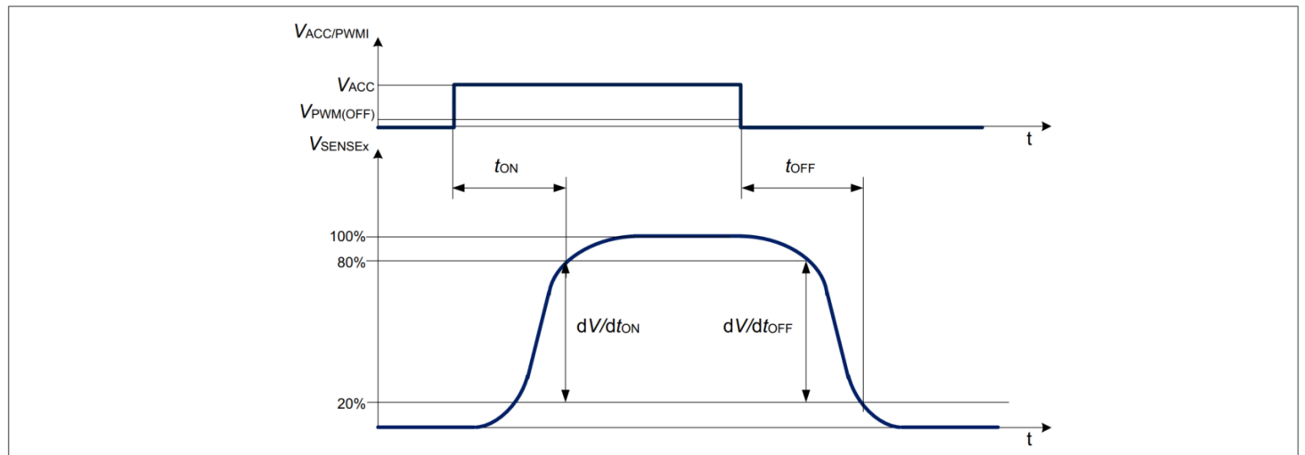
图 9 V_{ACC/PWMI} \geq 2.4 V 时的 PWM 控制时序图
