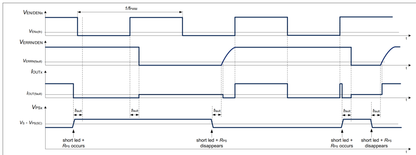
图 19 1-fail-all-ON 配置中的功率转移短路到供电条件时序图示例，EN/DENx 引脚上应用数字调光
