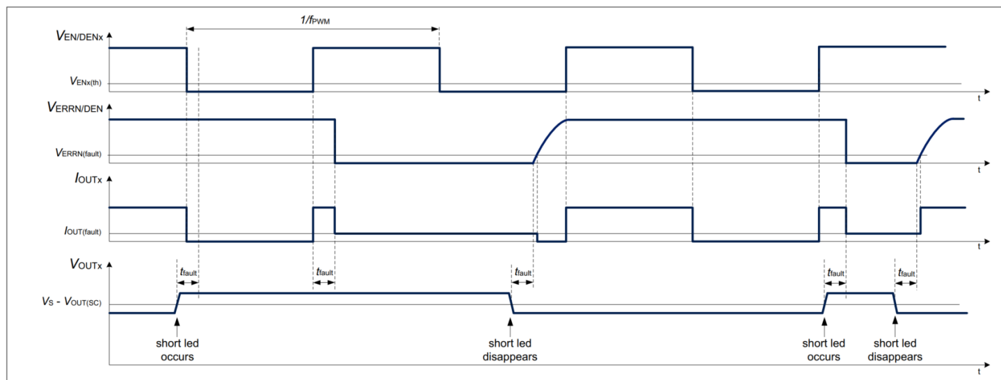
图 17 1-fail-all-ON 配置中的输出短路电源条件时序图示例,并在 EN/DENx 引脚上应用数字调光
