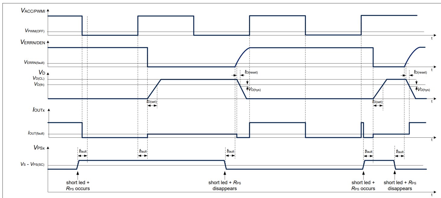
图 19 功率转移短路到供电条件图示例 1-fail-all-OFF 配置 (D 引脚开路或连接到外部电容器)
