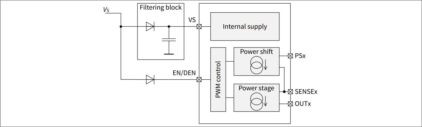
图 8 通过 EN/DEN 输入引脚进行 PWM 控制
