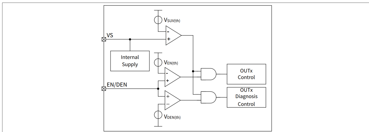
图 13 EN/DEN 框图
