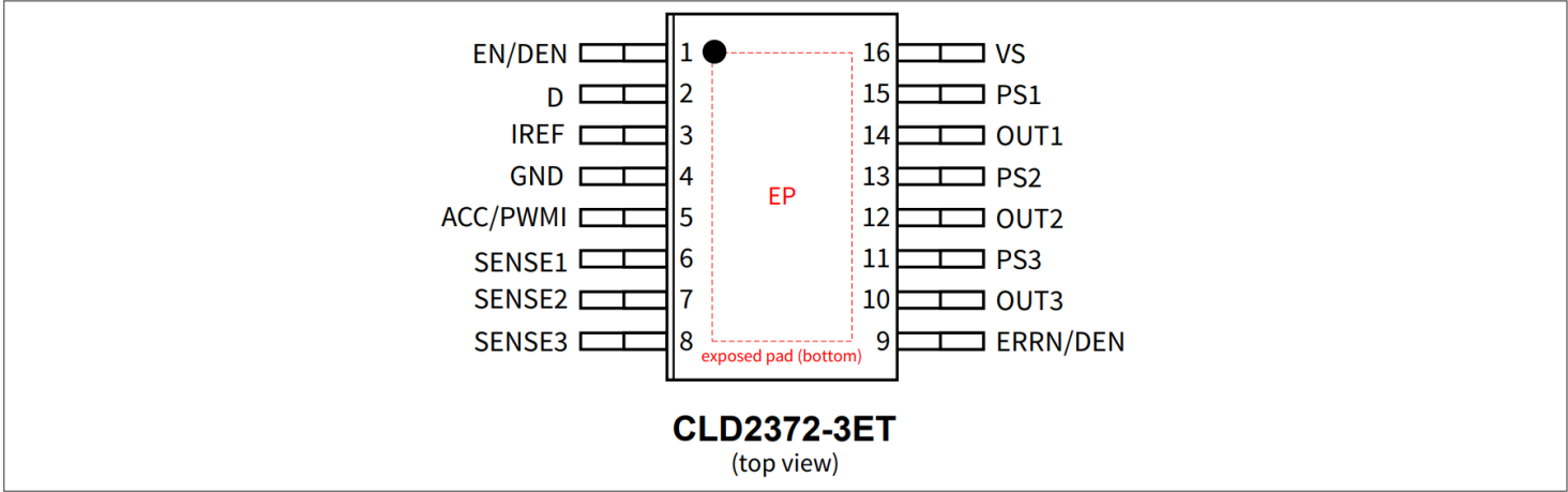
图3 PG-TFDSO-16 引脚配置
