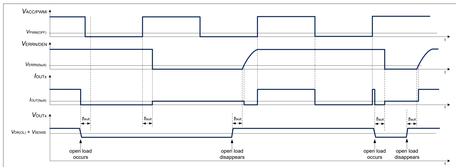
图 20 负载开路条件图示例 1-fail-all-ON 配置 (D 引脚短接到接地)
