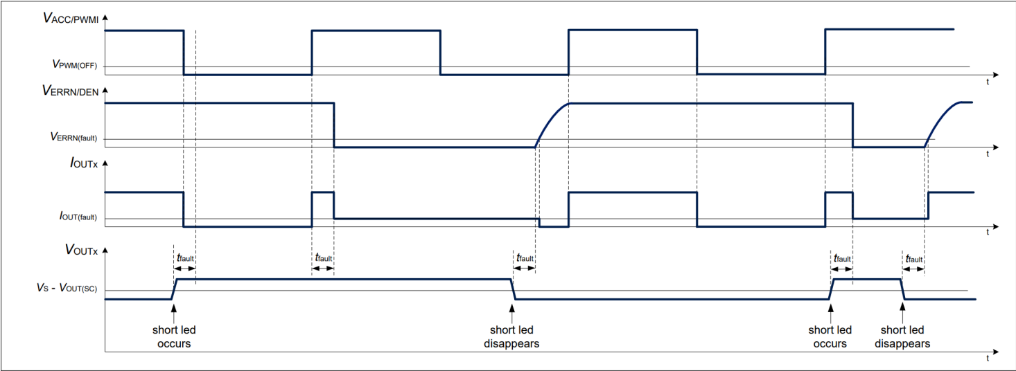
图 21 1-fail-all-ON 配置中的输出短路电源条件图示例（D 引脚对接地短路）
