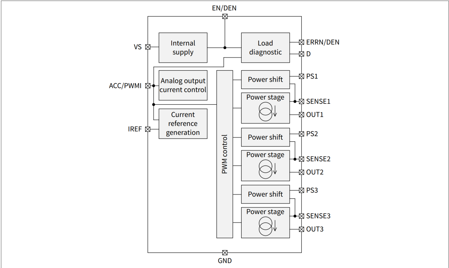
图2 CLD2372-3ET框图
