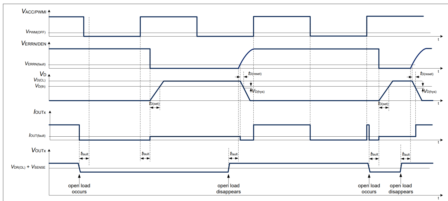
图 17 负载开路条件图示例 1-fail-all-OFF 配置（D 引脚开路或连接到外部电容器）
