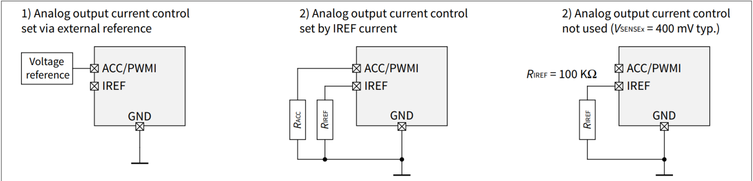
图 12 模拟输出电流控制配置
