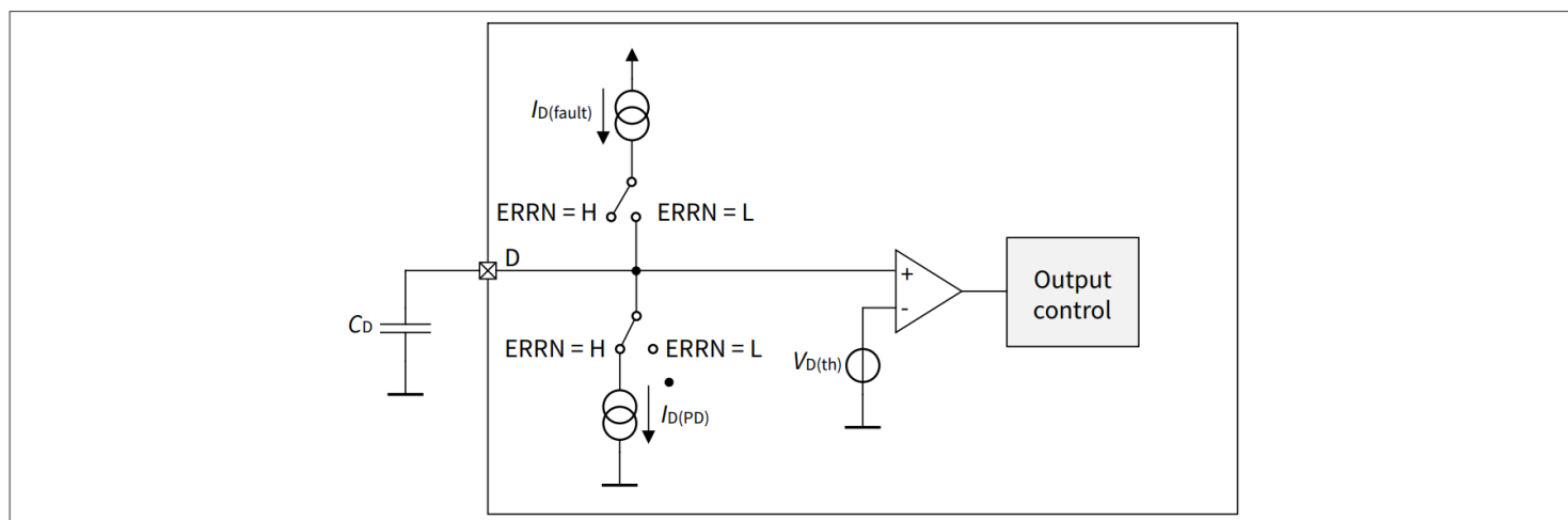
图 16 D 引脚（框图）
