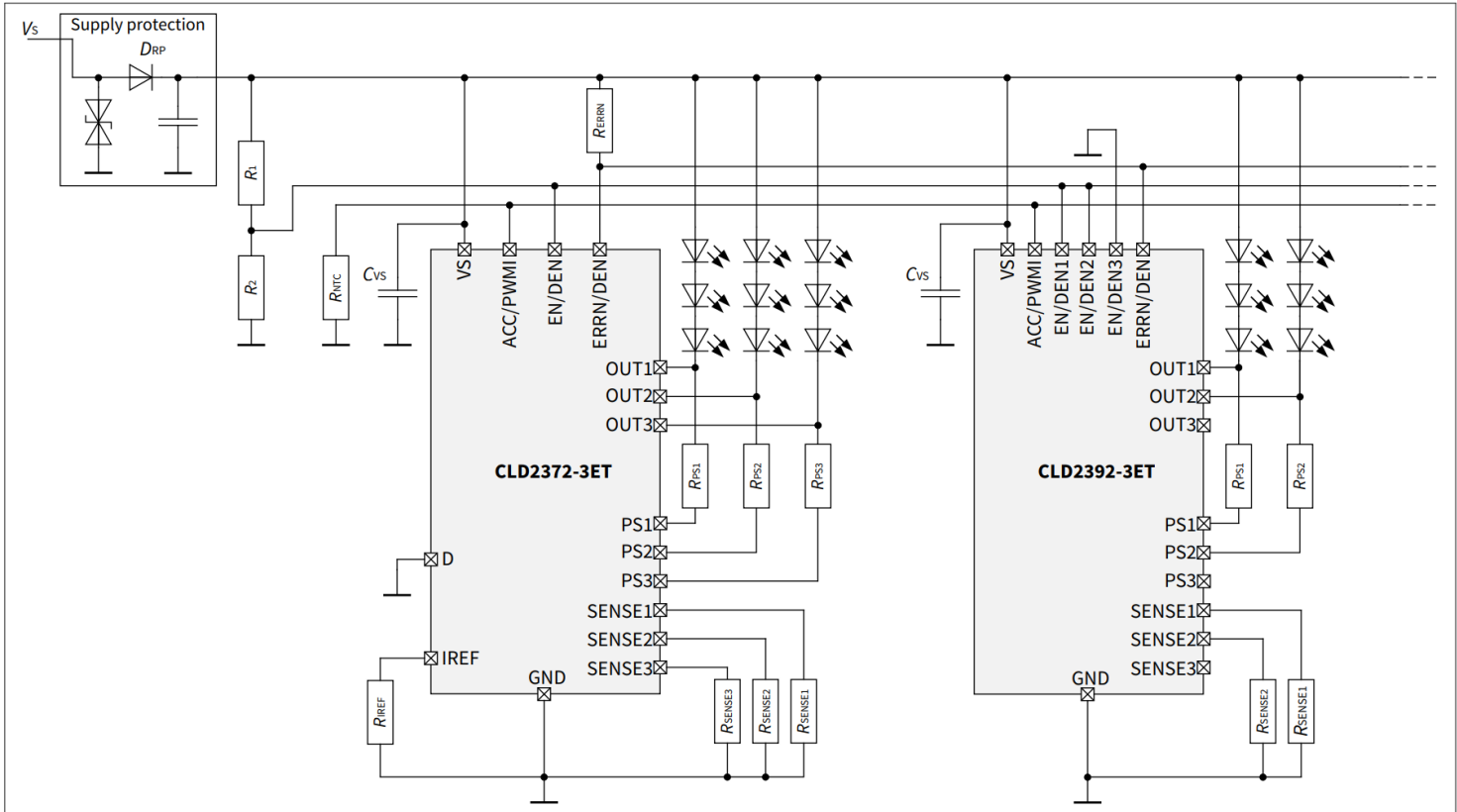
图 25 共享网络中 5 通道照明功能的应用图示例，具有“一错全开”故障管理和中央热降额功能
