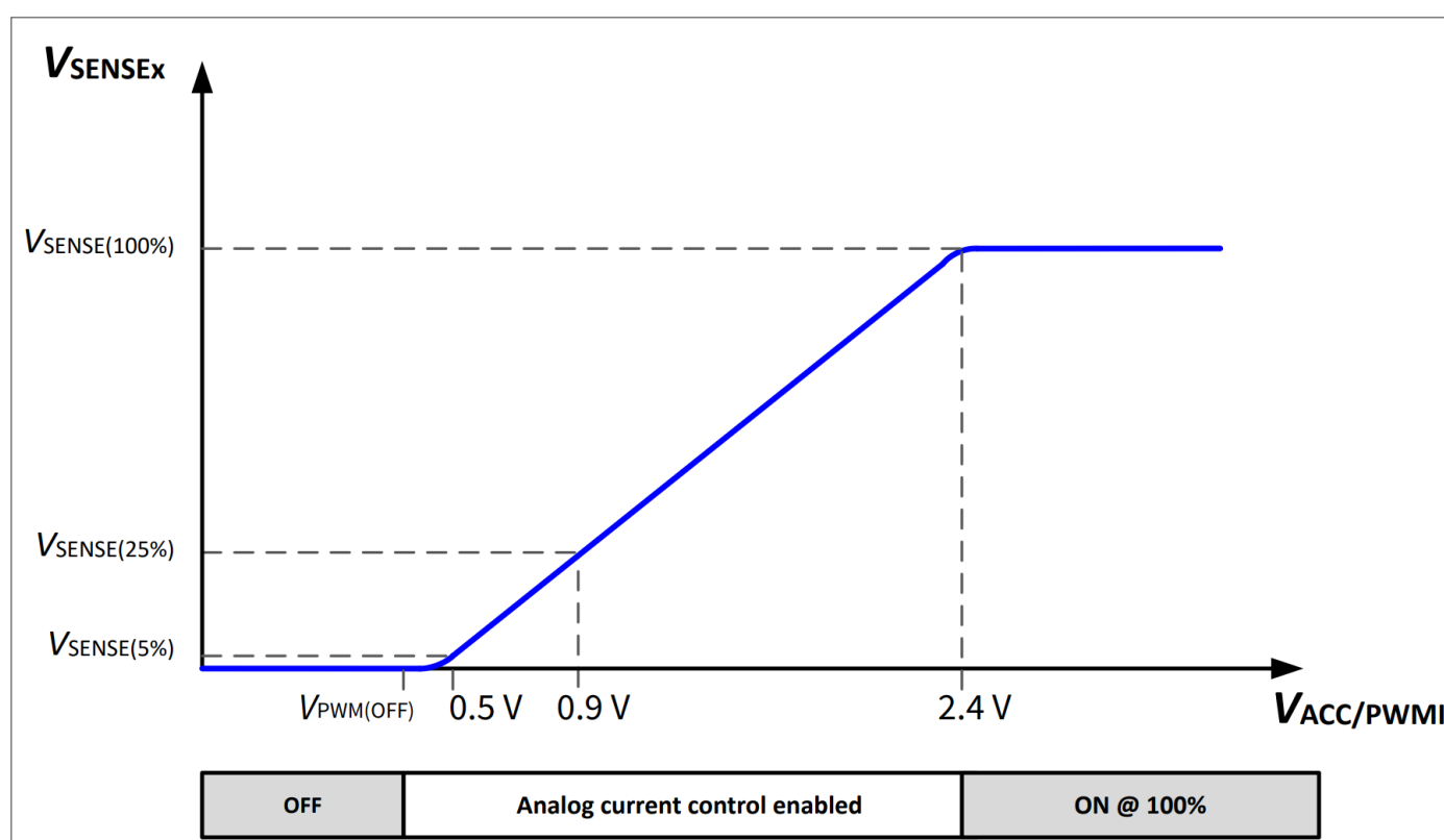
图11 模拟输出电流控制
