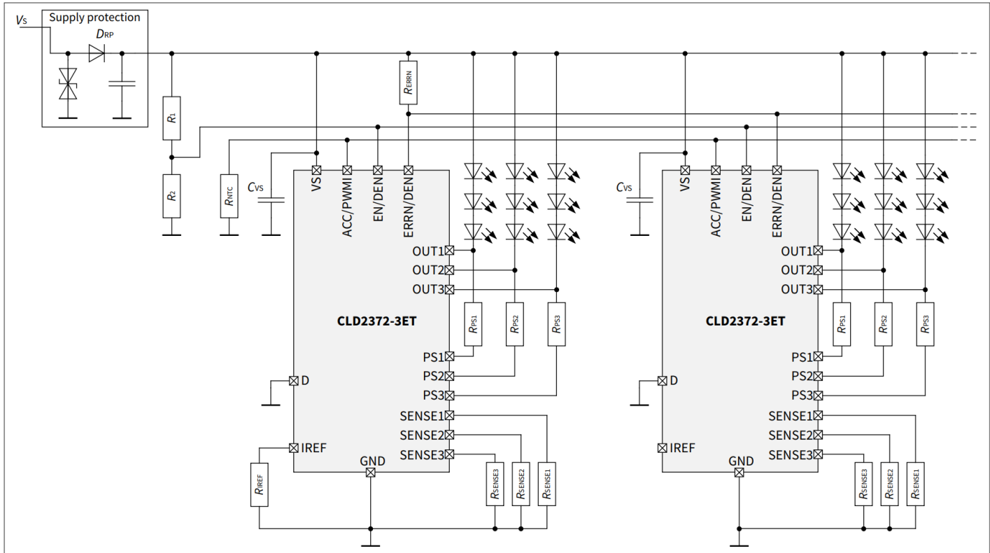
图 23 具有“一错全关”故障管理和中央热降额 的共享网络中的应用图示例
