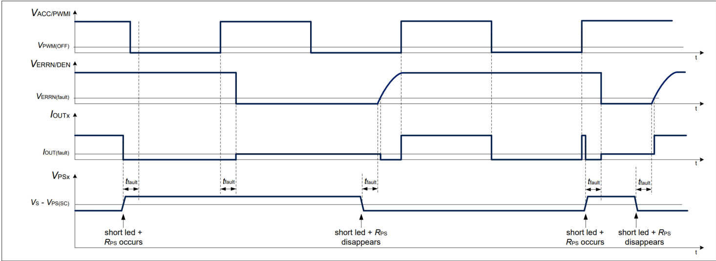
图 22 1-fail-all-ON 配置功率转移短路到电源条件图示例（D 引脚短路到接地）
