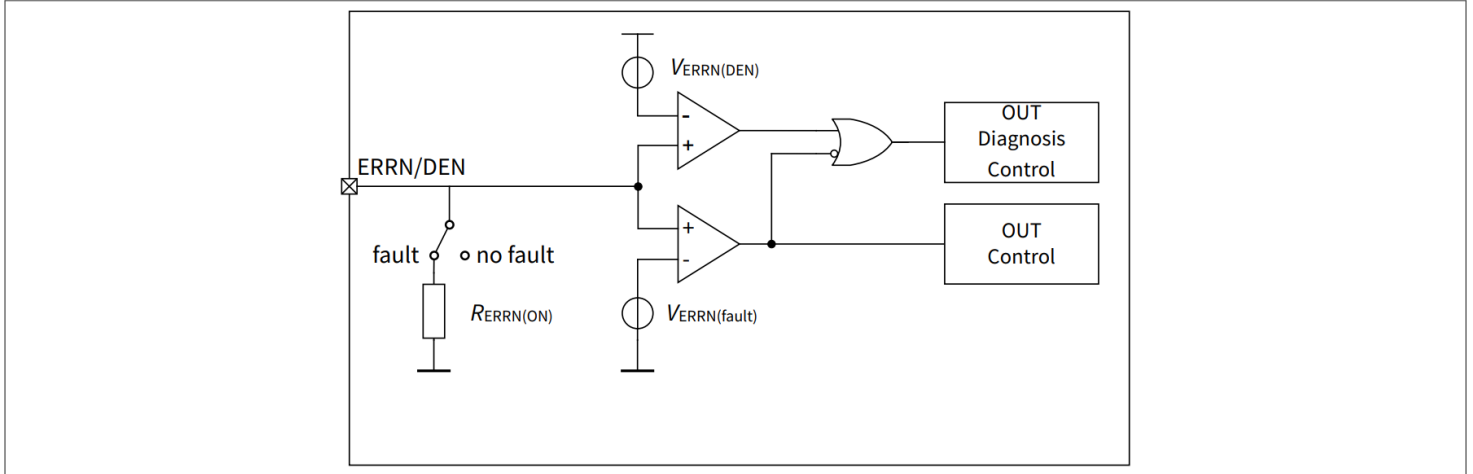
图 14 ERRN/EN 引脚（框图）
