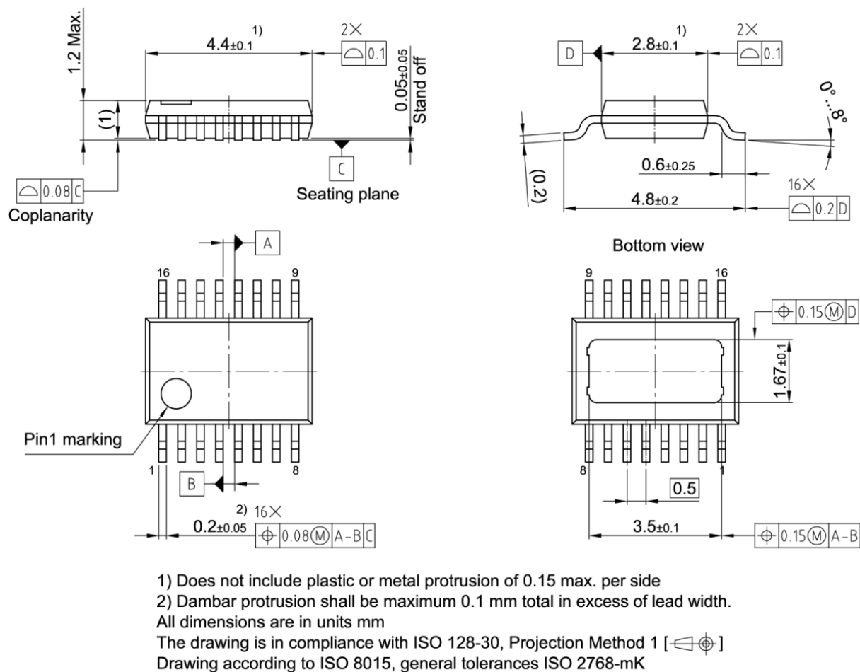
图 26 PG-TFDSO-16 封装外形 png
