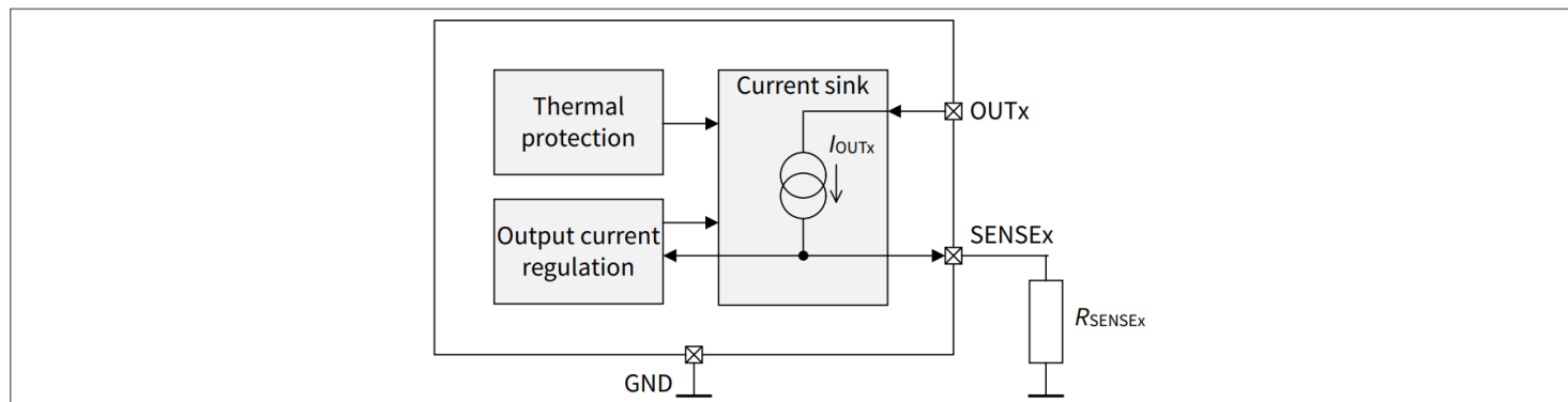
图 5 功率级框图
