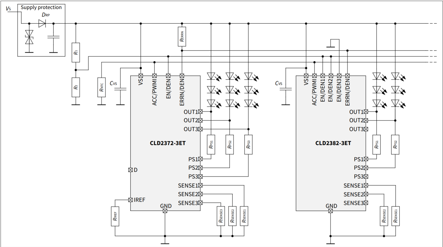
图 24 共享网络中 5 通道照明功能的应用图示例，具有“一错全关”故障管理和中央热降额功能
