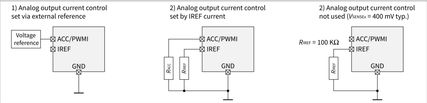
图 11 模拟输出电流控制配置
