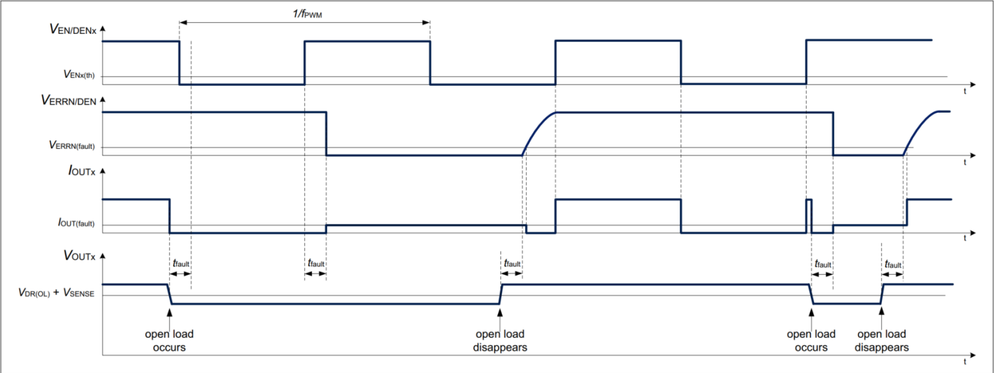
图 21 1-fail-all-ON 配置中的负载开路条件时序图示例（D 引脚对接地短路），并在 EN/DENx 引脚上应用数字调光
