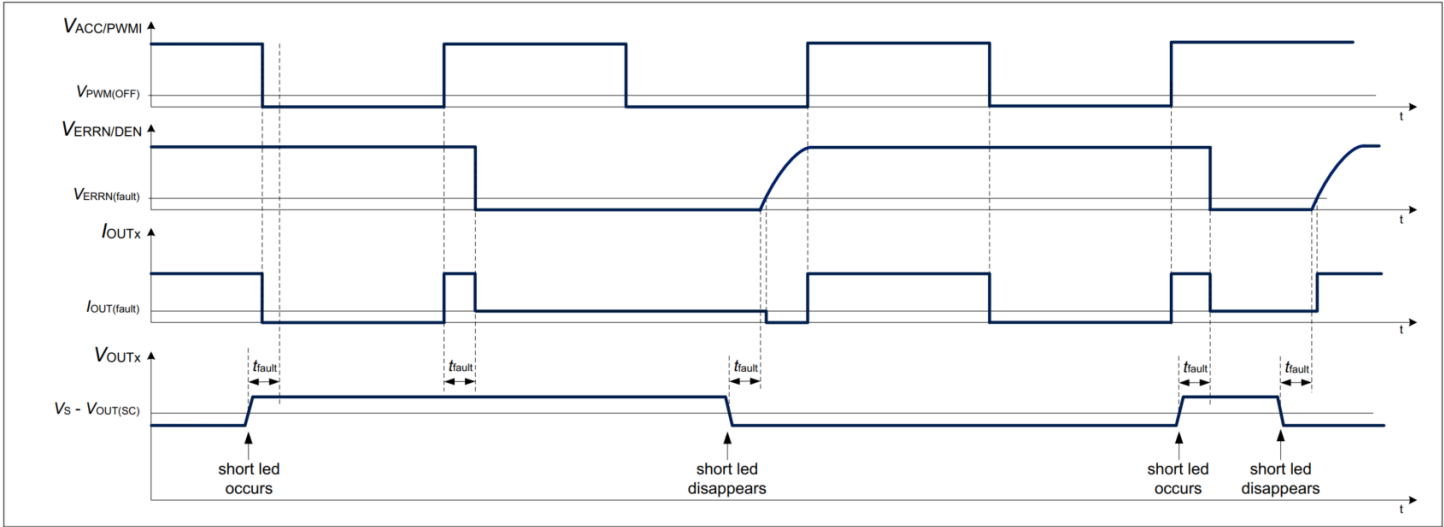
图 22 1-fail-all-ON 配置中的输出短路电源条件时序图示例（D 引脚对接地短路）
