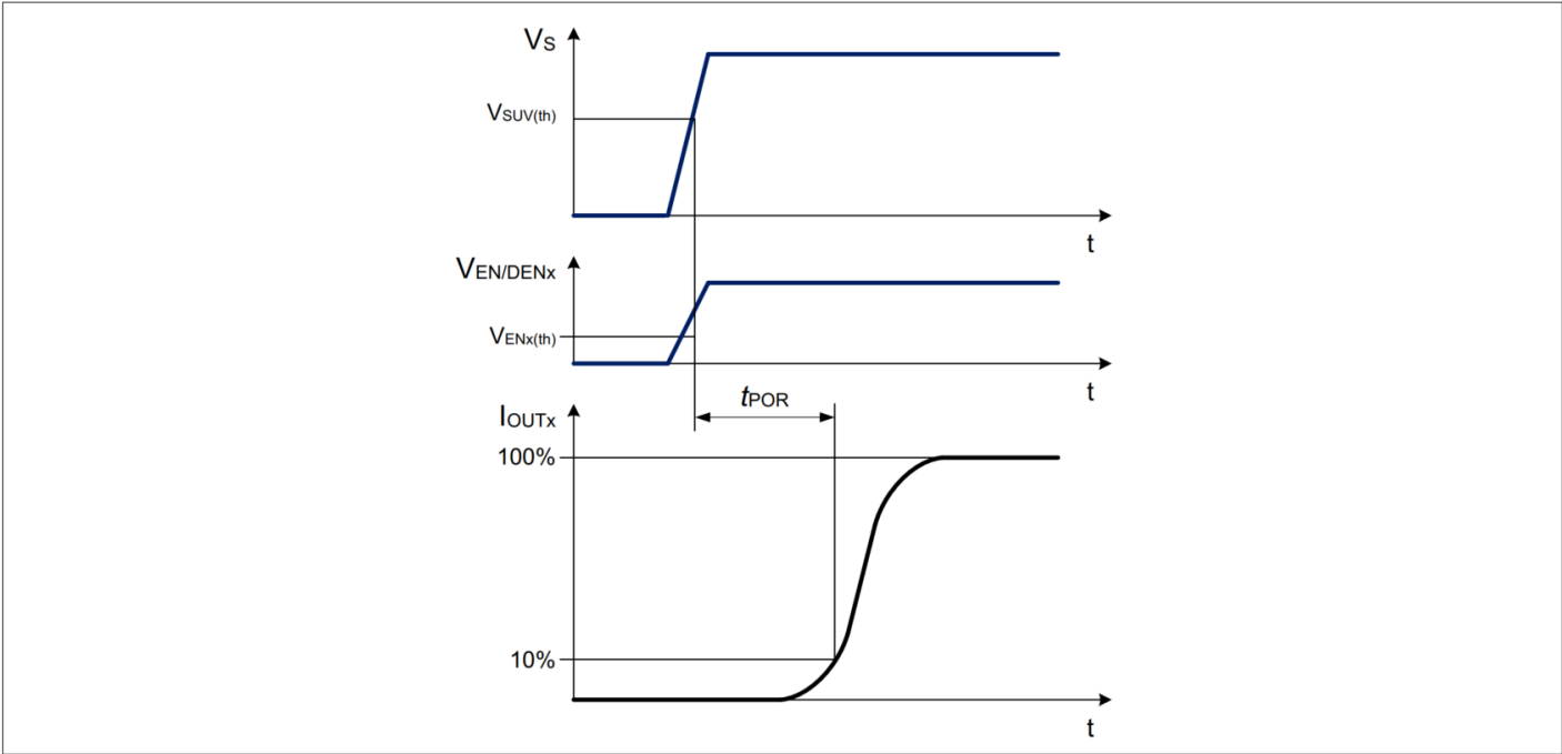
图 4 上电复位时序图
