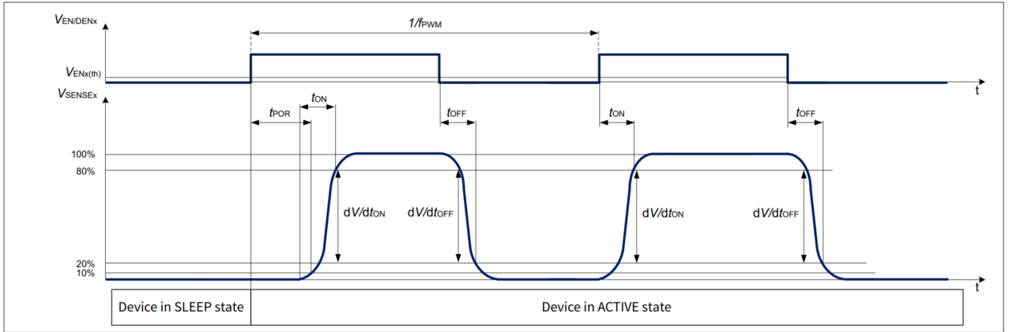
图 9 V_{ACC/PWMI} \geq 2.4V 时 EN/DENx 上的 PWM 控制时序图
