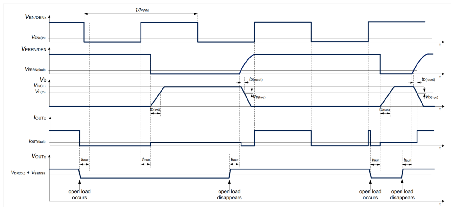
图 17 1-fail-all-OFF 配置中的负载开路条件时序图示例（D 引脚开路或连接到外部电容器），并在 EN/DENx 引脚上应用数字调光
