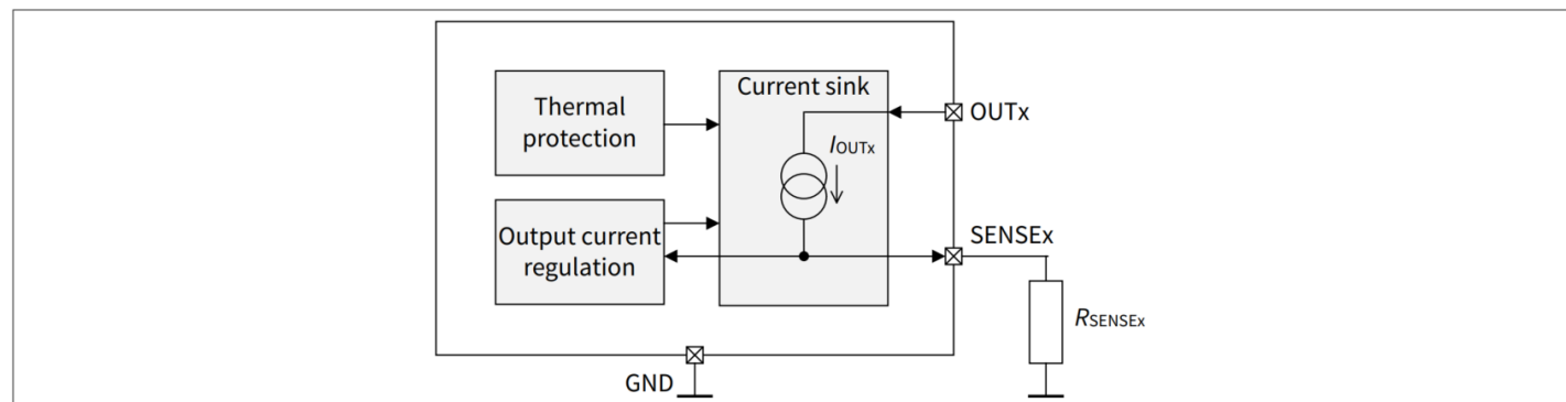
图 5 功率级框图
