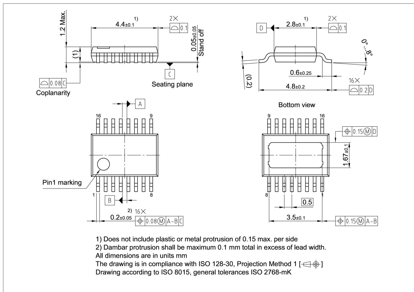
图 26 PG-TFDSO-16 封装外形 png
