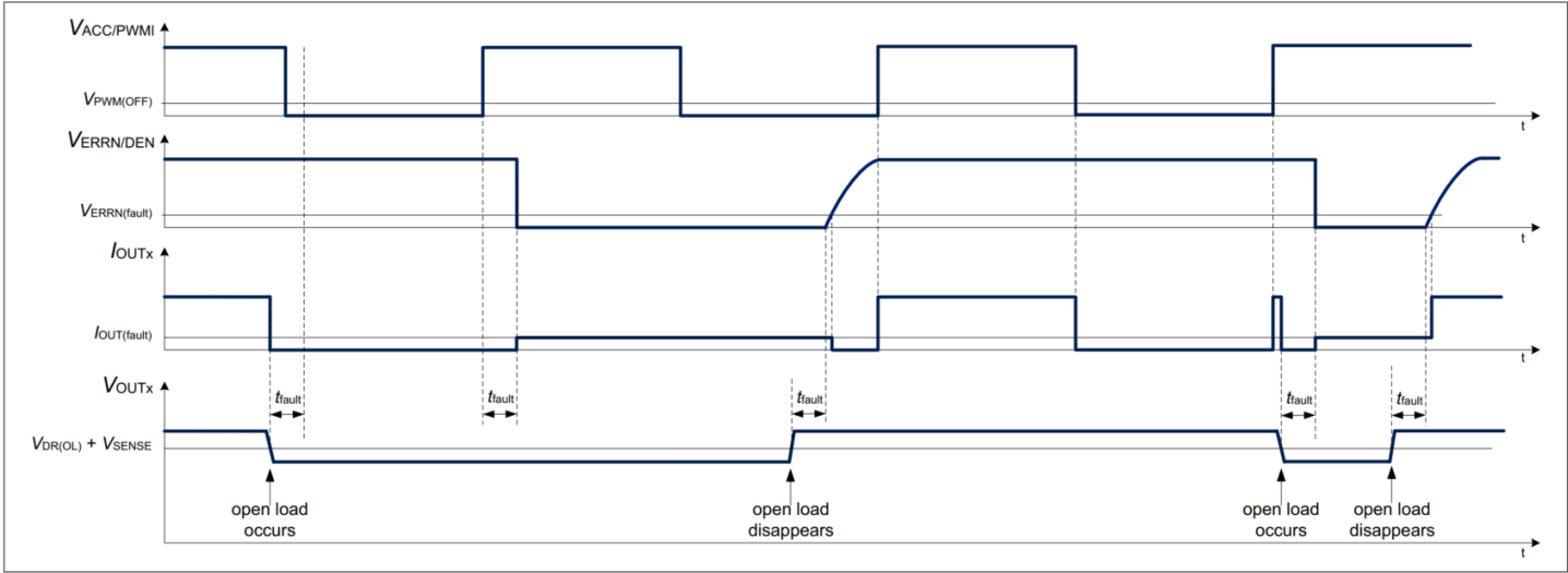
图 20 1-fail-all-ON 配置中的负载开路条件时序图示例（D 引脚短接到接地）
