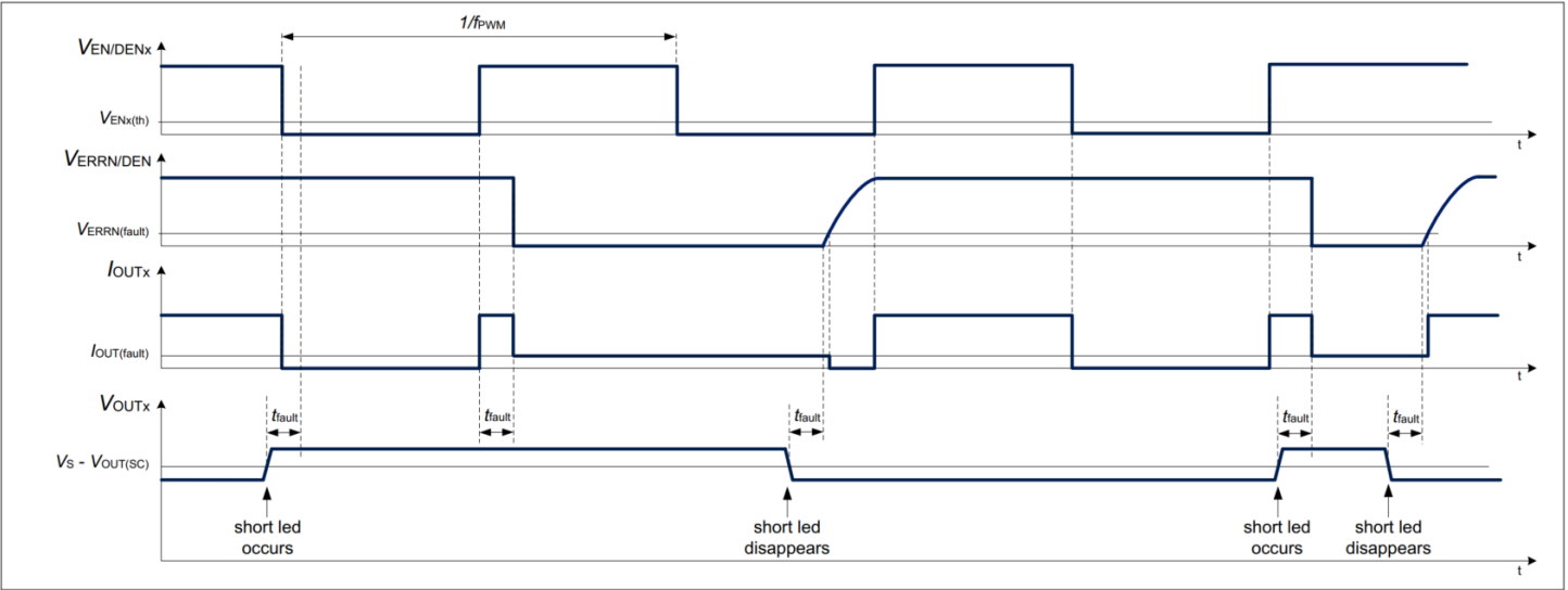
图 23 1-fail-all-ON 配置中的输出短路电源条件时序图示例（D 引脚对接地短路）,并在 EN/DENx 引脚上应用数字调光
