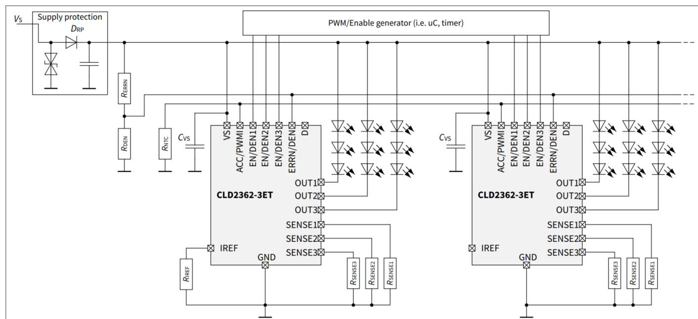
图 25 共享网络中动态照明功能的应用图示例，具有“一错全关”故障管理和中央热降额功能
