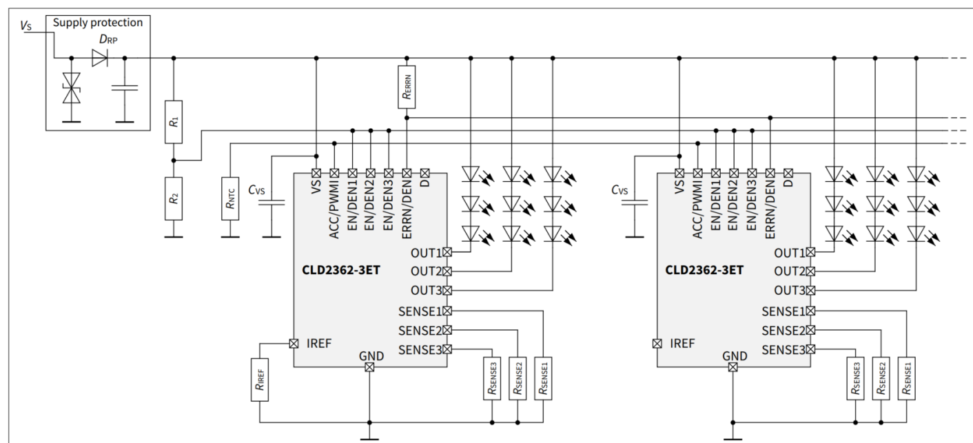
图 24 具有“一错全关”故障管理和中央热降额的共享网络中的应用图示例
