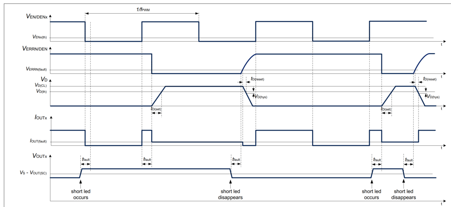
图 19 1-fail-all-OFF 配置中的输出短路电源条件时序图示例（D 引脚开路或连接到外部电容器），并在 EN/DENx 引脚上应用数字调光。
