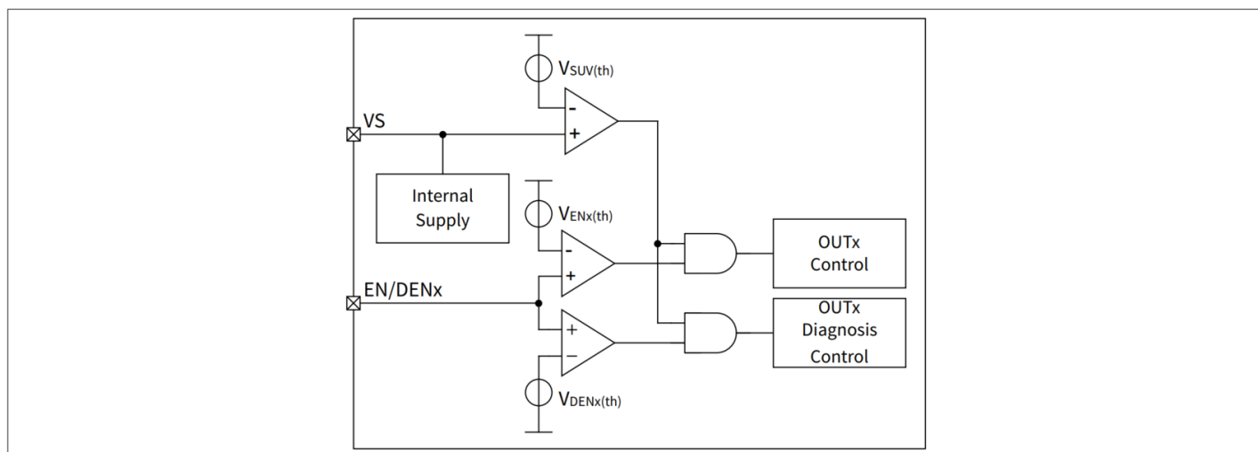
图 12 EN/DEN 框图
