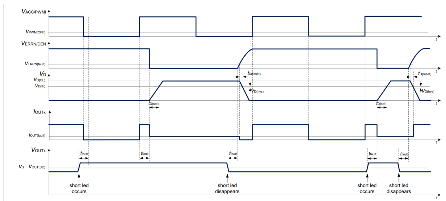
图 18 1-fail-all-OFF 配置中的输出短路电源条件时序图示例（D 引脚开路或连接到外部电容器）
