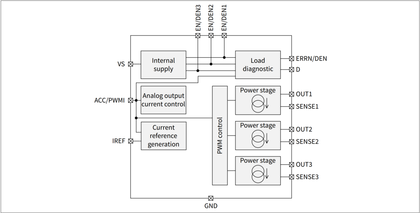
图2 CLD2362-3ET 框图
