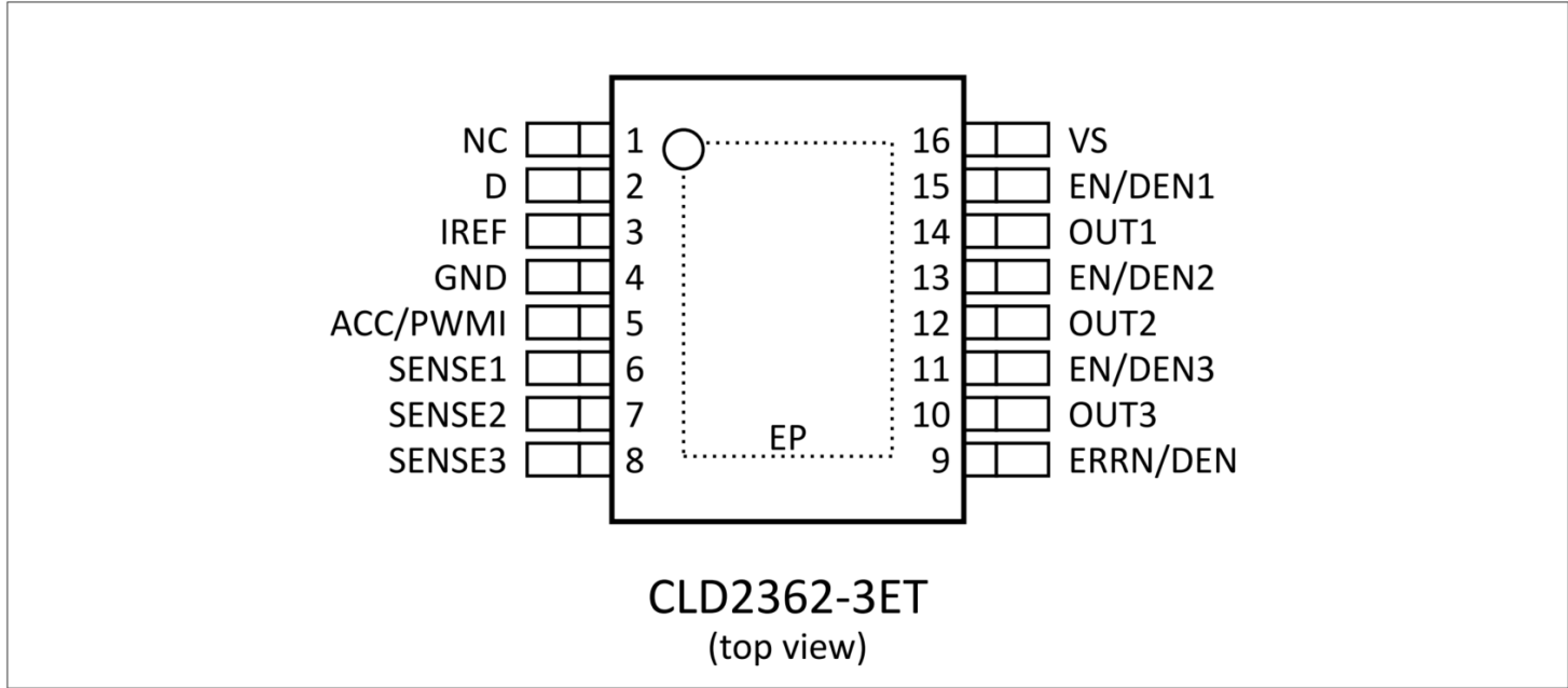
图3 PG-TFDSO-16 引脚配置
