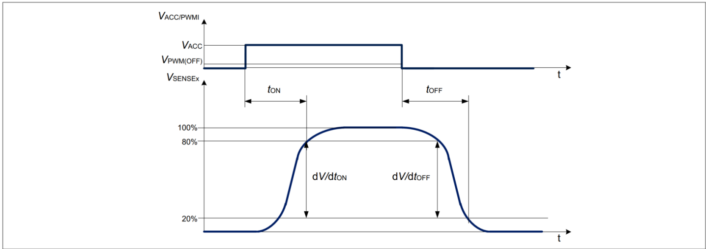
图 8 V_{ACC/PWMI} \geq 2.4 V 时的 PWMI 控制时序图
