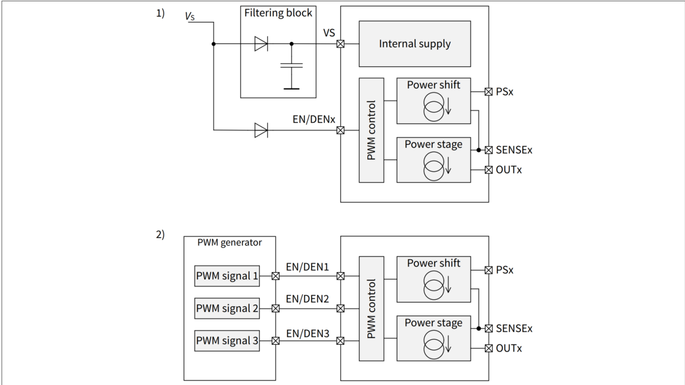
图 7 通过 EN/DENx 输入引脚进行 PWM 控制
