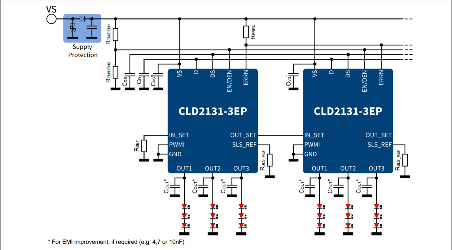
图 26 应用图示例
