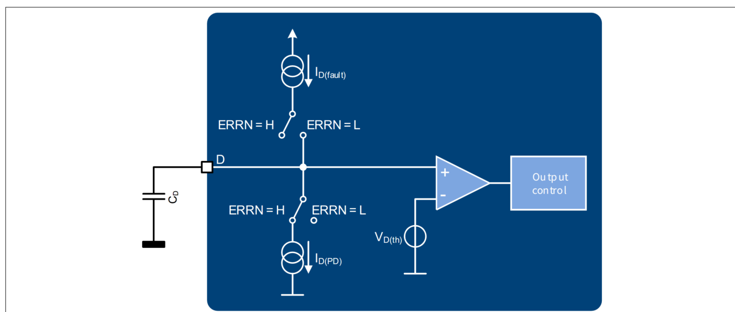
图 17 D 引脚（框图）。
