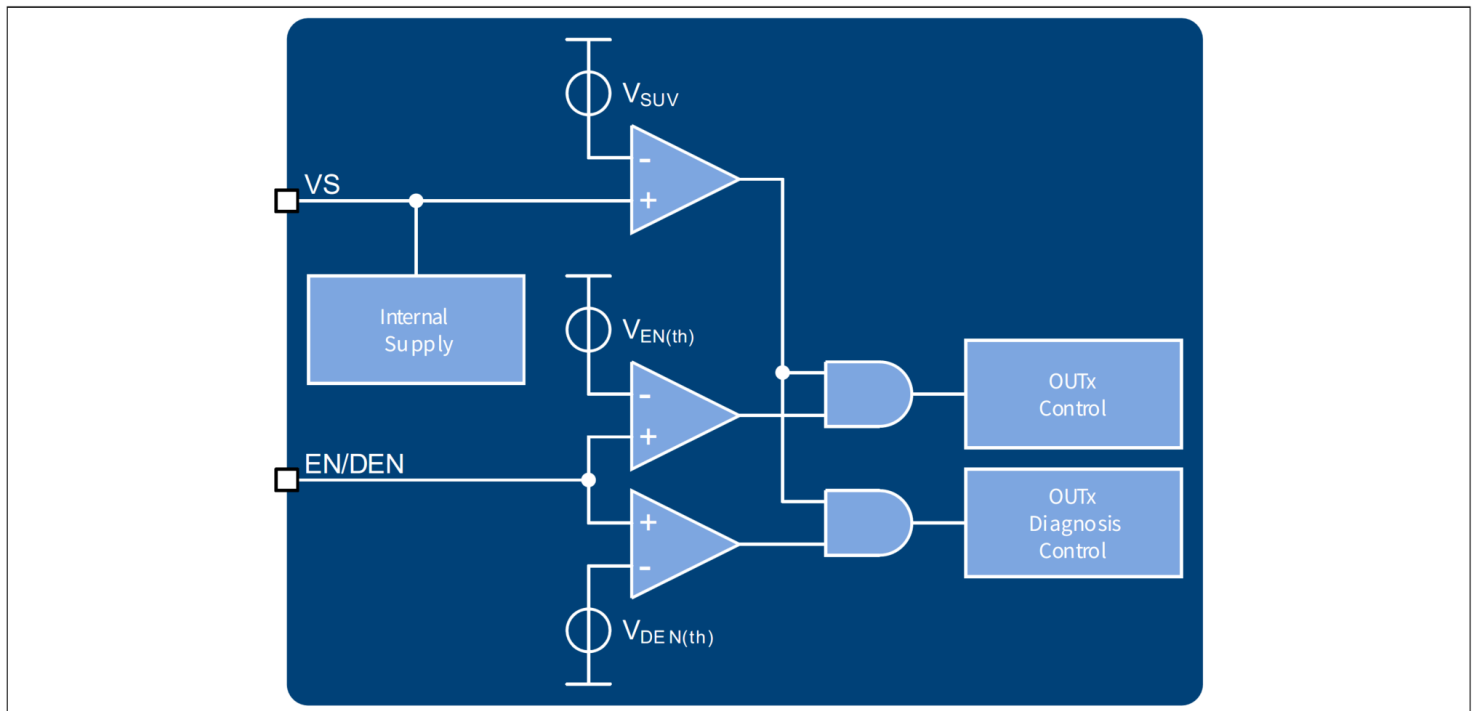
图 3 内部供电
