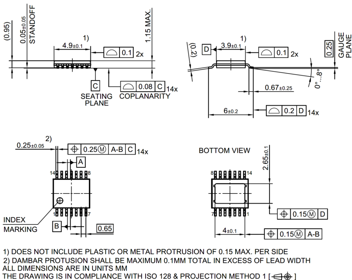
图 27 PG-TSDSO-14
