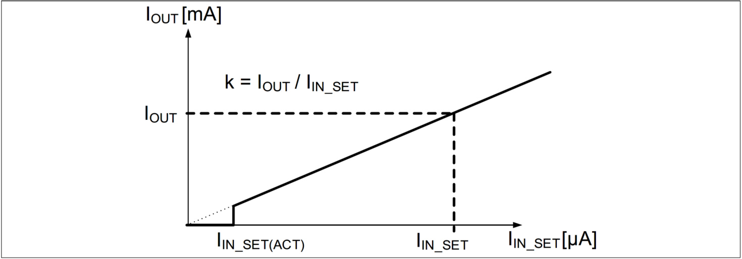
图 7 I_{OUT} 与 I_{IN\_SET}
