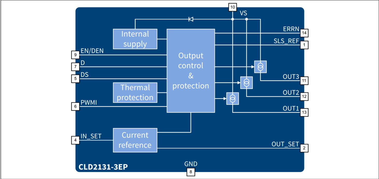
图 1 框图
