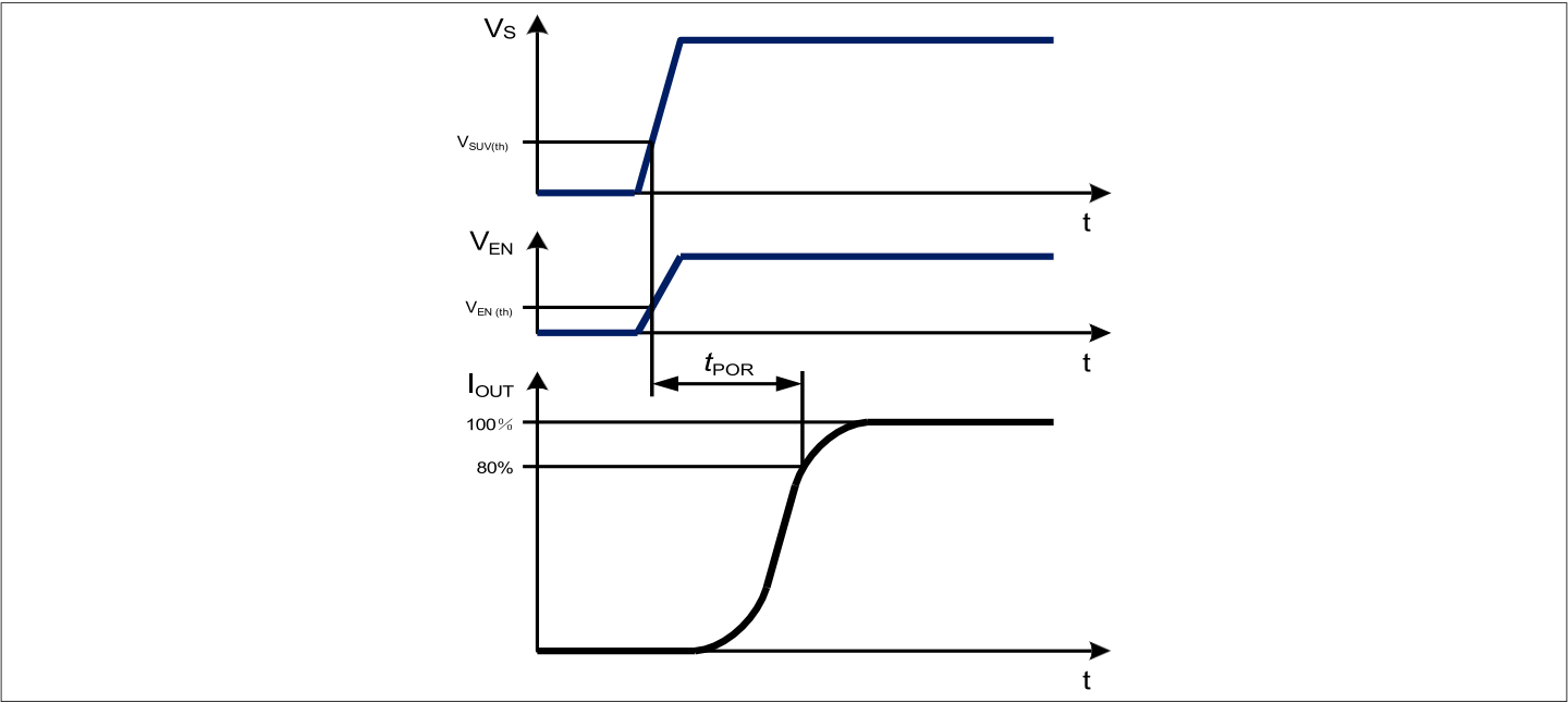
图 4 上电复位时序图
