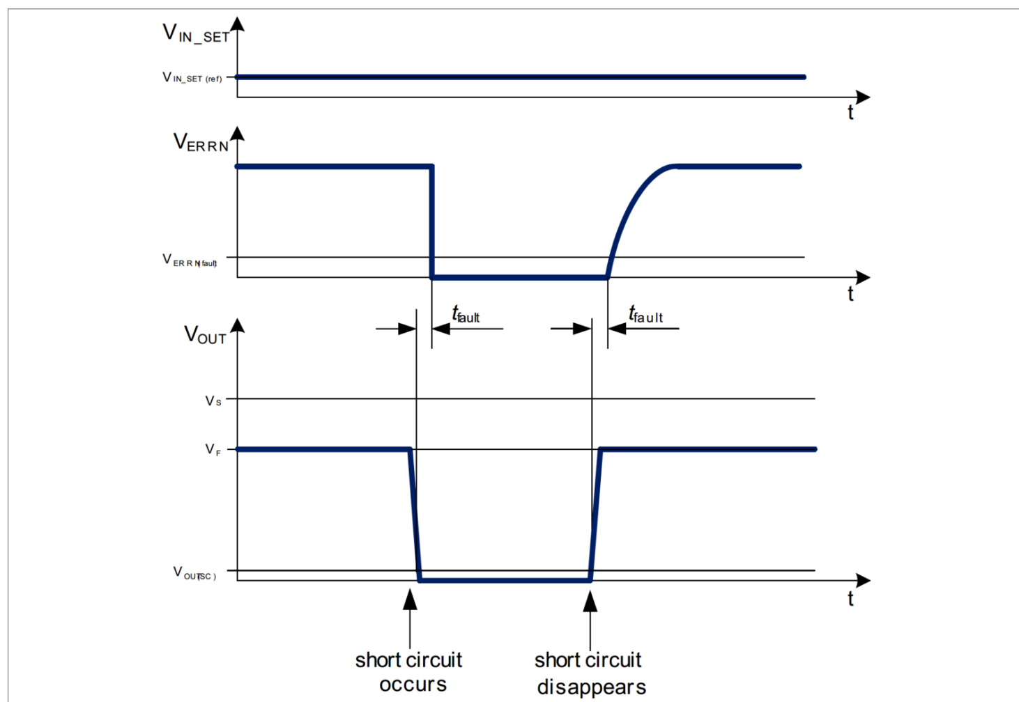
图 21 短路条件时序图示例 (D 引脚连接到 GND, V_F 表示输出负载的正向电压)
