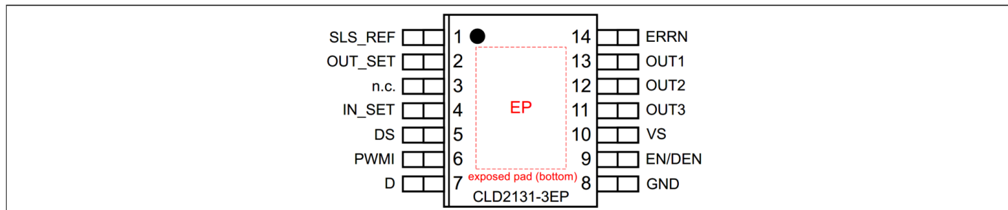
图 2 引脚配置
