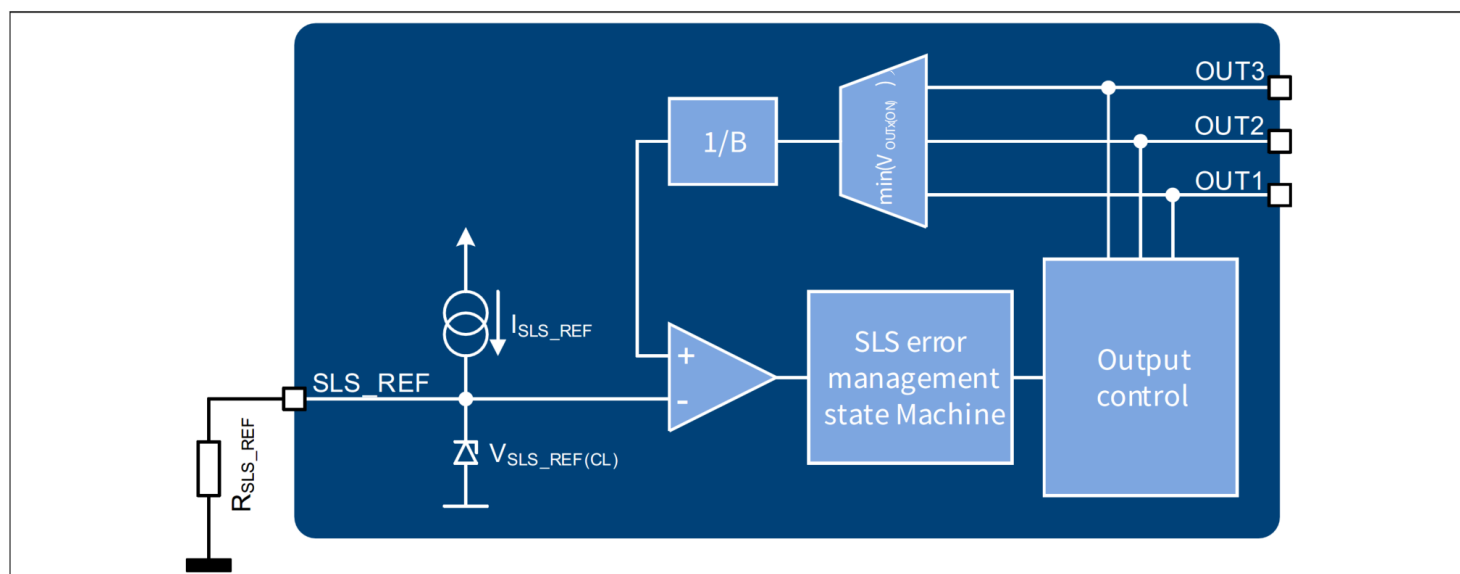
图 22 带电阻终端的 SLS_REF 引脚（框图）
