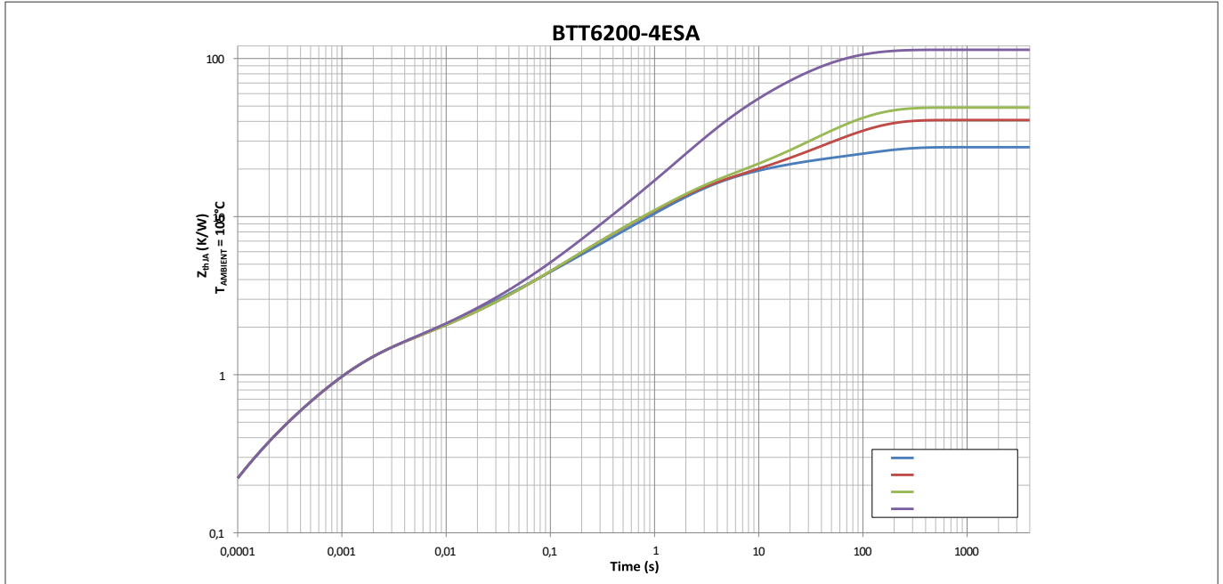
图 7 典型热阻抗2s2p PCB 设置如图 5 所示
