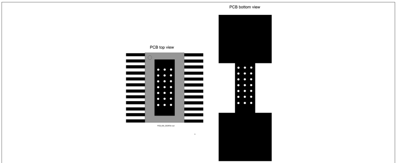
图 6 带有 600 mm 2 冷却面积的 PC 板热仿真顶视图和底视图
