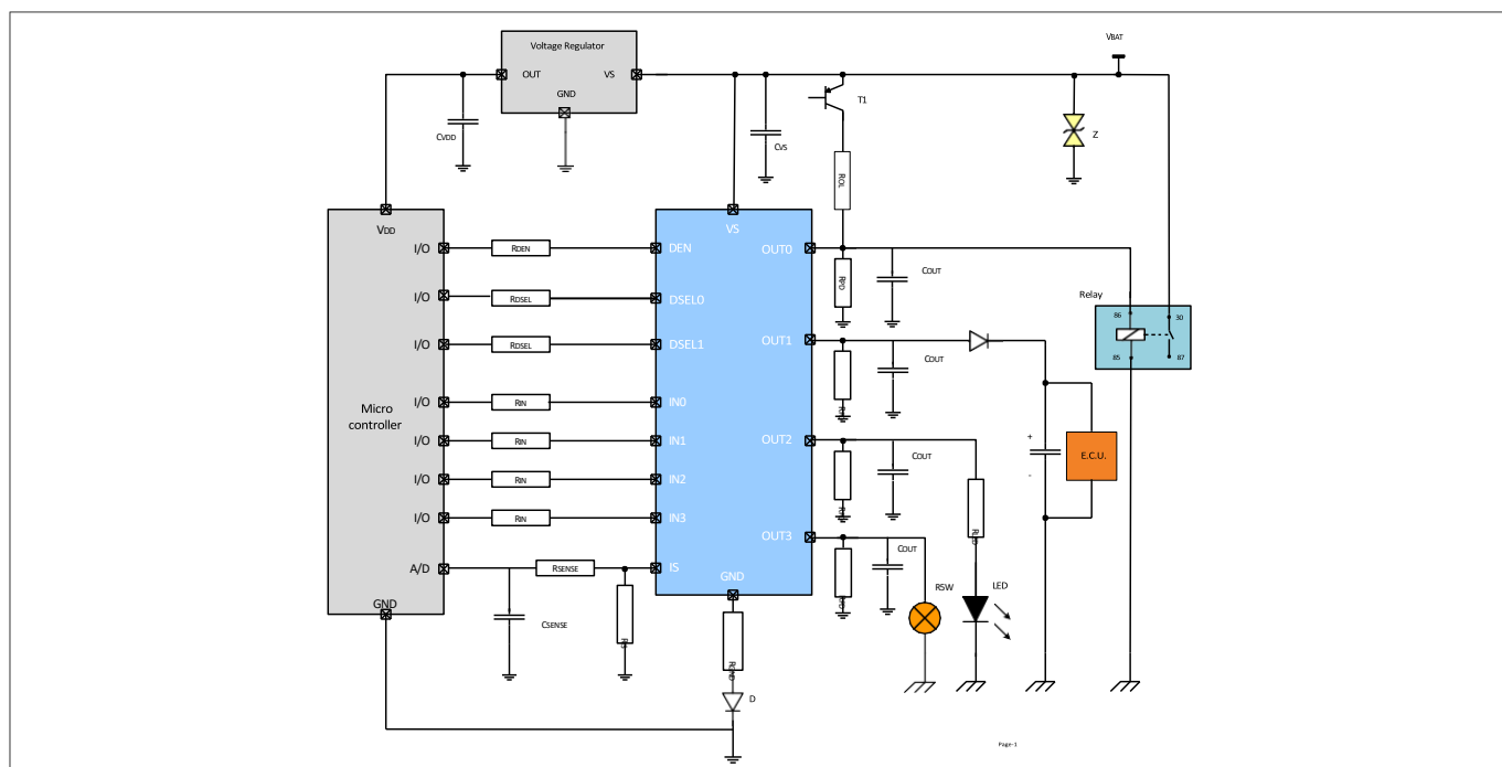
图 1 BTT6200-4ESA 应用图
