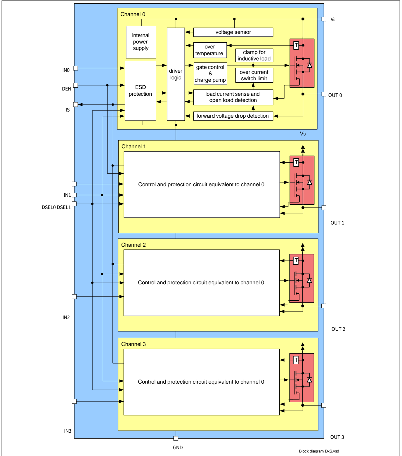
图 2 BTT6200-4ESA 框图
