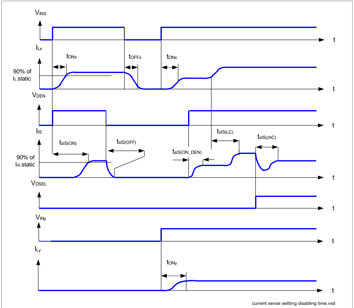
图 23 电流检测建立/禁用时序
