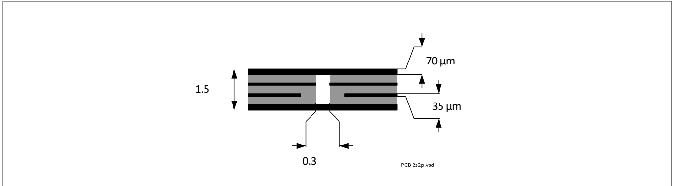
图 5 2s2p PCB 截面
