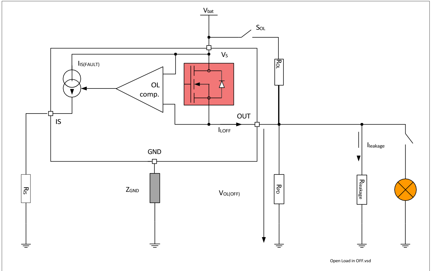
图 25 负载开路检测 OFF 电气等效电路
