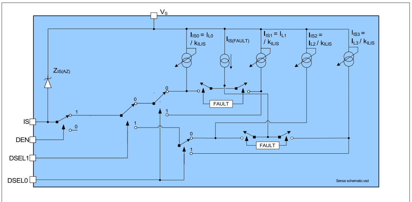
图 20 诊断框图
