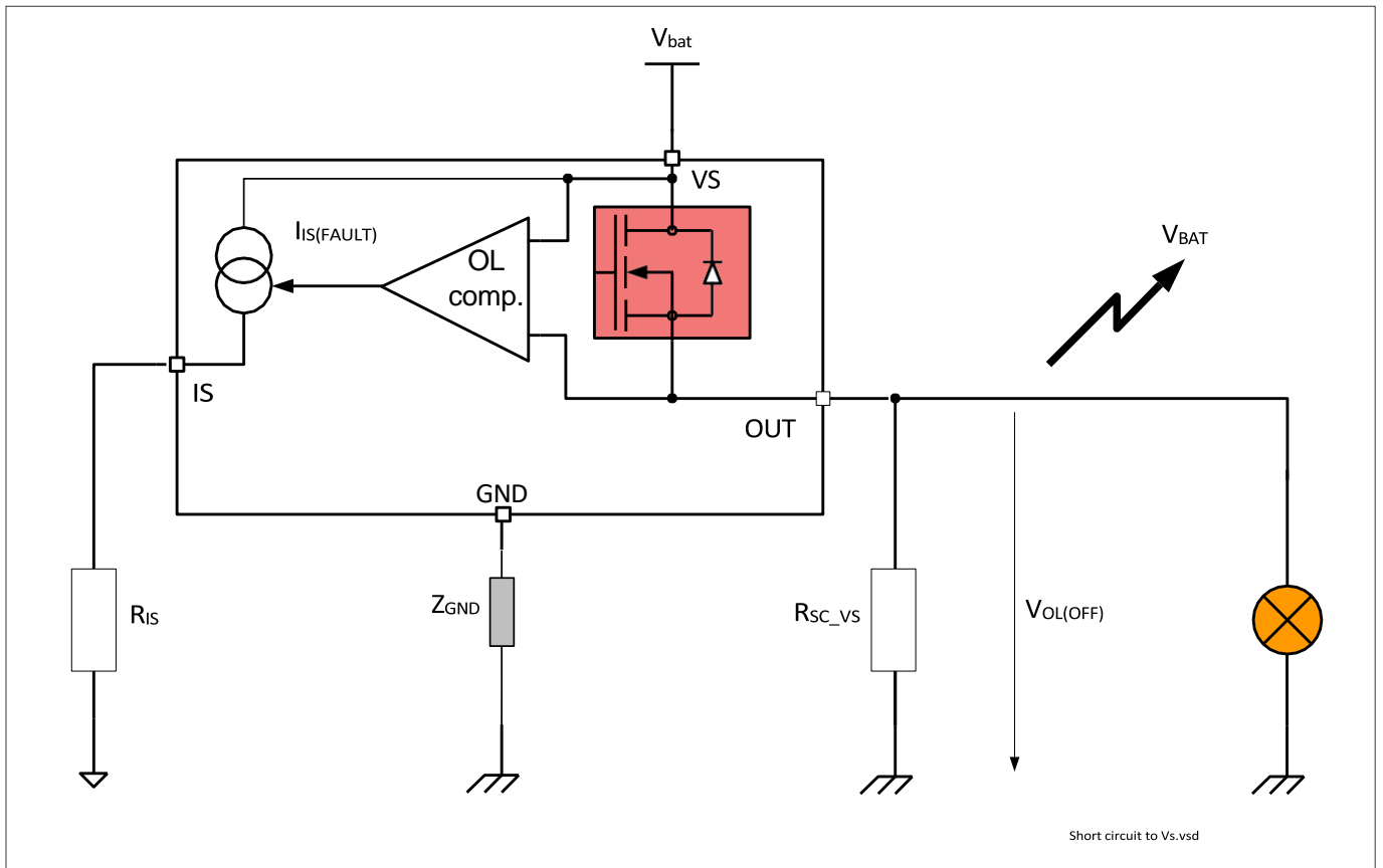
图 27 对电池短路检测 OFF 电气等效电路
