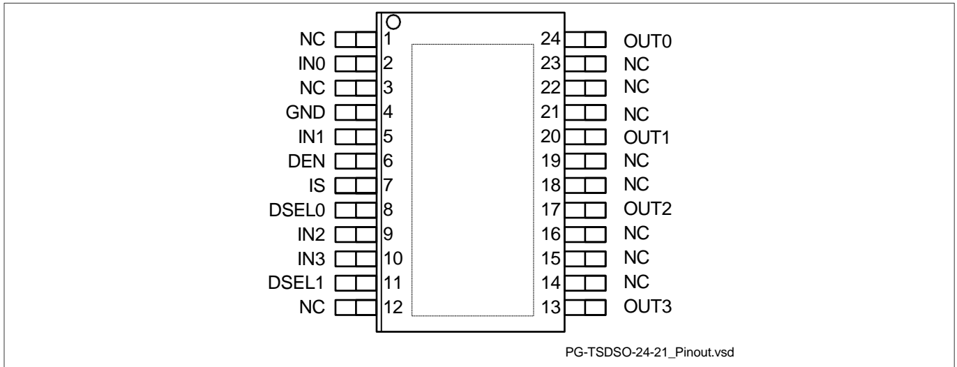
图 3 引脚配置
