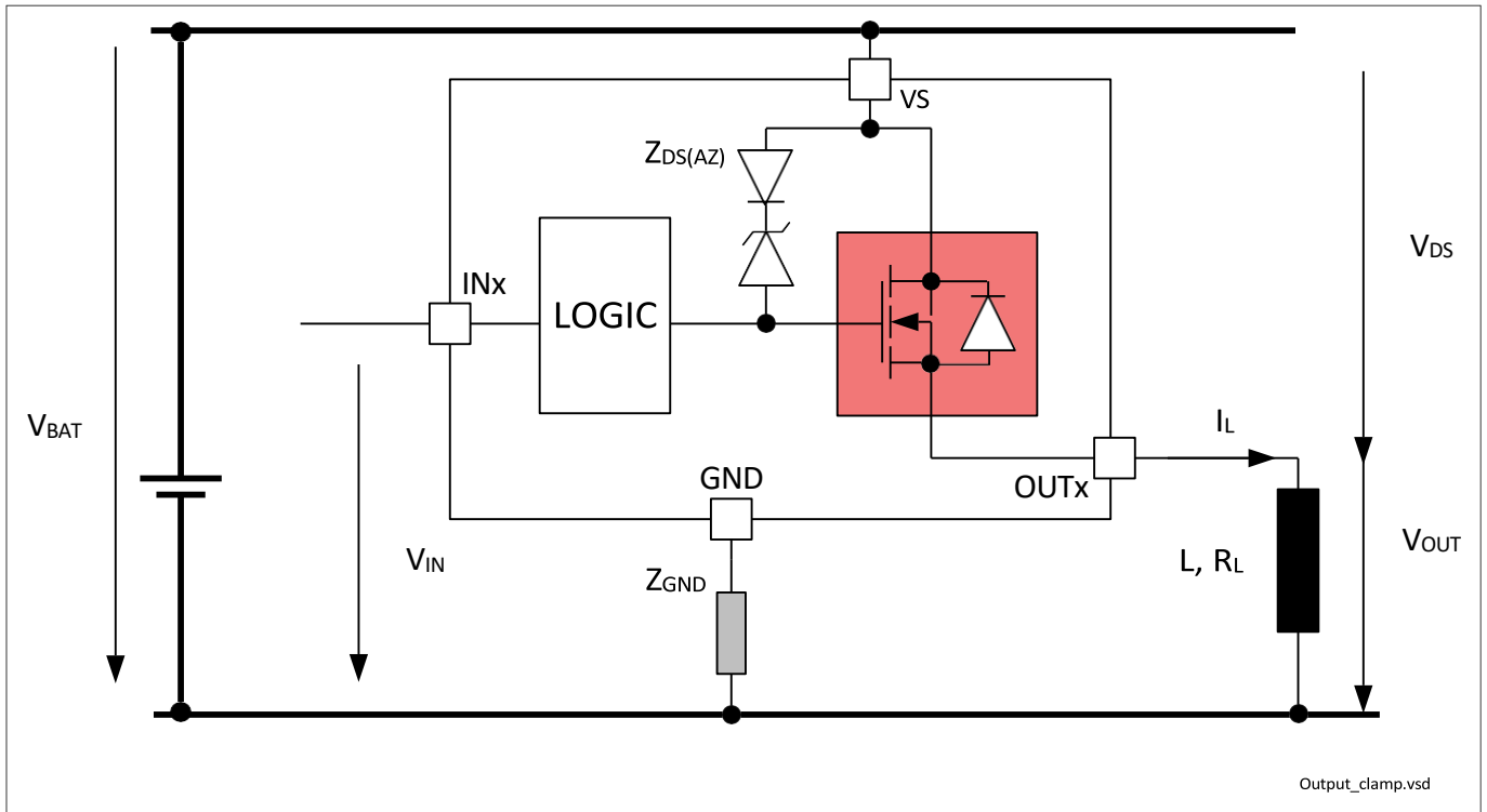
图 11 输出钳位
