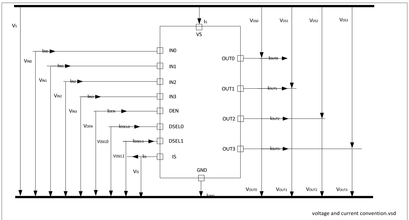
图 4 电压和电流定义
