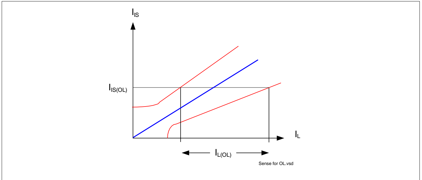
图 24 低电流的电流检测比
