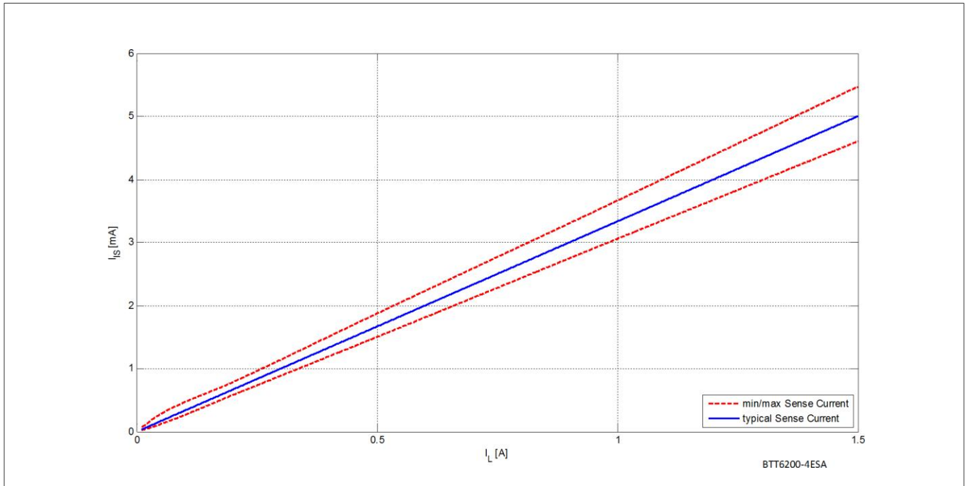
图 21 标称负载的电流检测
