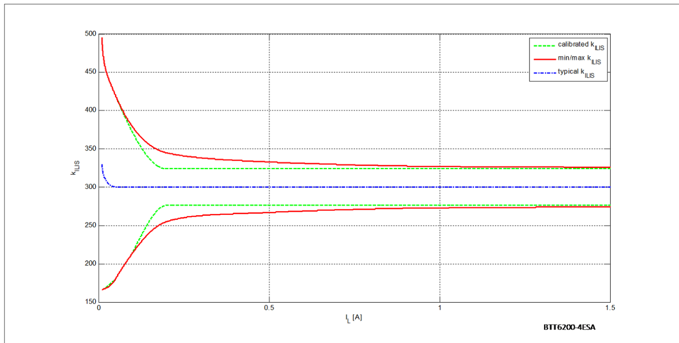
图 22 0.2 A 下 1 个调整点提高电流检测精度
