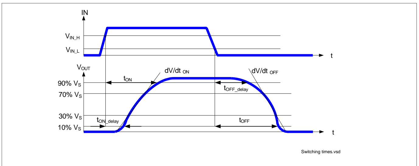
图 10 开关电阻性负载时序
