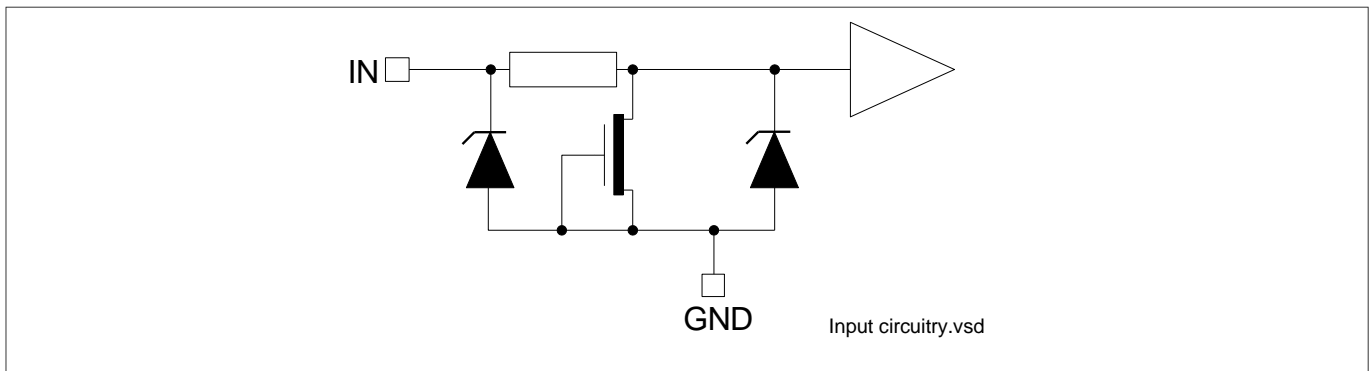
图 28 输入引脚电路
