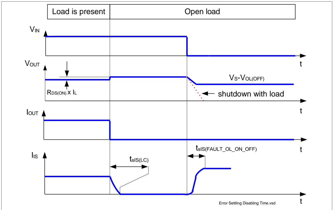
图 26 负载开路过程中的检测信号
