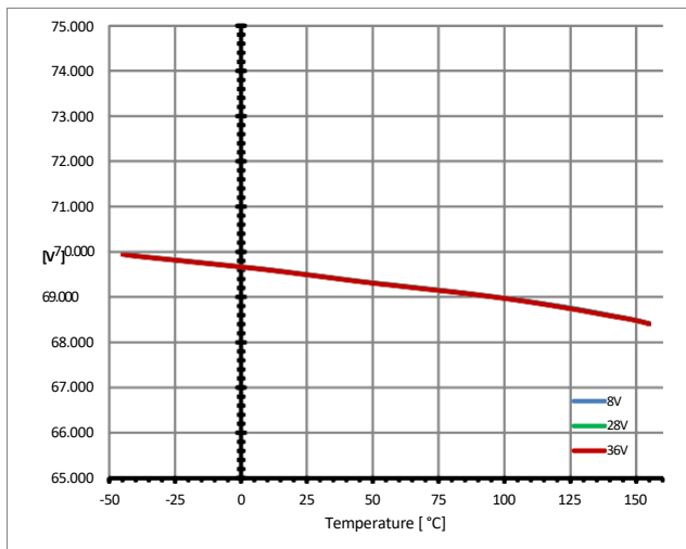
最大电压处的检测信号 V_{IS(AZ)} = f(T_J; V_S)
