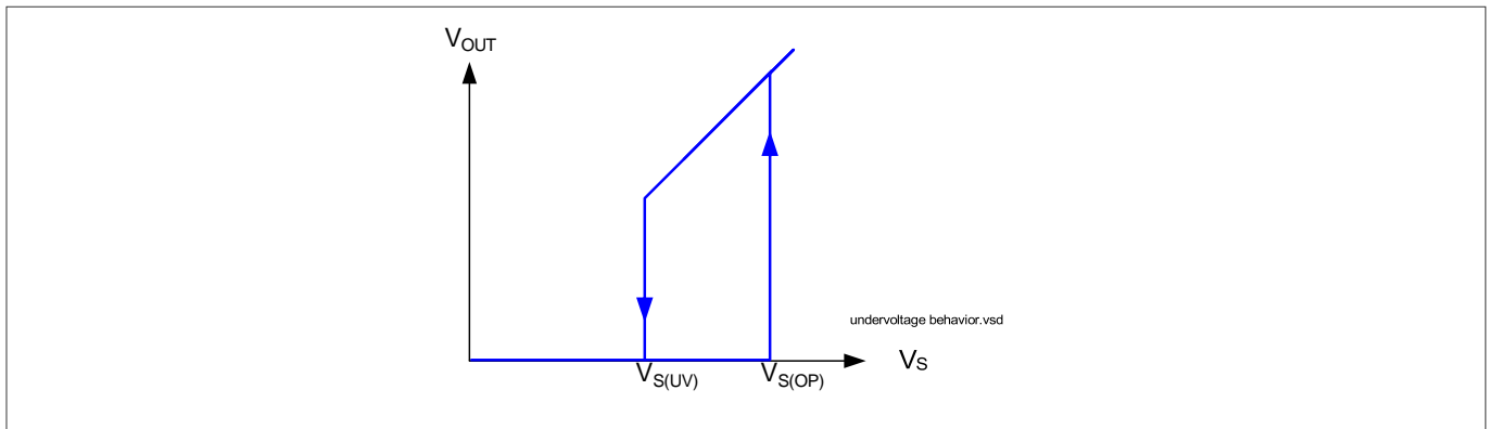
图 16 欠压行为
