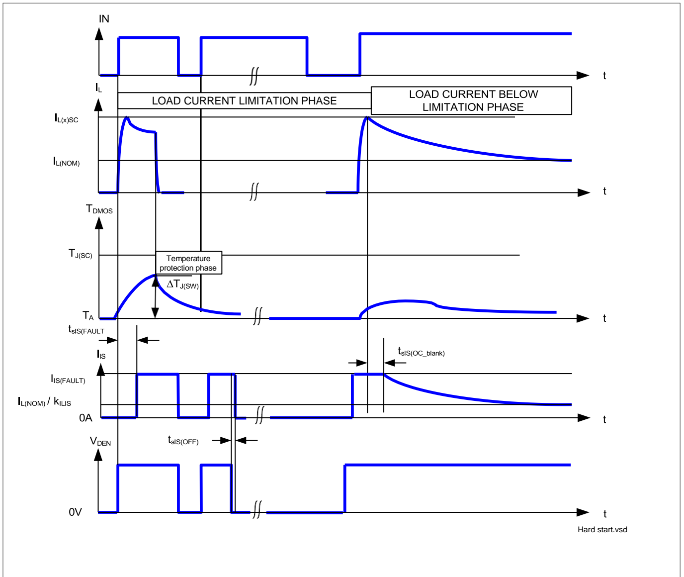
图 19 过载保护
