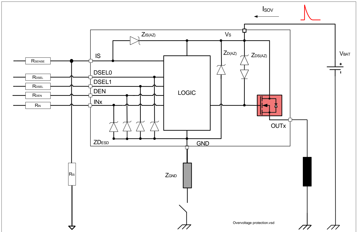
图 17 采用外部元件的过压保护
