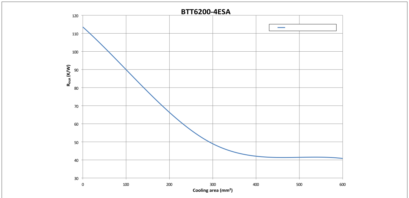
图 8 典型热阻PCB 设置 1s0p
