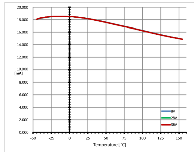
默认状态下的检测信号最高电流 I_{IS(FAULT)} = f(T_J; V_S)
