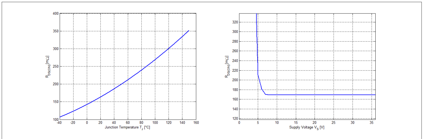
图 9 典型导通电阻
