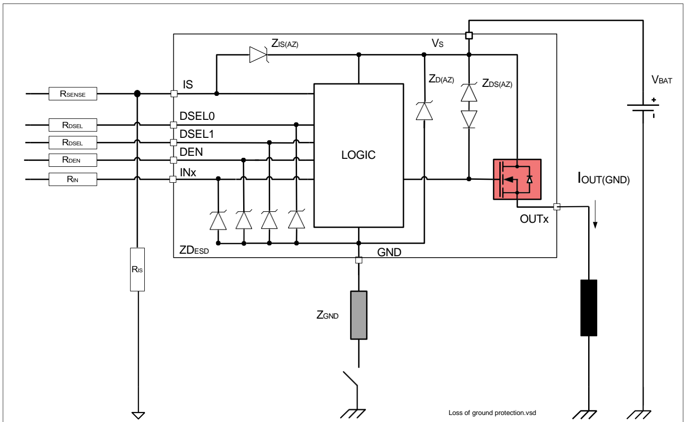
图 15 与外部元件的接地丢失保护
