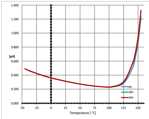
空载电流检测 I_{IS} = f(T_J; V_S) I_L = 0
