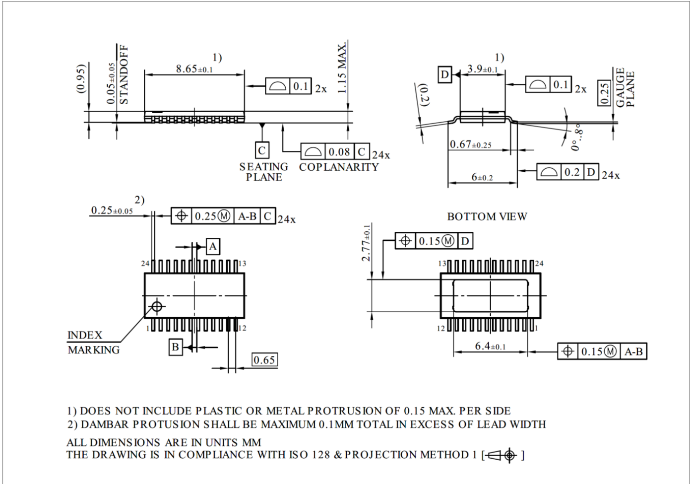
图 30 PG-TSDSO-24 (塑料双小外形封装) (符合 RoHS 标准)
