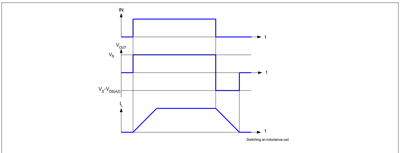
图 12 开关感性负载时序
