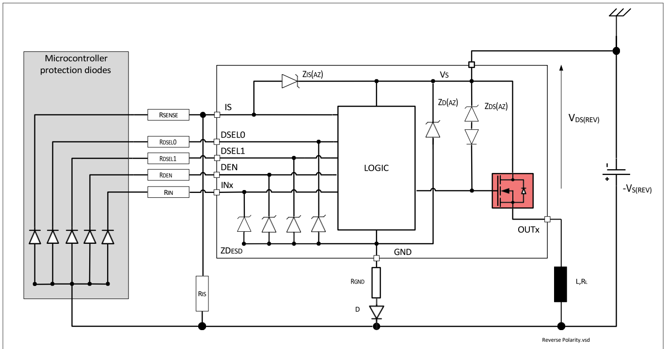
图 18 使用外部元件实现反极性保护
