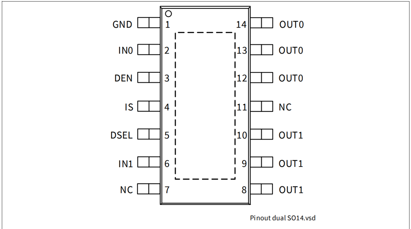
图 2 引脚配置
