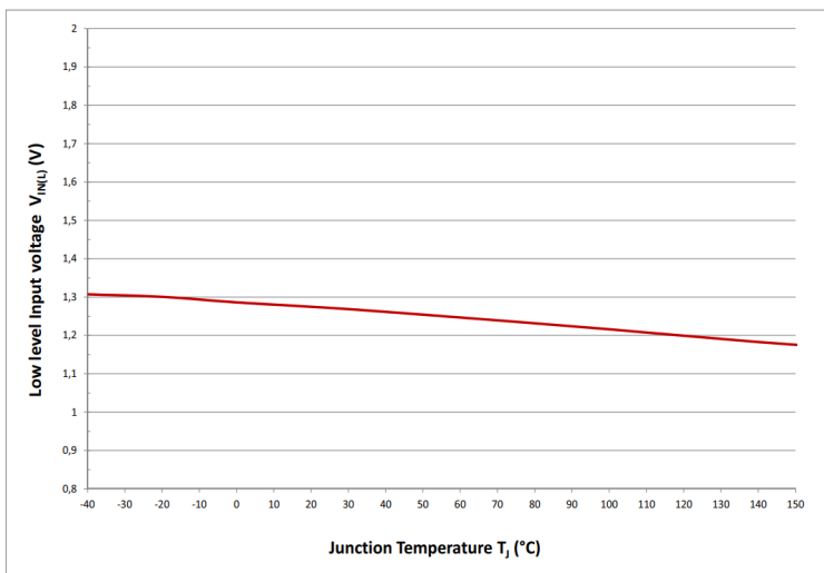
图 49 输入电压阈值 V_{IN(L)} = f(T_J; V_S)
