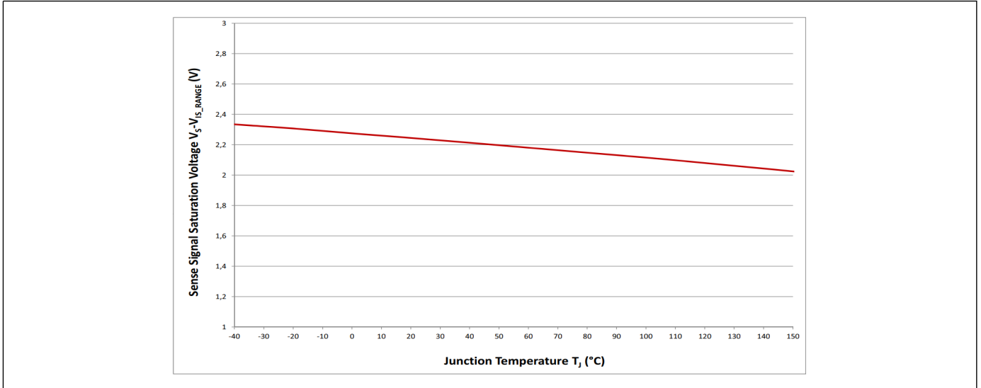
图 47 Sense 信号饱和电压 V_S - V_{IS(RANGE)} = f(T_J; V_S)
