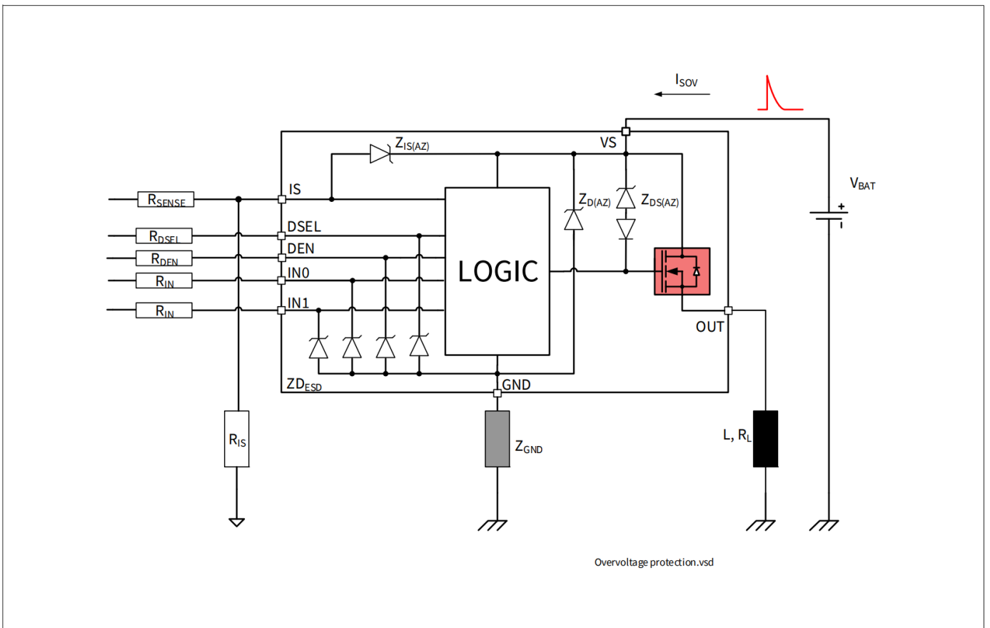
图 16 使用外部元器件的过压保护
