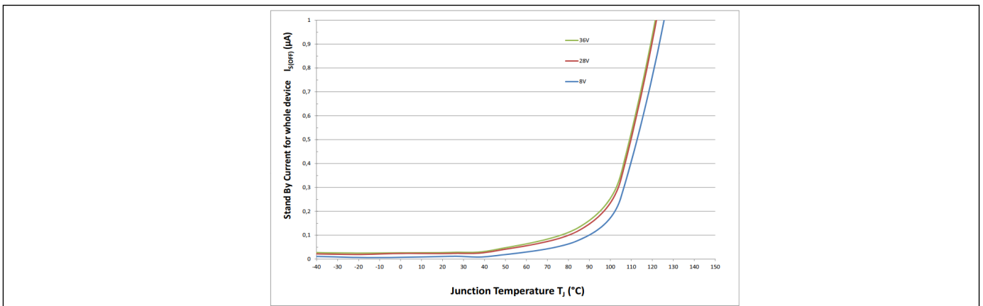
图 33 整个器件带负载的待机电流。 I_{S(OFF)} = f(T_J; V_S)
