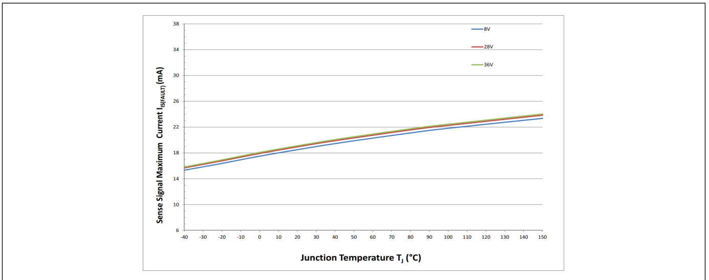
图 48 默认状态下的Sense信号最大电流 I_{IS(FAULT)} = f(T_J; V_S)
