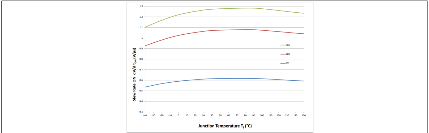
图 36 开启时间斜率 dV/dt_{ON} = f(T_j; V_s), R_L = 12\Omega
