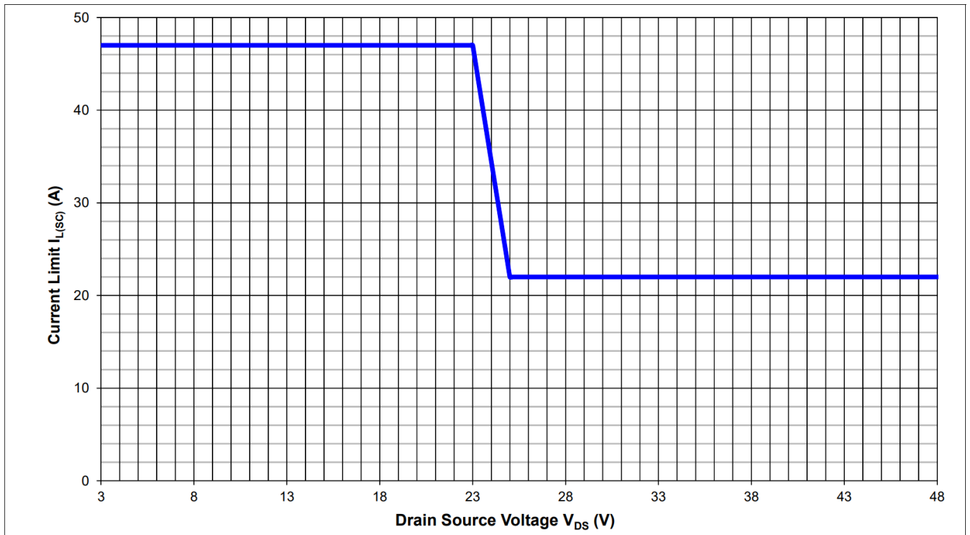
图 18 电流限制（典型行为）
