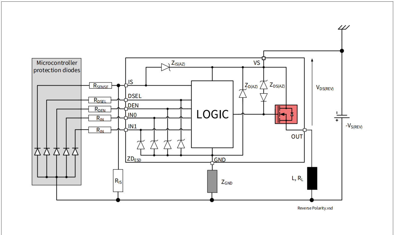
图 17 使用外部元器件实现反极性保护
