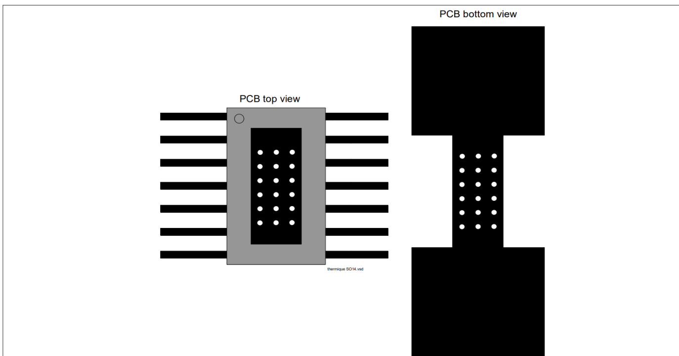
图 5 带有 600 mm 2 冷却面积的PC板热仿真顶视图和底视图
