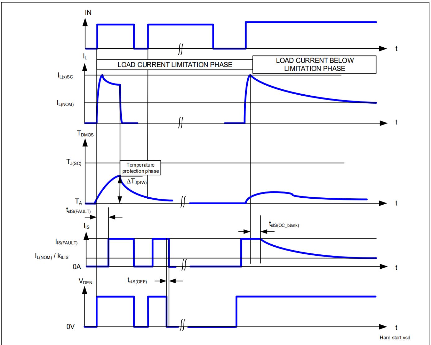
图 19 过载保护
