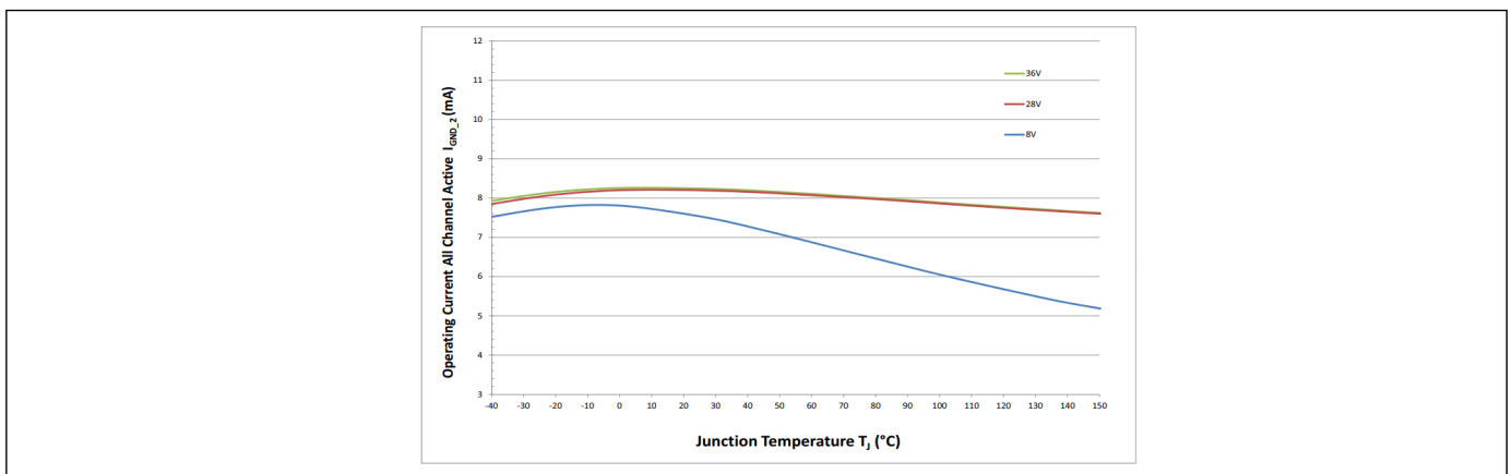
图 32 整个器件带负载的电流损耗。双通道有效 I_{GND\_2} = f(T_J; V_S)
