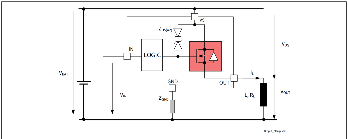
图 10 输出钳位 (OUT0 和 OUT1)
