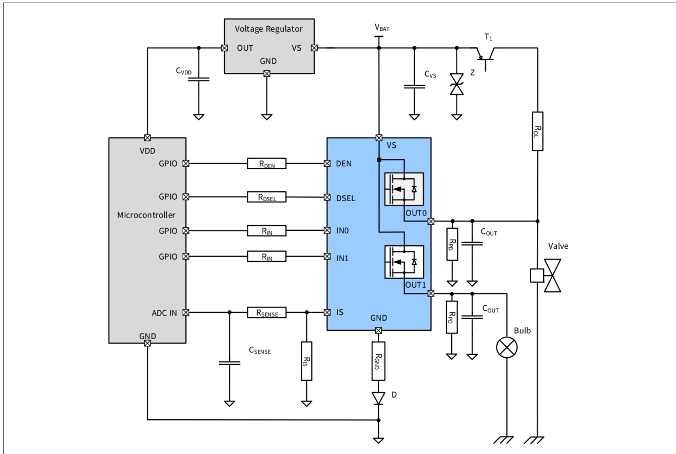
BTT6050-2ERA 应用图
