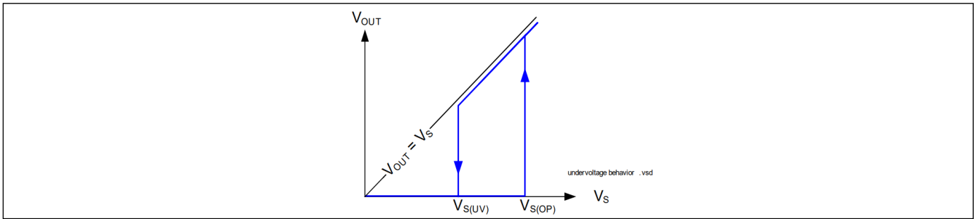
图 15 欠压行为
