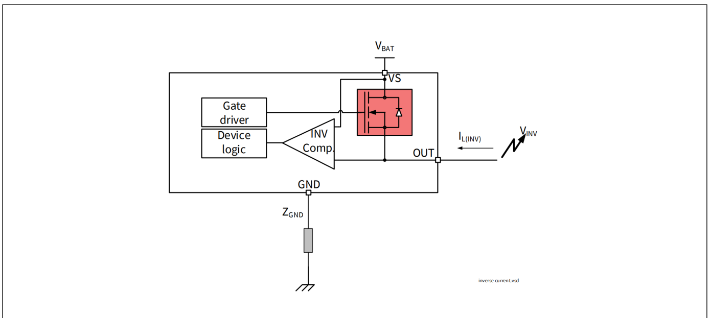
图 13 反向电流电路
