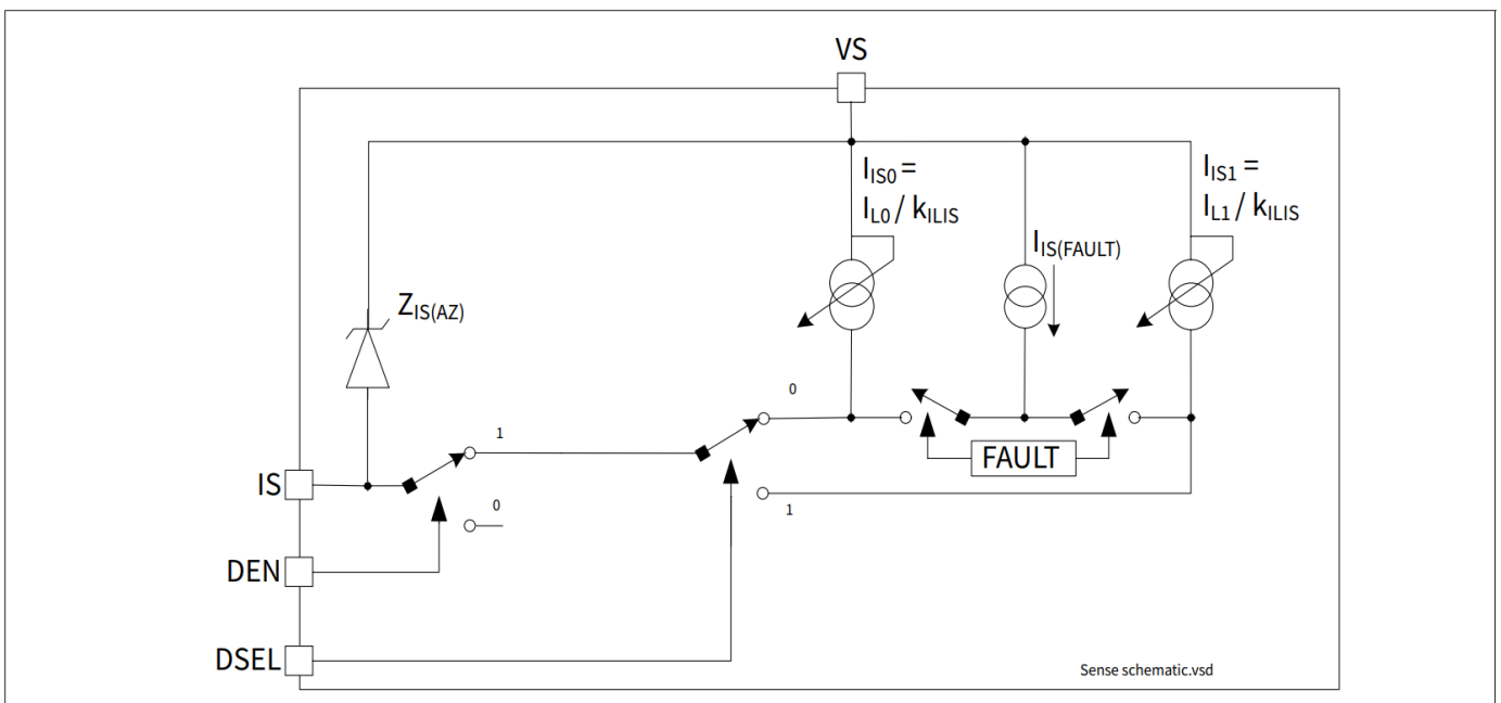
图 20 诊断框图
