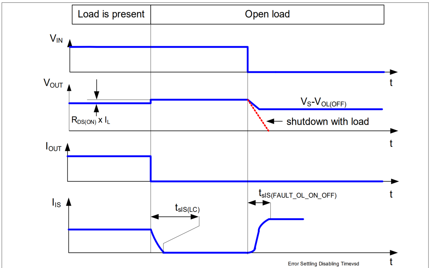
图 26 负载开路中的 SENSE 信号
