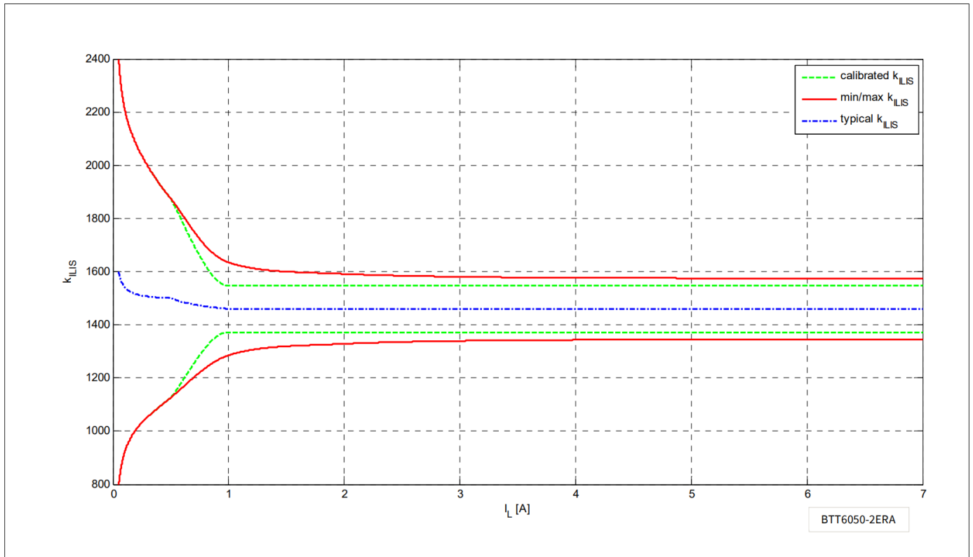
图 22 通过一个校准点提高 SENSE 精度
