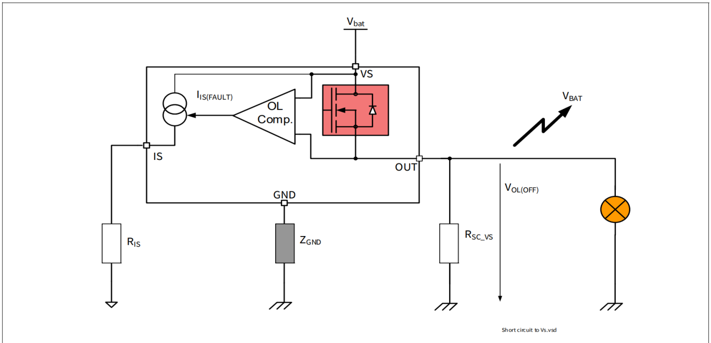
图27 对电池短路检测OFF电气等效电路
