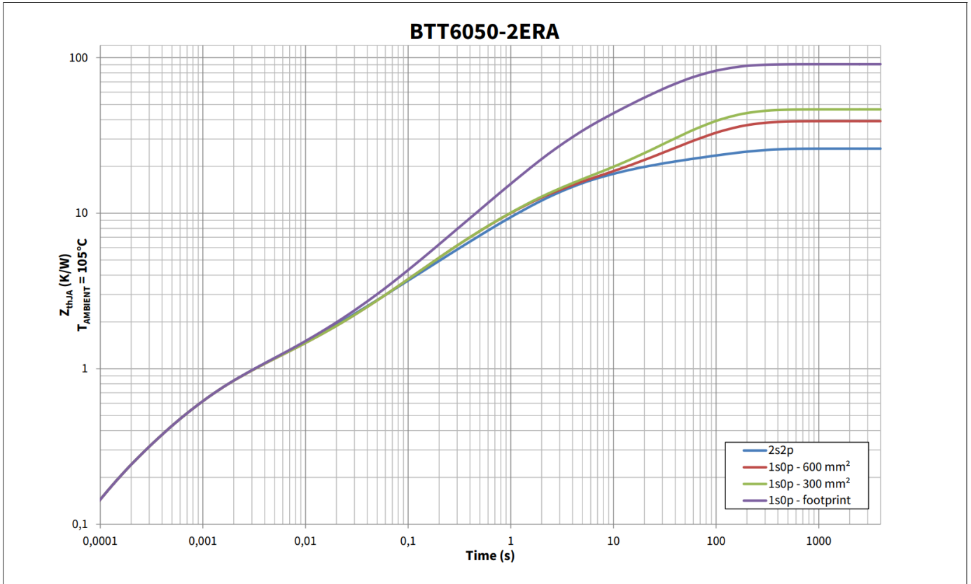
图 6 典型热阻抗- 2s2p 设置如图 4
