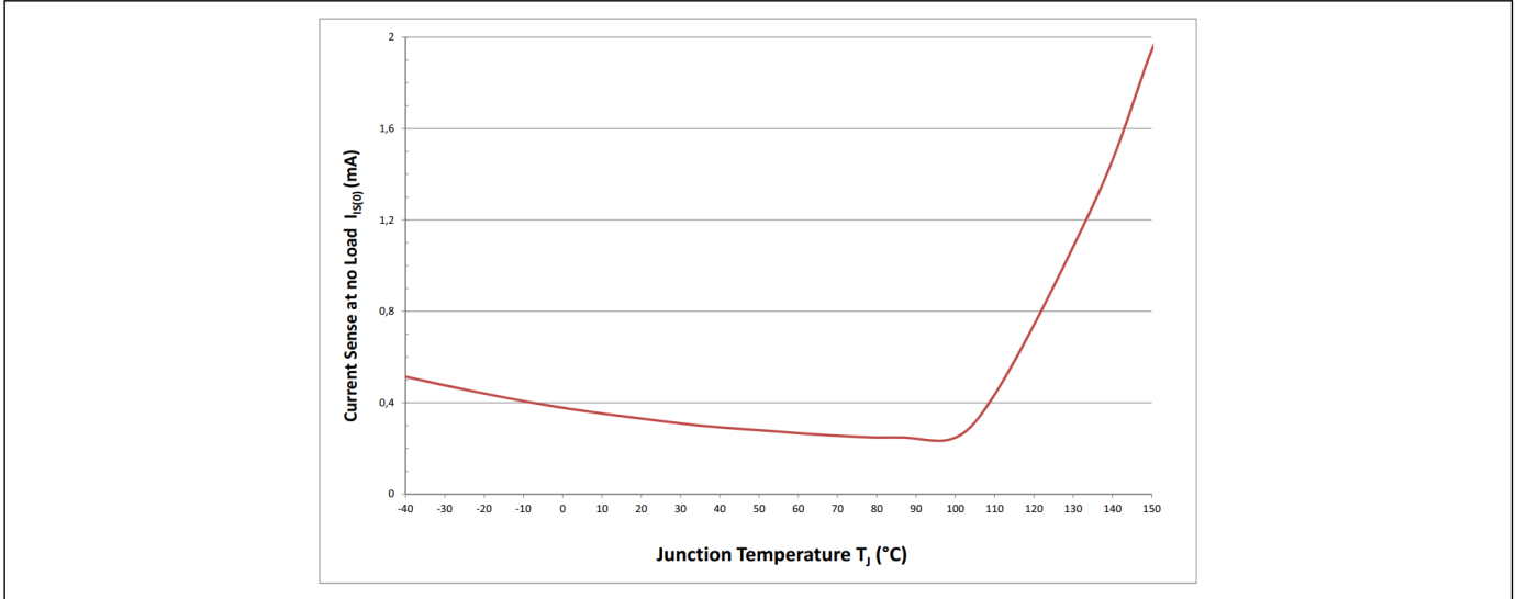
图 45 空载电流检测 I_{L(OL)} = f(T_J; V_S), I_L = 0 A
