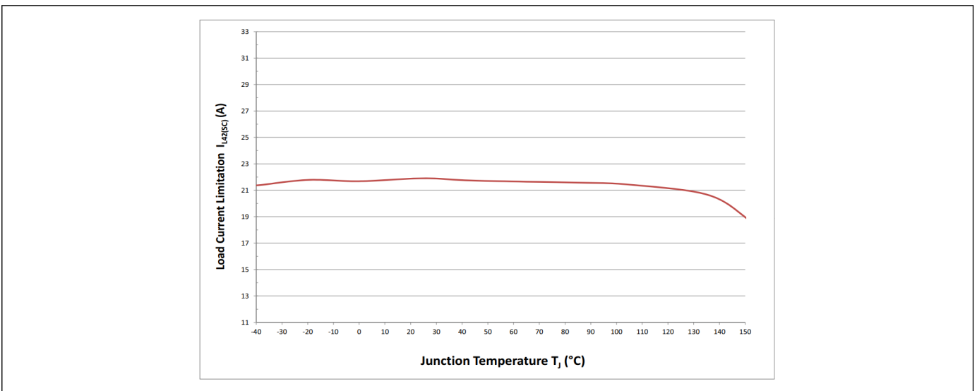
图 44 高压区过载条件 I_{L28(SC)} = f(T_j; V_s)
