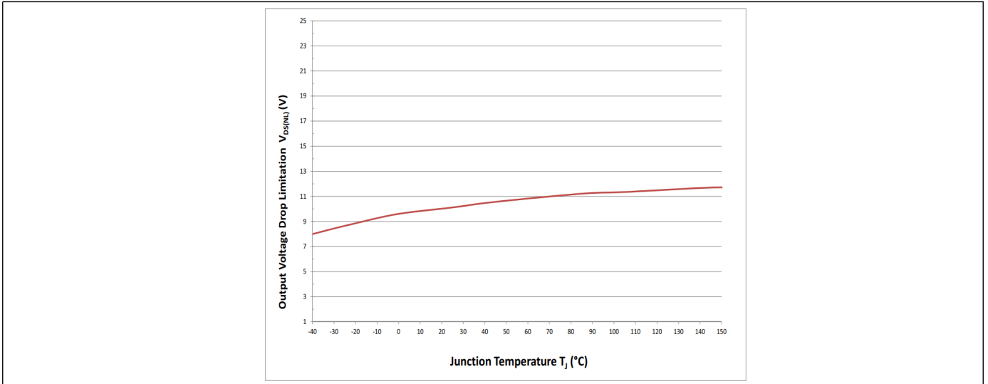
图 34 低负载电流时的输出电压降限制 V_{DS(NL)} = f(T_J; V_S) ; I_L = I_{L(0)} = 50 \text{ mA}
