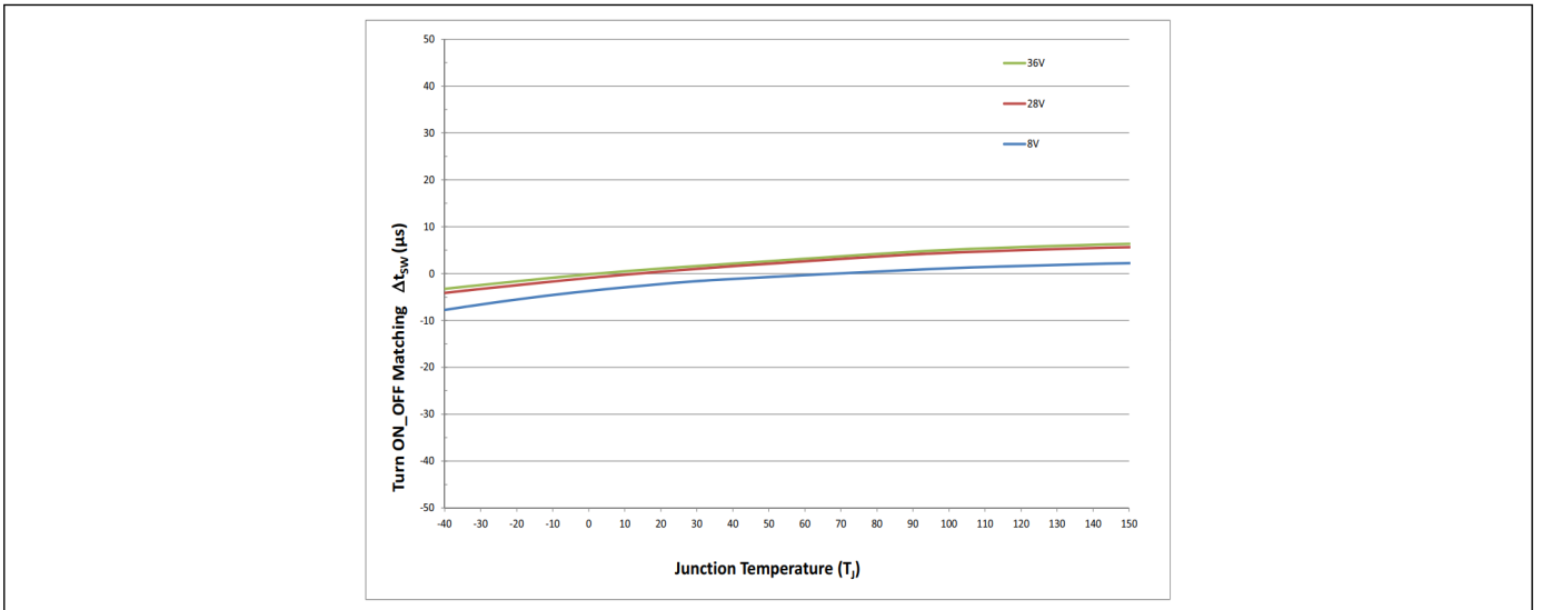
图 40 开启/关断匹配 \Delta t_{SW} = f(T_j; V_s) , R_L = 12\Omega
