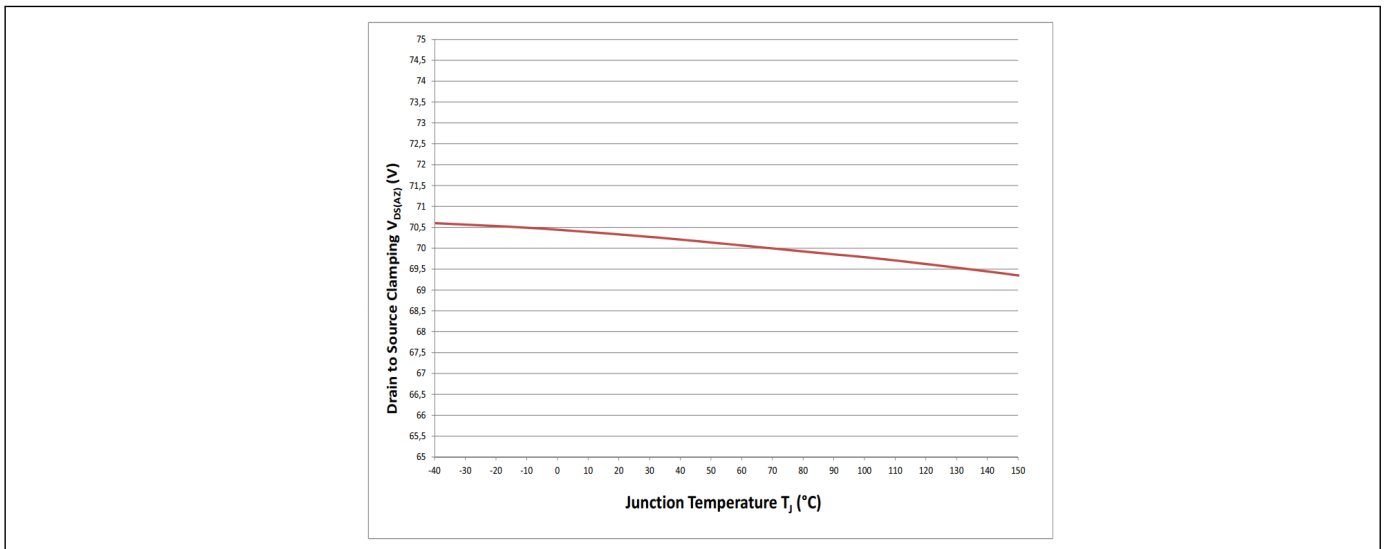
图 35 漏源钳制电压 V_{DS(AZ)} = f(T_J)
