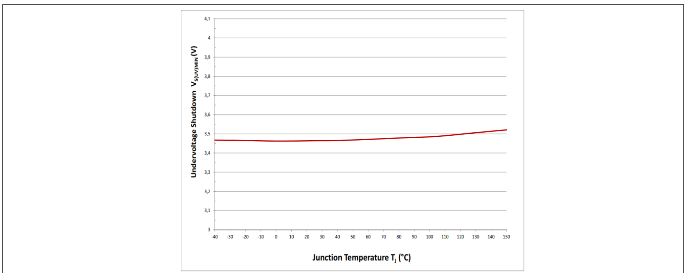
图 30 欠压阈值 V_{S(UV)} = f(T_j)
