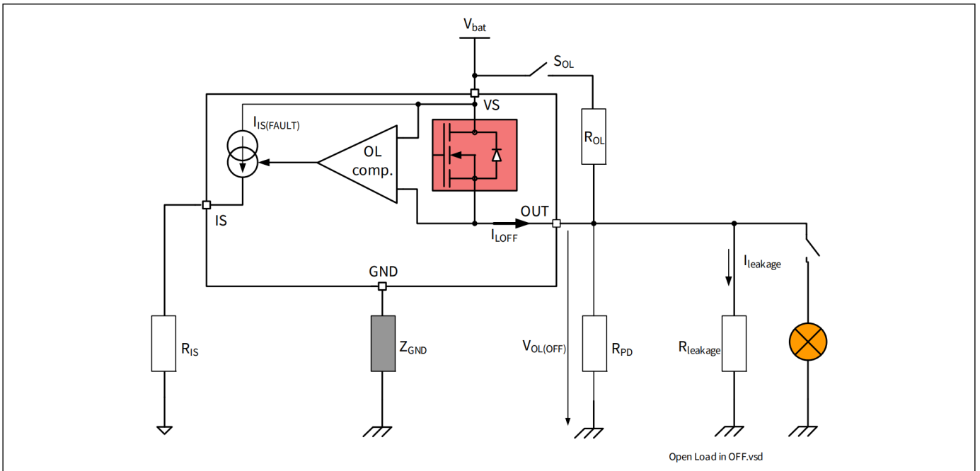
图25 负载开路OFF电气等效电路检测
