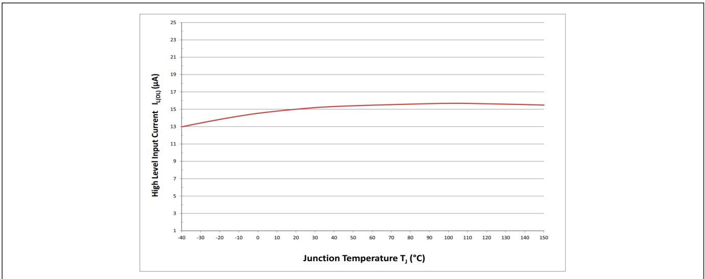
图 52 输入电流高电平 I_{IN(H)} = f(T_J; V_S)
