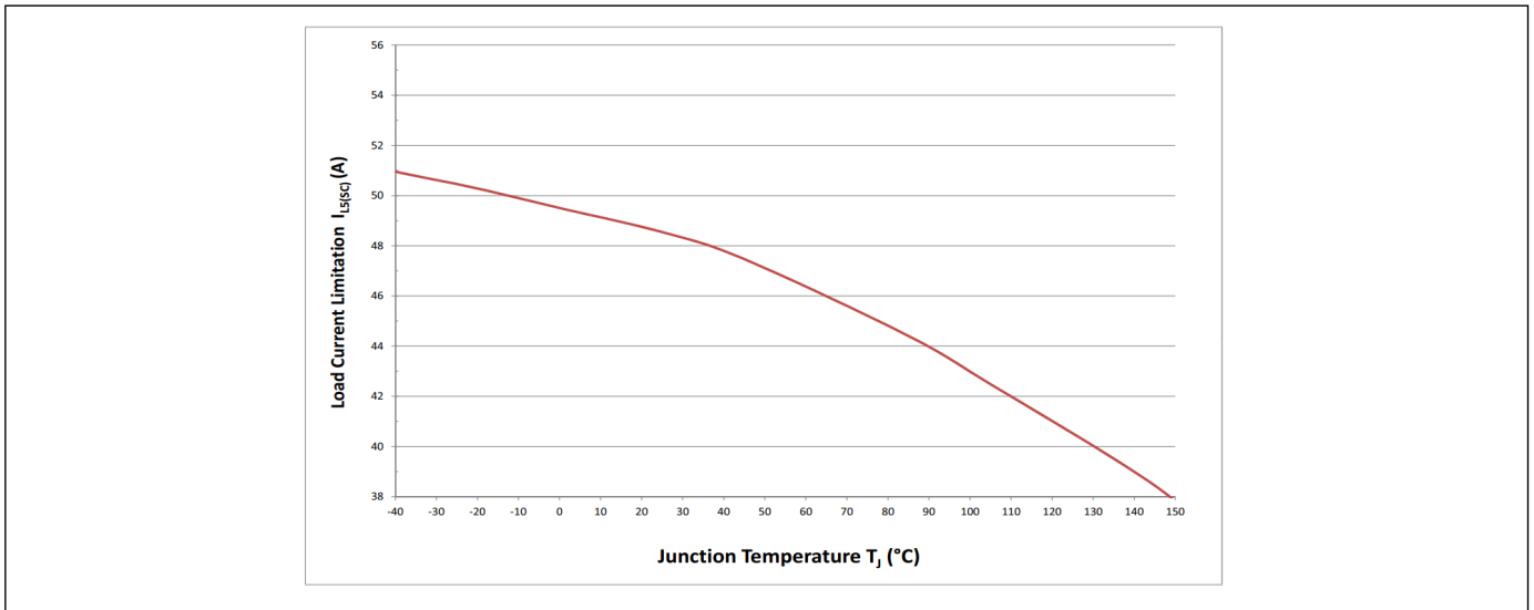
图43 低压区过载条件 I_{L5(SC)} = f(T_j; V_s)
