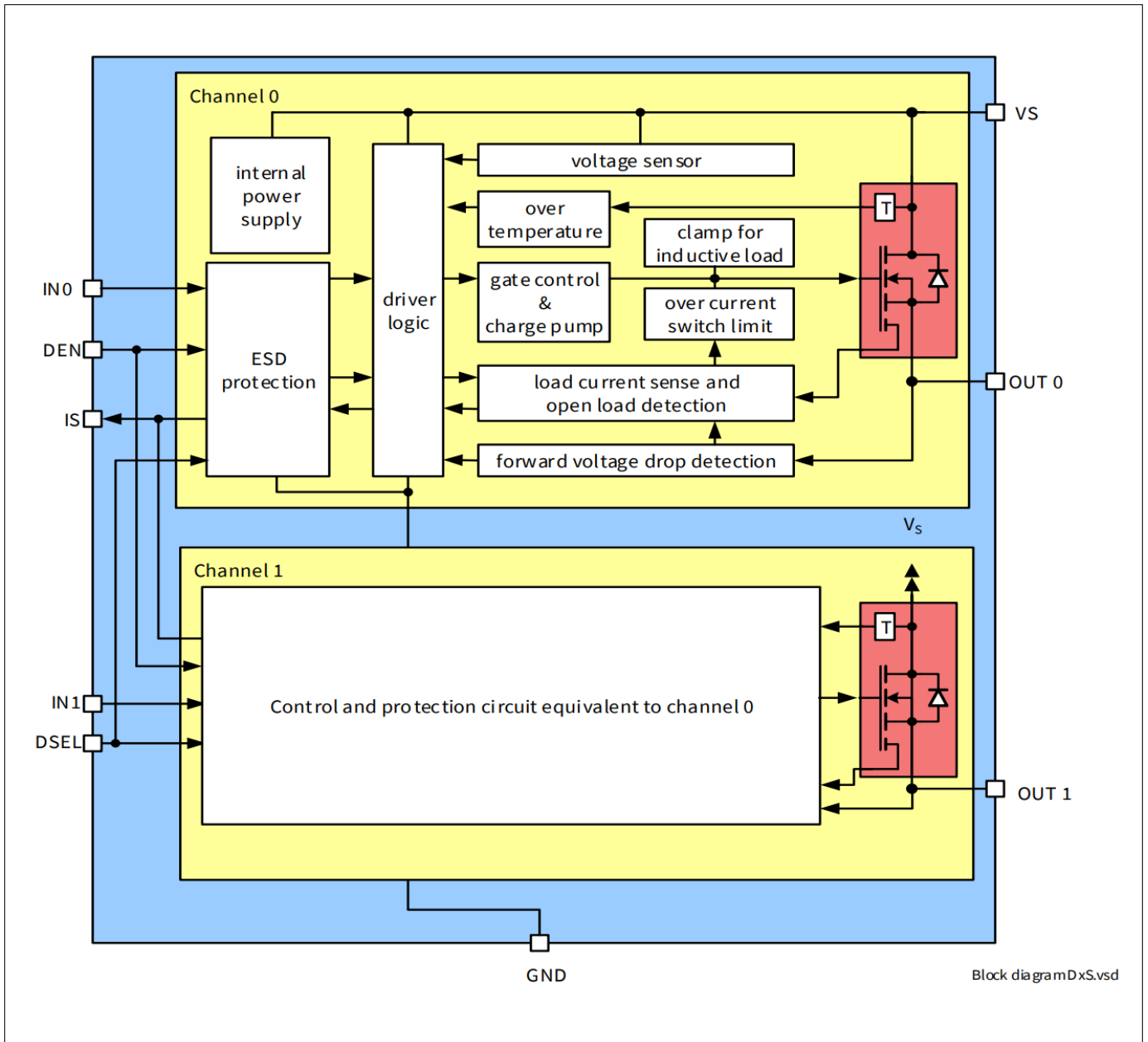
图 1 BTT6050-2ERA 框图
