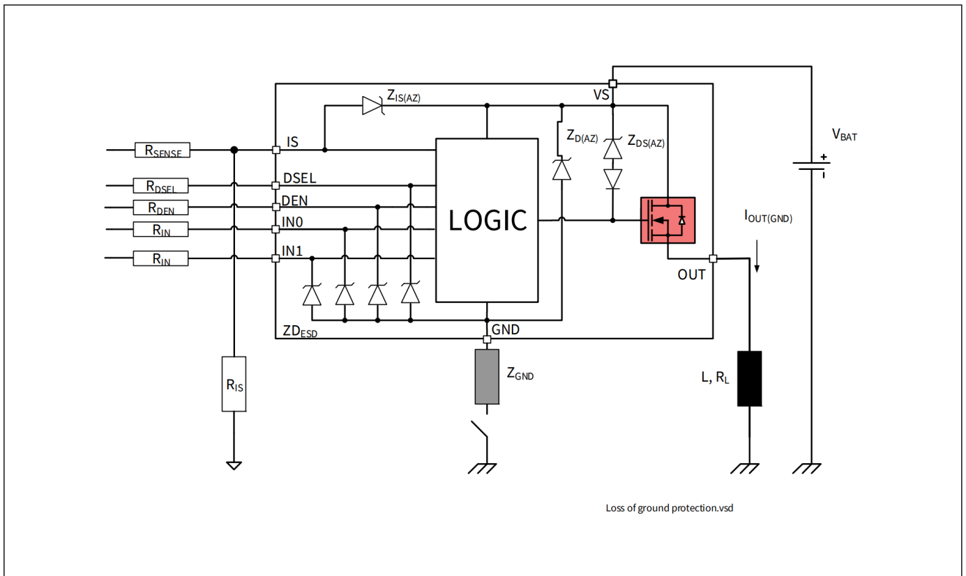
图 14 与外部元件的接地丢失保护
