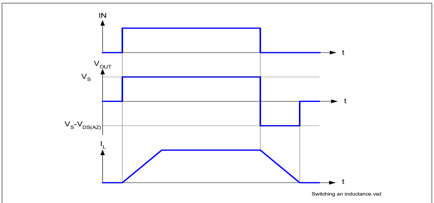
图 11 开关感性负载时序
