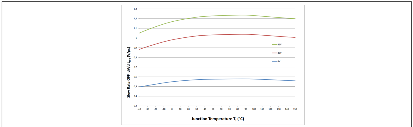
图 37 关断时间斜率 - dV/dt_{OFF} = f(T_j; V_s), R_L = 12\Omega
