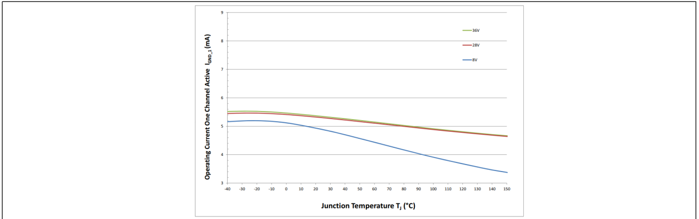
图 31 整个器件带负载的电流损耗。单通道有效 I_{GND\_1} = f(T_J; V_S)
