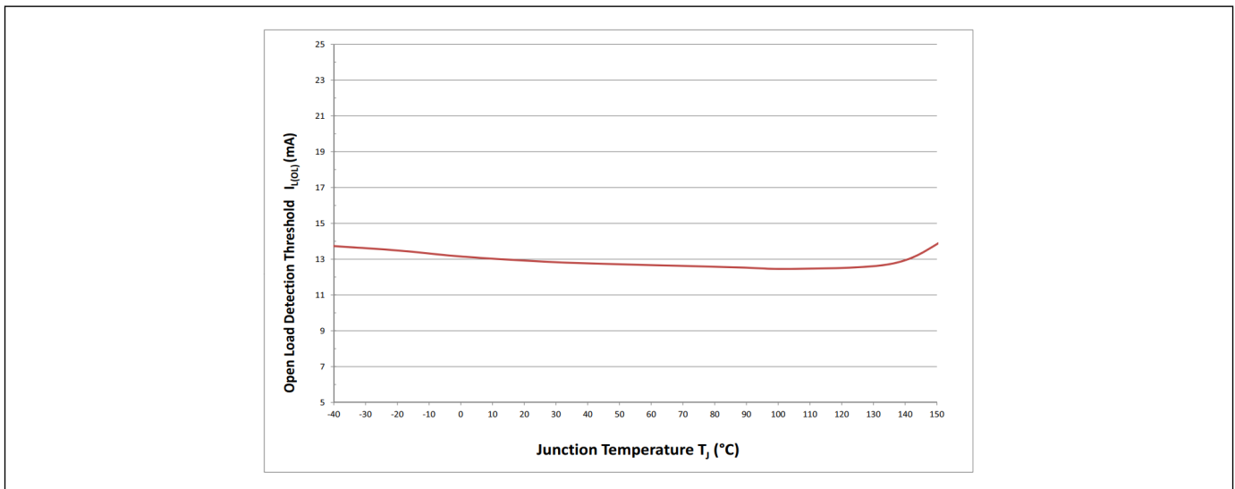
图 46 ON 状态负载开路检测阈值 I_{L(OL)} = f(T_J; V_S)
