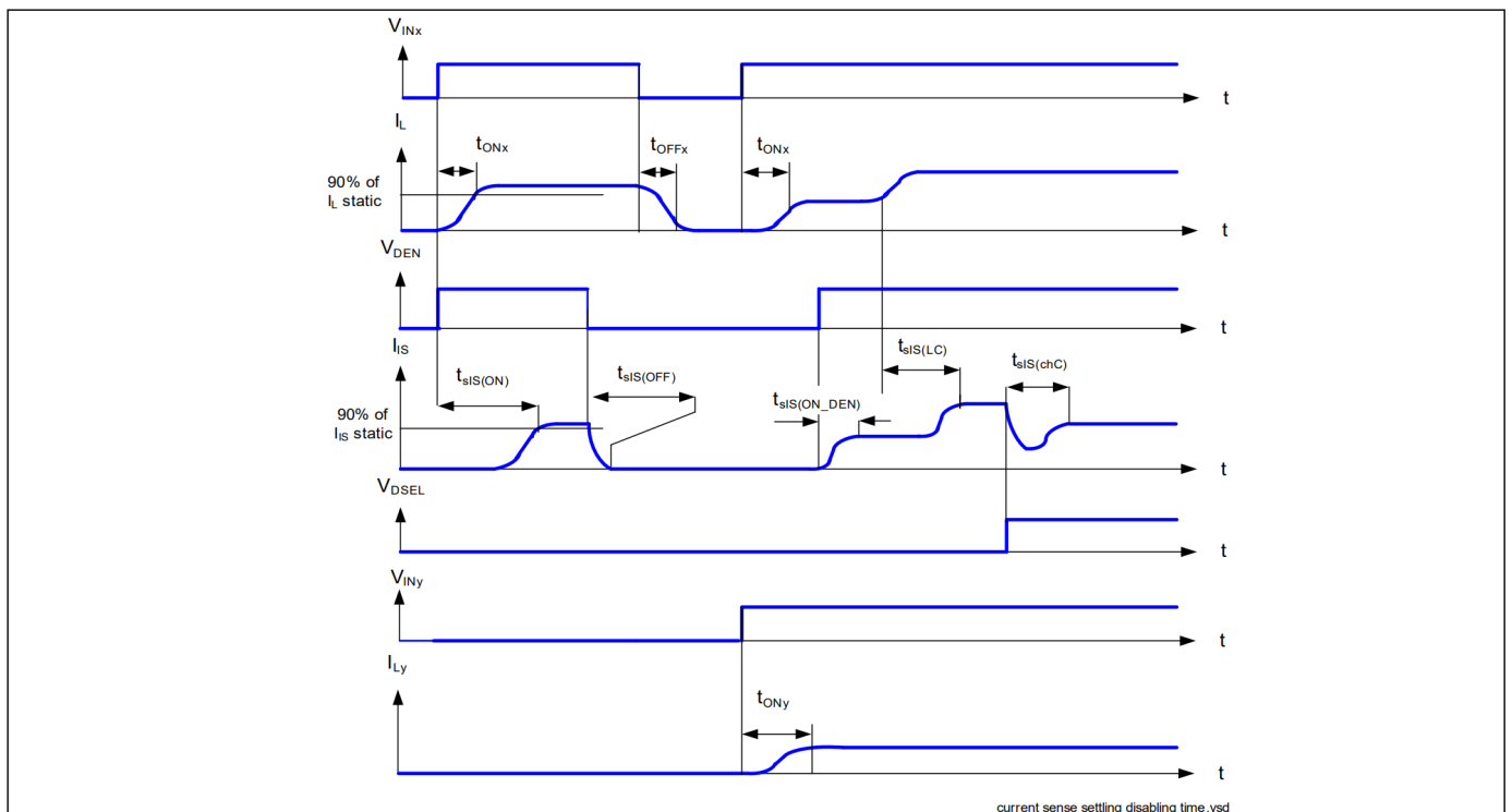
图23 Sense设置/失效时序
