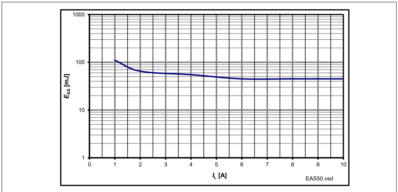
图 12 单脉冲最大能量耗散, T_{J(0)} = 150^\circ\text{C} ; V_S = 28 \text{ V}
