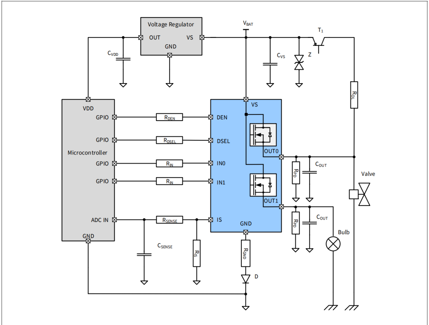
图 53 BTT6050-2ERA 应用图
