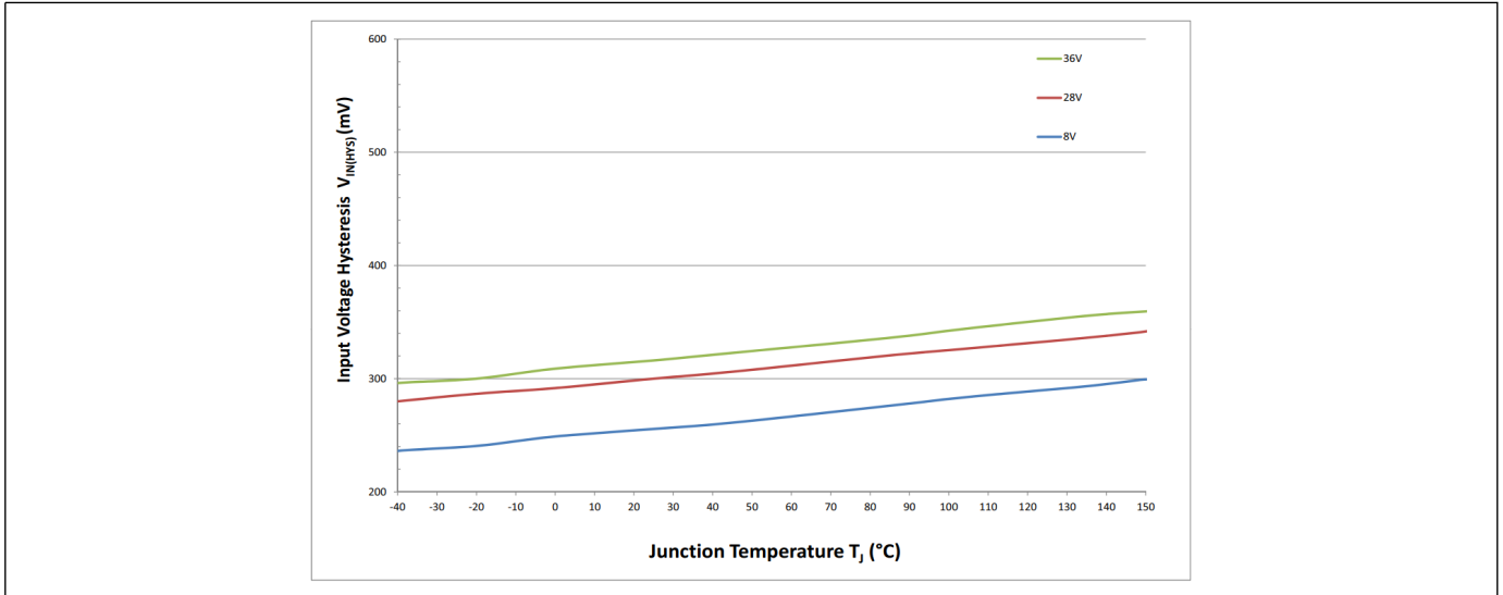
图 51 输入电压滞回区 V_{IN(HYS)} = f(T_J; V_S)
