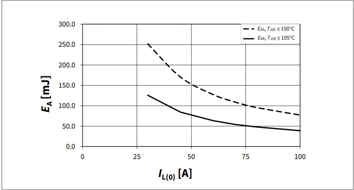
图 6 关断电感负载最大能量耗散, E_{AS/AR} vs. I_L at V_S = 13.5\text{ V}
