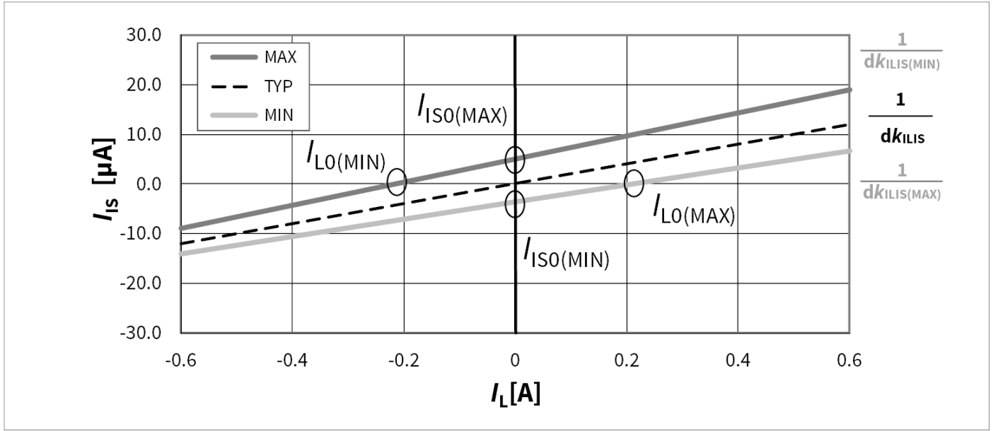
图 22 I_{iso} 和 I_{Lo} 定义
