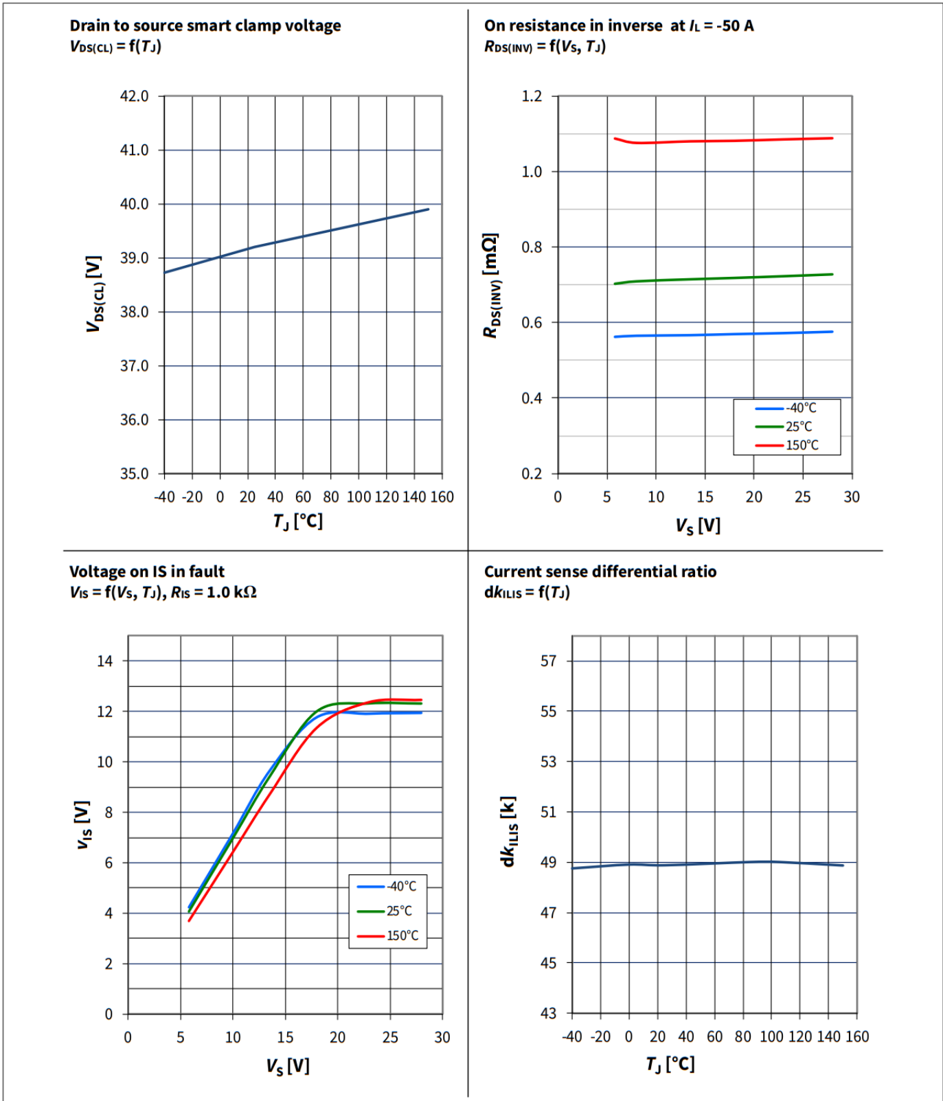
图 30 典型性能特性 (续)
