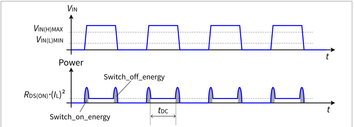
图 10 PWM 开关
