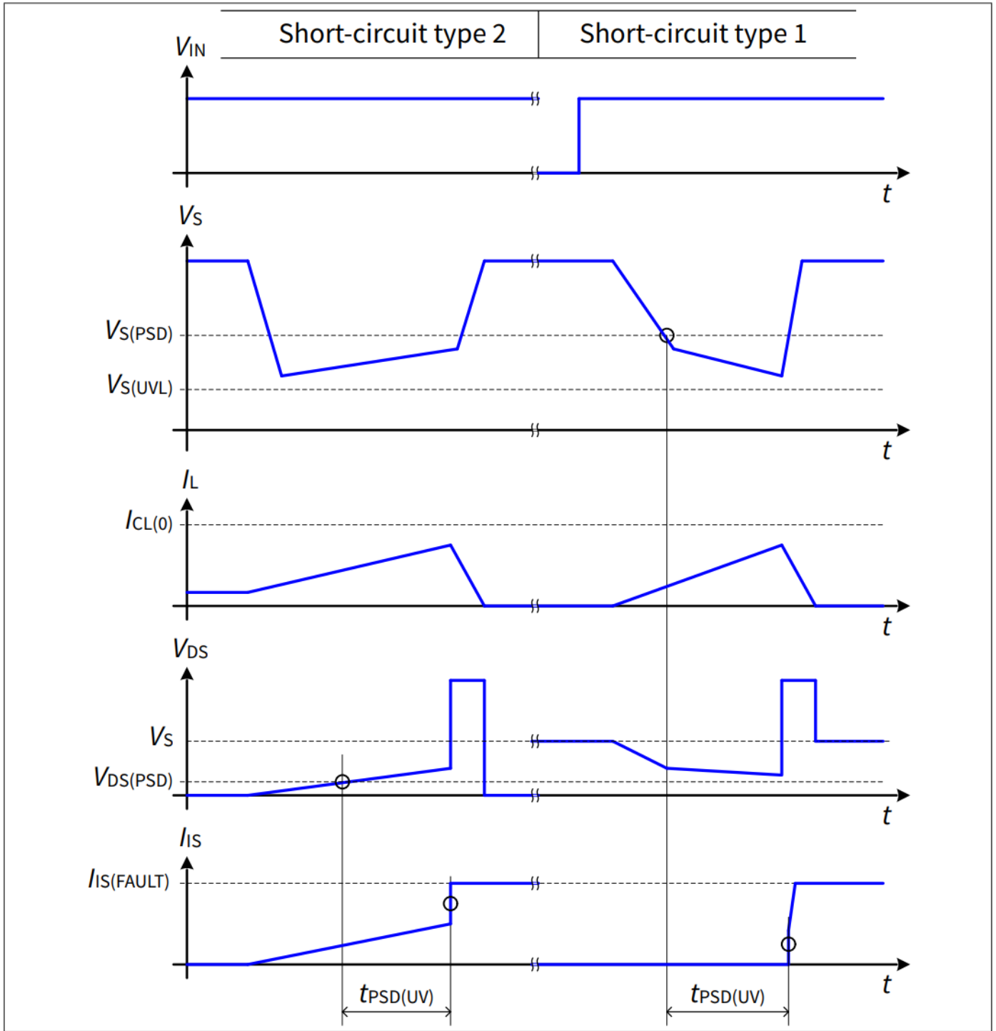
图 17 供电电压下降期间的过功率关断行为
