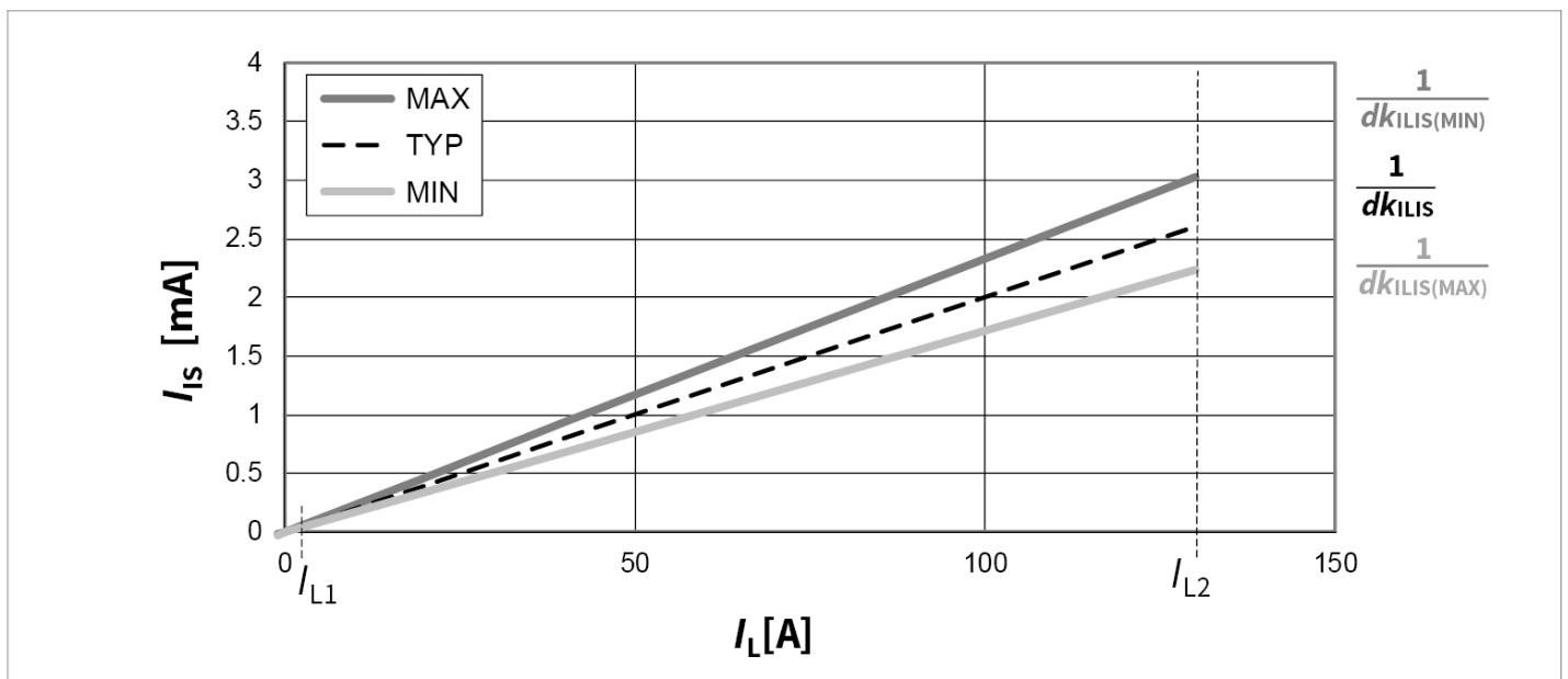
图 21 IS 引脚的电流检测与负载电流的关系
