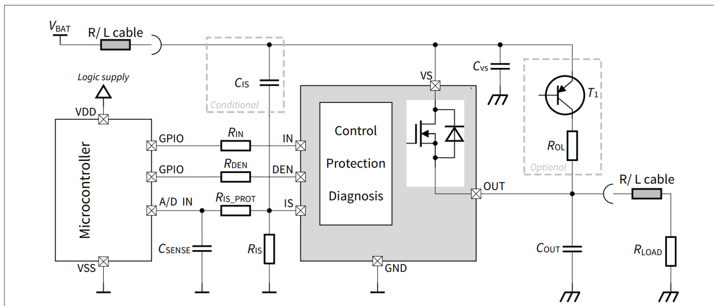
应用框图
