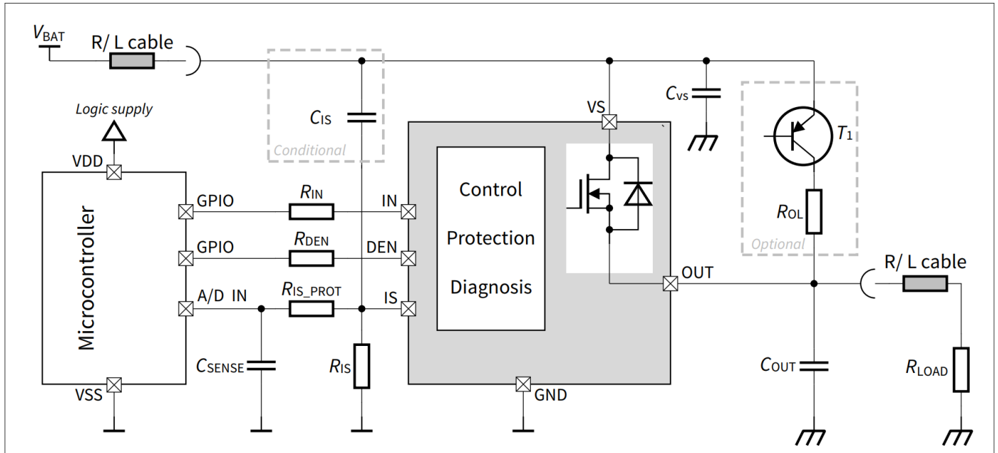
图 32 应用图：由微控制器控制的器件
