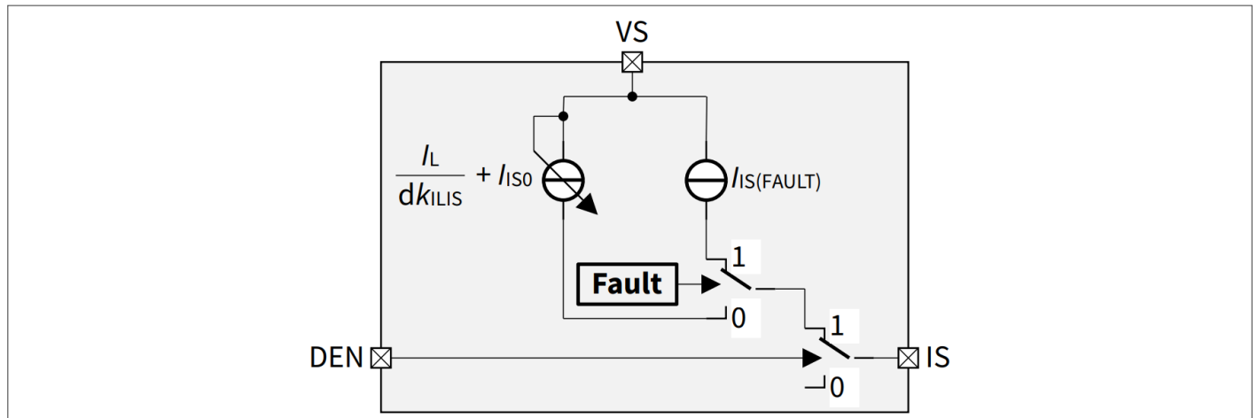
图 19 检测功能框图
