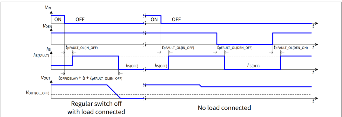
图 26 连接负载和未连接负载时负载开路检测的行为关闭特性
