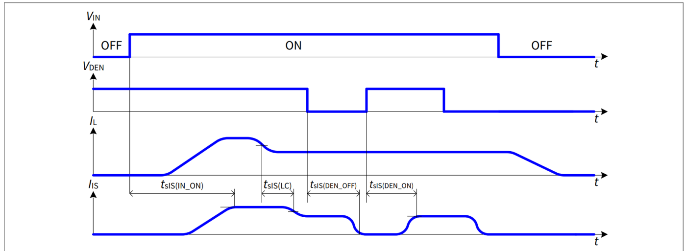
图 24 正常运行时电流检测时序
