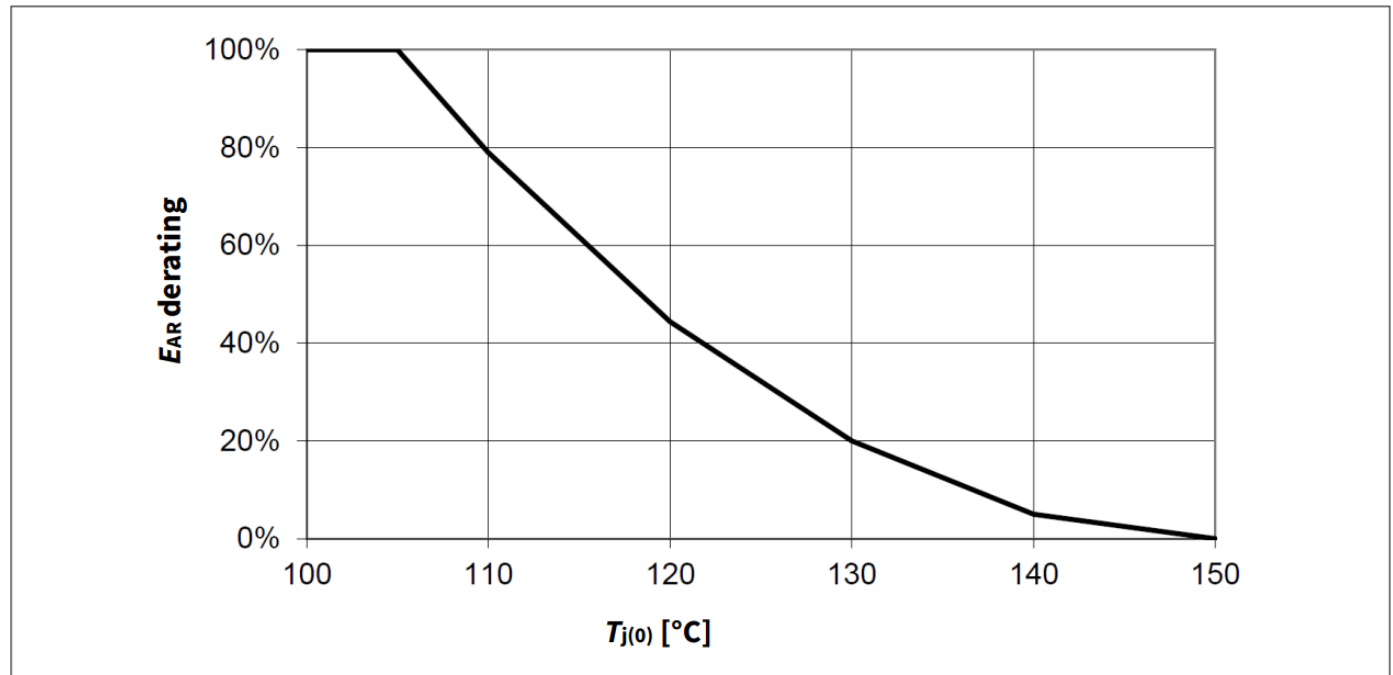
图 7 重复的脉冲温度降额最大能量耗散
