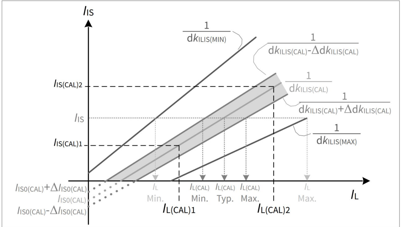
图 23 通过2个校准点提高电流检测精度
