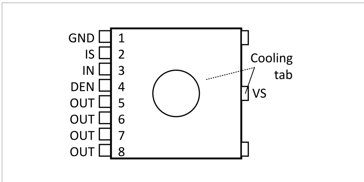
图 5 引脚分配
