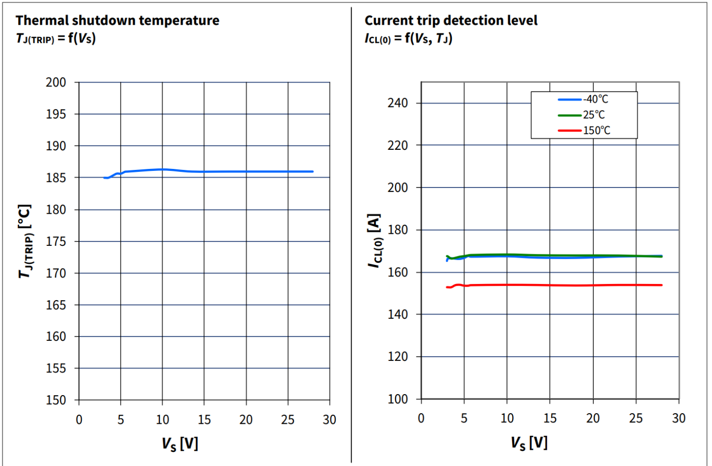
图 31 典型性能特性 (续)
