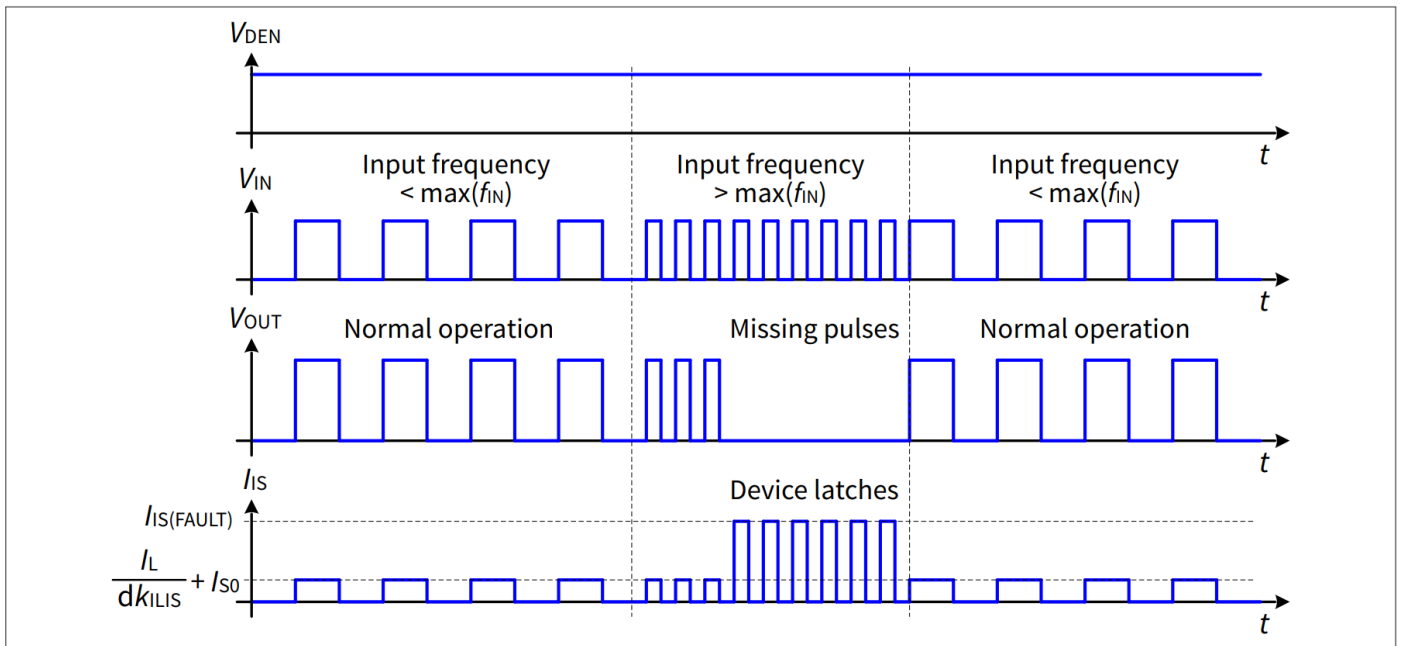
图 16 PWM 操作期间 f_{IN} 最大值以上的行为
