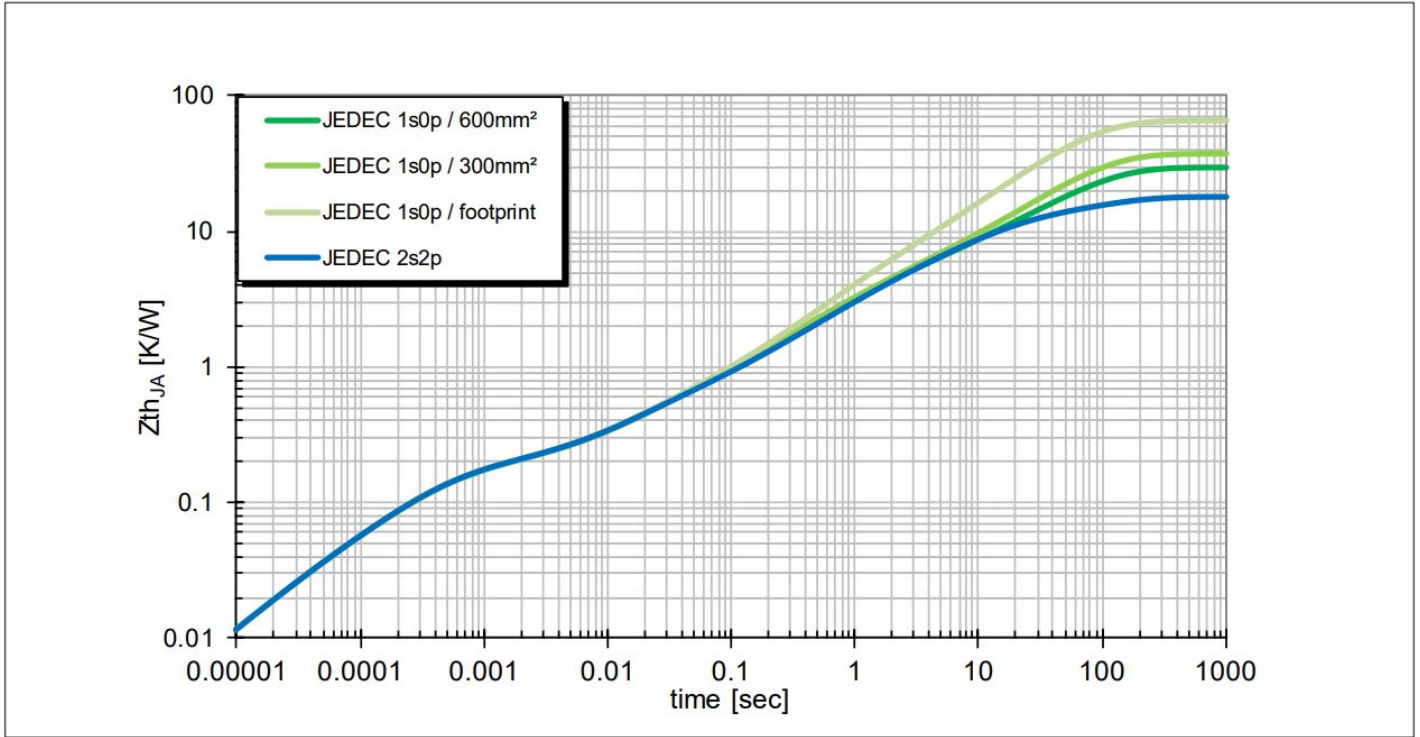
图 8 不同 PCB 条件下的典型瞬态热阻抗 Z_{th(JA)} = f(\text{time})
