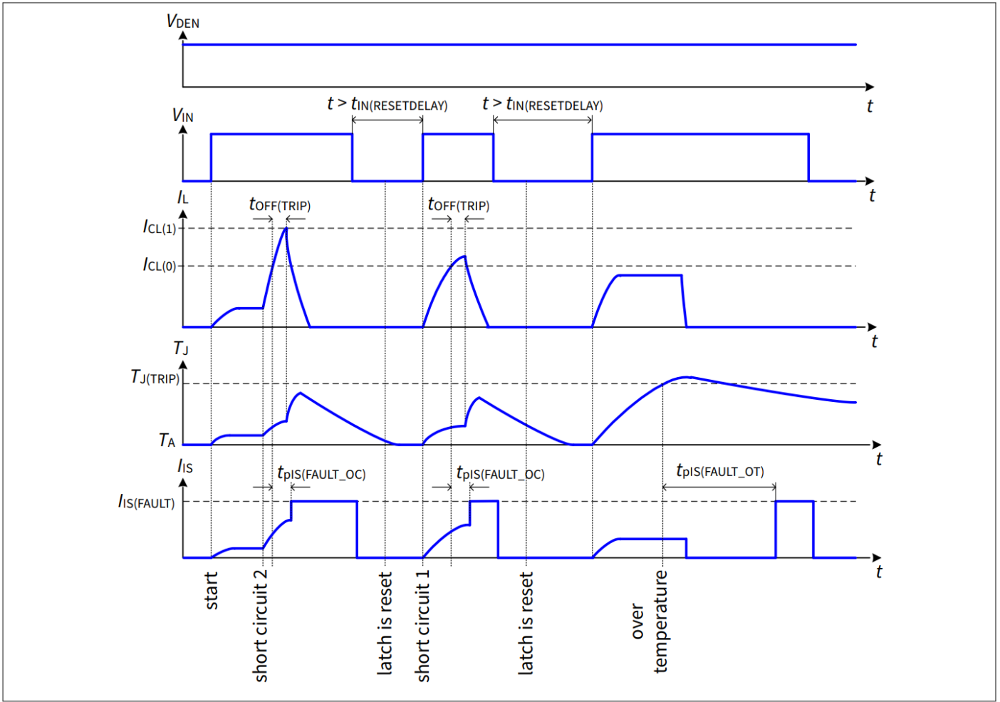
图 25 保护状态下的 IS 引脚行为
