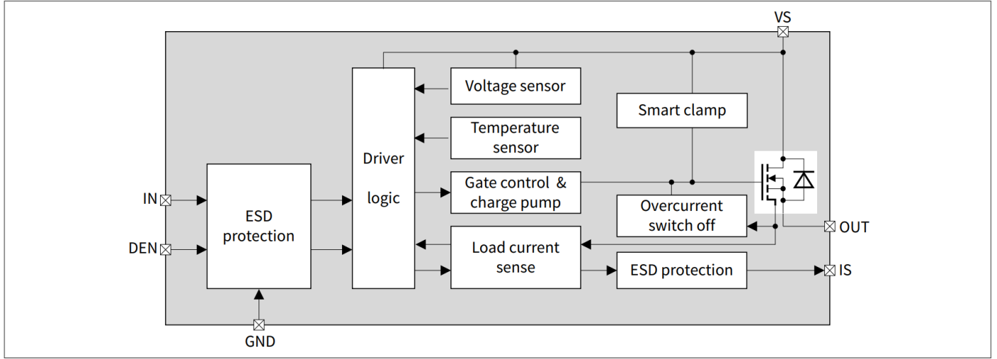
图 2 框图
