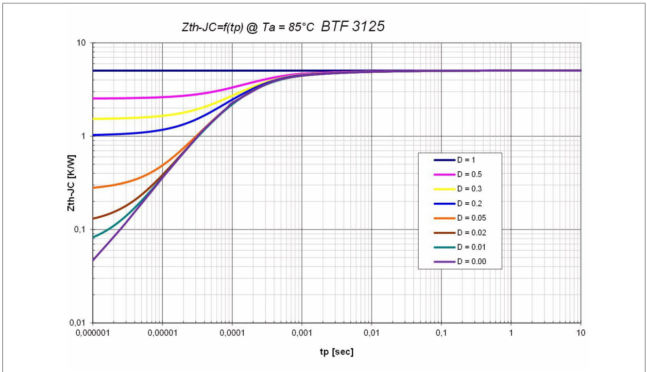
图 8 Z_{th(JC)} 与占空比的关系
