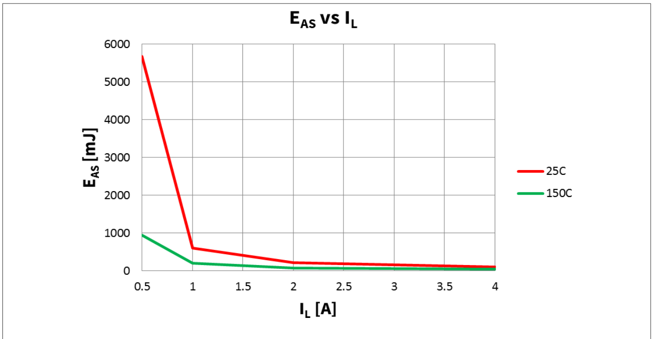
图 29 E_{AS} 与 I_L @ T_{J(0)} = 25^\circ C, 150^\circ C, V_{BAT} = 13.5V ; V_{IN} = V_{ENABLE} = V_{DD} = 开路; I_L = I_{L(NOM)}/4, I_{L(NOM)}/2, I_{L(NOM)}, 2 * I_{L(NOM)}
