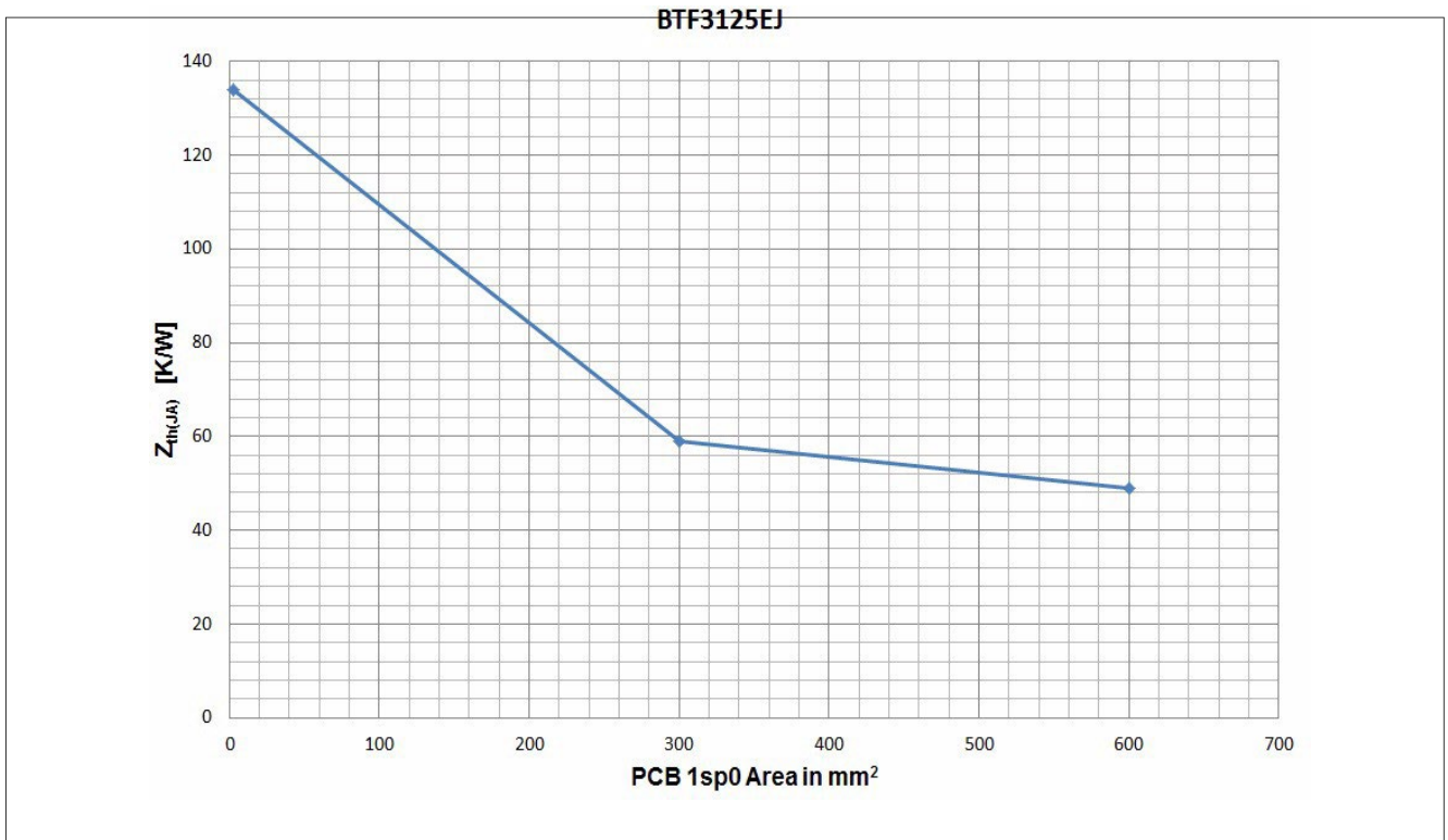
图 9 PCB 1sp0 - R_{thja} 与冷却区域
