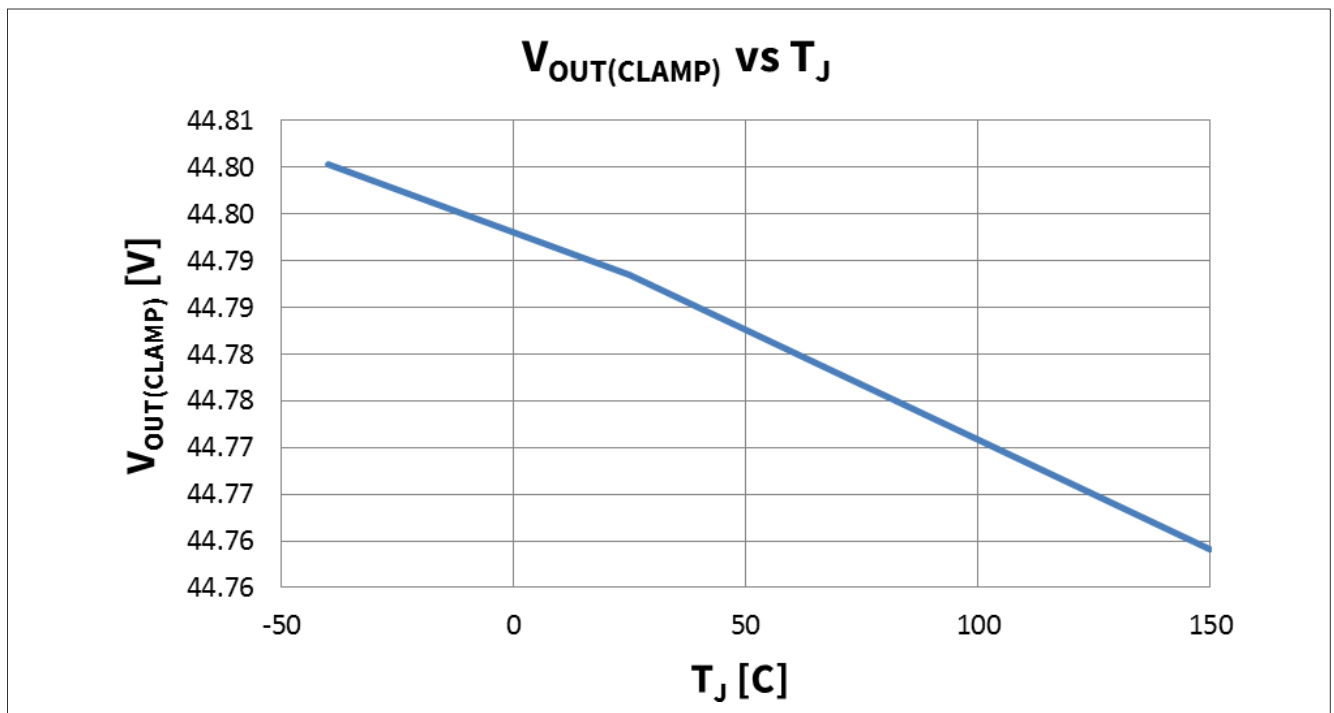
图 40 V_{OUT(clamp)} vs. T_J ; V_{IN}=0V ; V_{ENABLE}=V_{DD}=5V ; I_L=4mA
