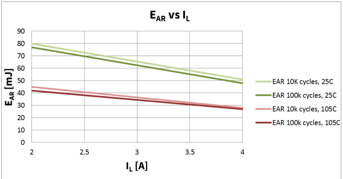
图 30 E_{AR\_10k, \_100k} 与 I_L @ T_{J(0)}=25^{\circ}\text{C}, 105^{\circ}\text{C}, V_{BAT}=13.5\text{V}; V_{IN}=V_{ENABLE}=V_{DD}=5\text{V}; I_L=I_{L(NOM)}, 2*I_{L(NOM)}
