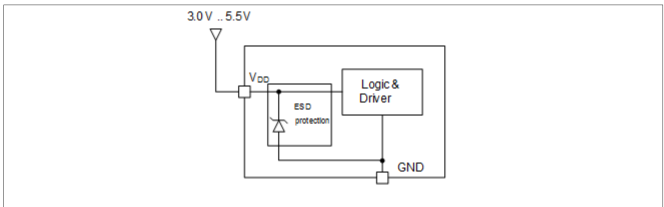
图 21 电源电路
