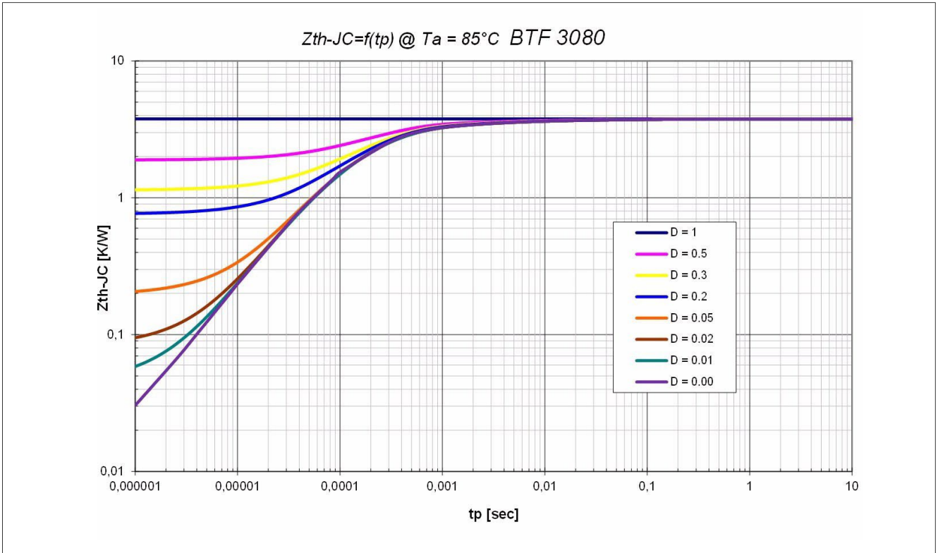
图 8 Z_{th(JC)} 与占空比的关系
