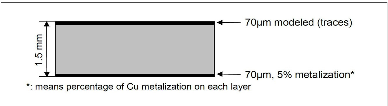
图 5 JEDEC1s0p 横截面
