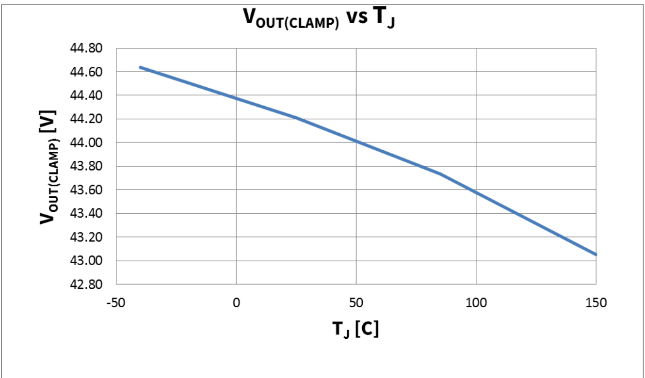
图 40 V_{OUT(clamp)} vs. T_J ; V_{IN}=0V ; V_{ENABLE}=V_{DD}=5V ; I_L=6mA
