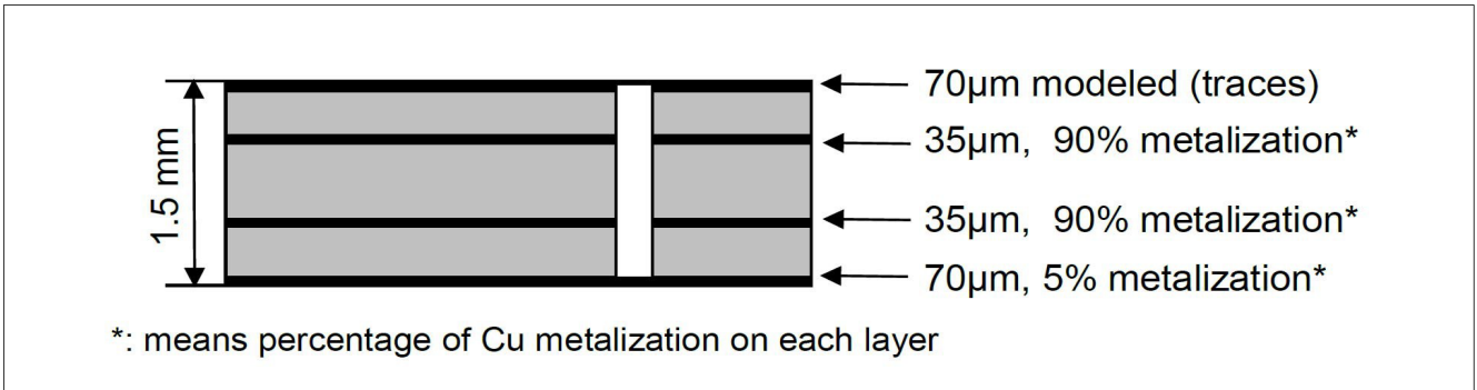
图 4 JEDEC2s2p 横截面
