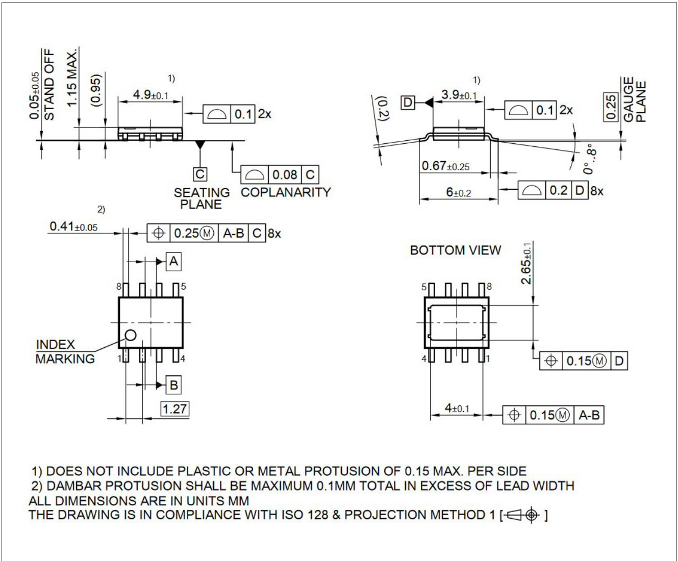
图 52 PG-TDSO-8-31 1)
