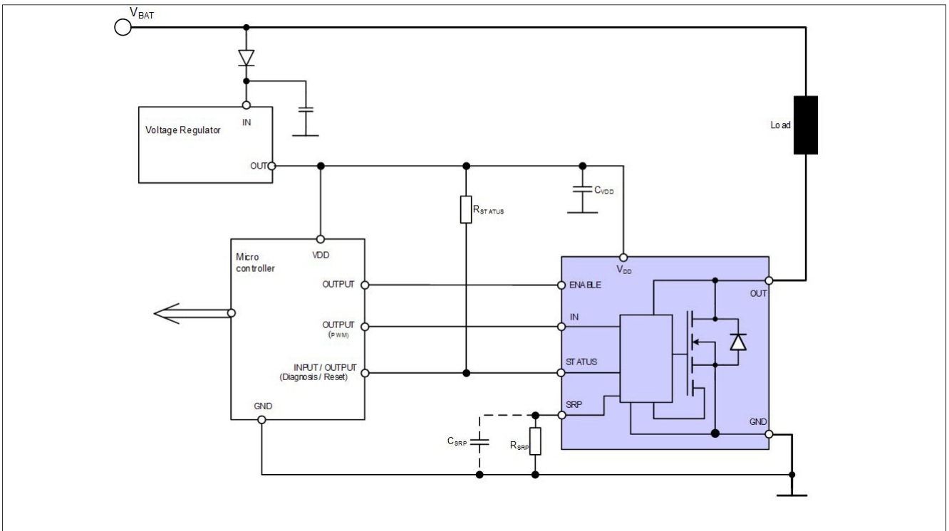
图51 简化应用框图
