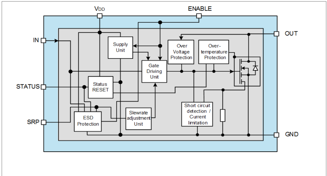
图 1 框图
