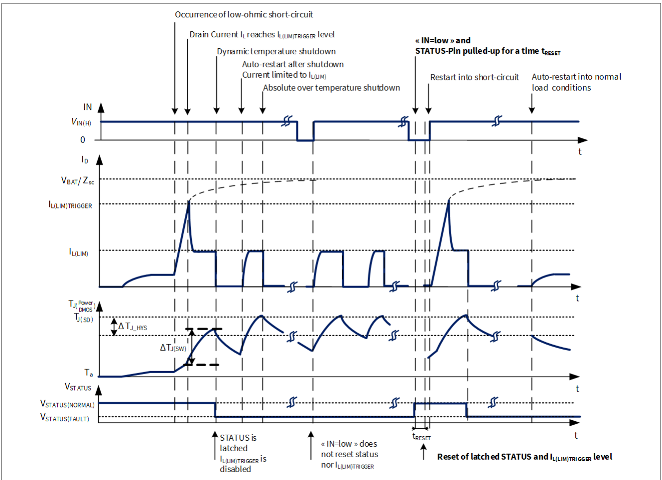
图 18 通过电流限制和热关断实现短路保护，并在 STATUS 上锁存故障信号
