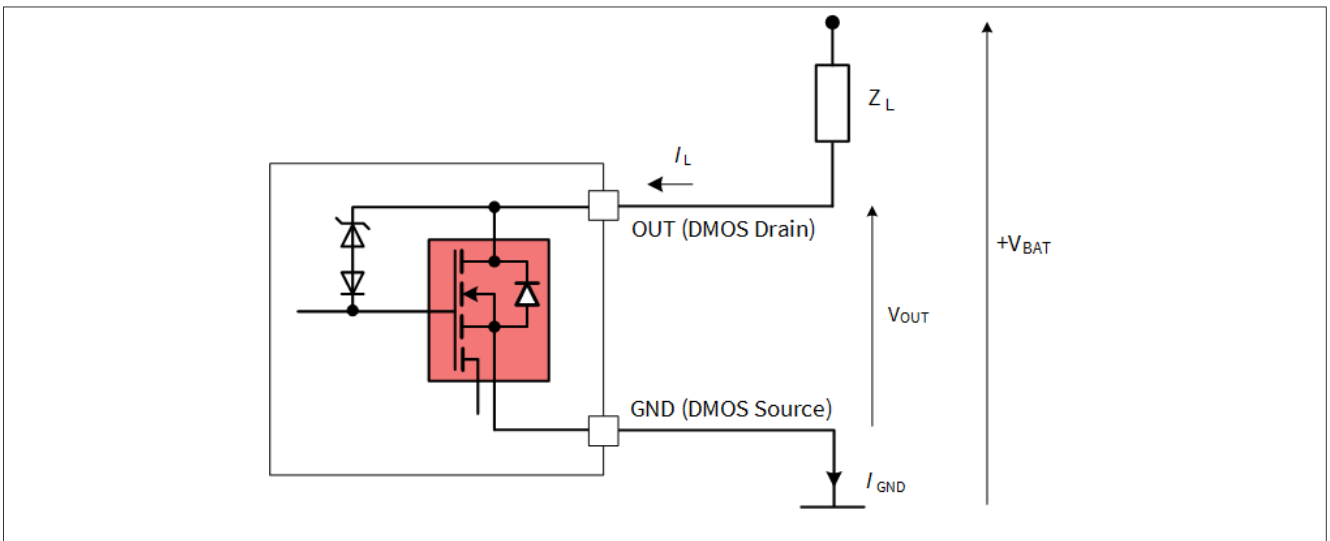
图 13 输出钳位电路
