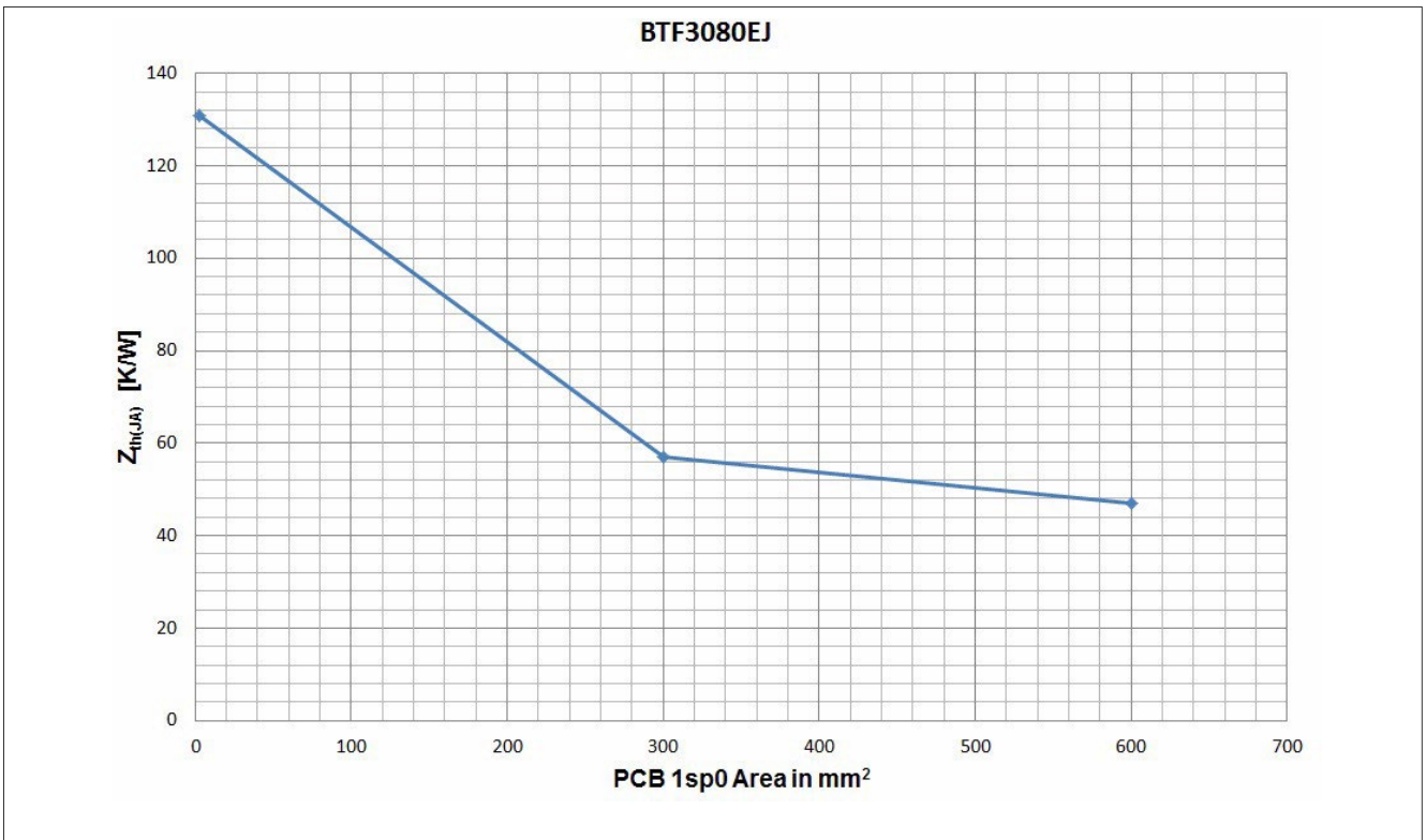
图 9 PCB 1sp0 - R_{thja} 与冷却区域
