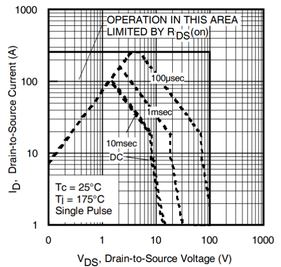
图 8.最大安全工作区
