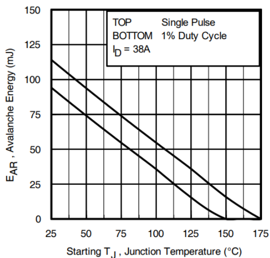
图 16.最大雪崩能量与温度的关系曲线
