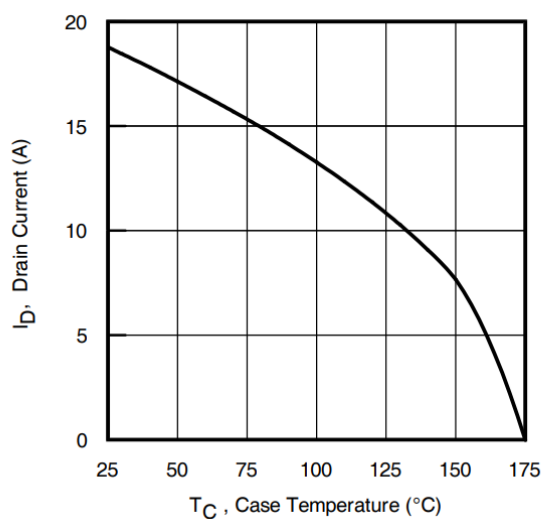
图 9.最大漏极电流与壳温的关系曲线
