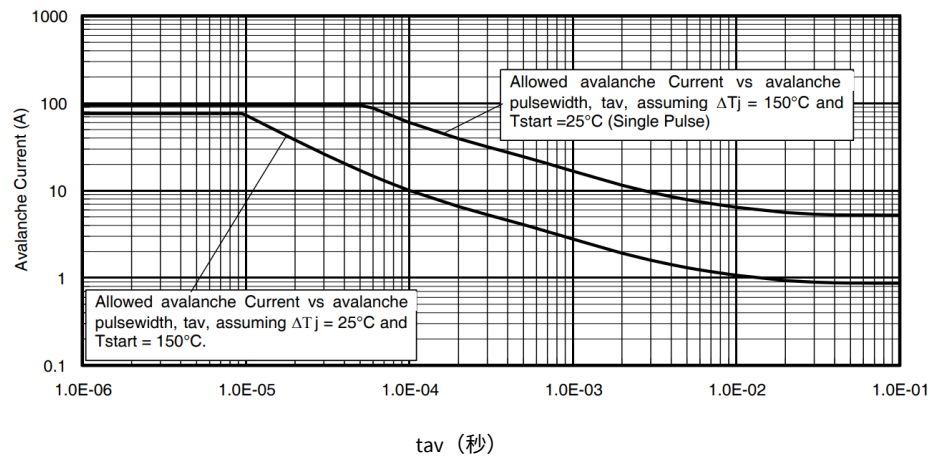
图 14.典型雪崩电流与脉冲宽度的关系曲线
