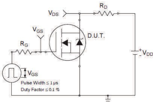
图 23a. 开关时间测试电路
