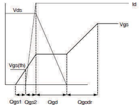
图 24b. 阻抗充电波形
