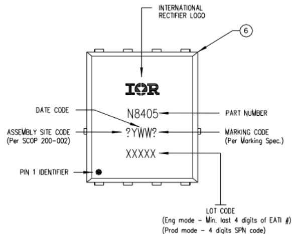
TOP MARKING (LASER)
