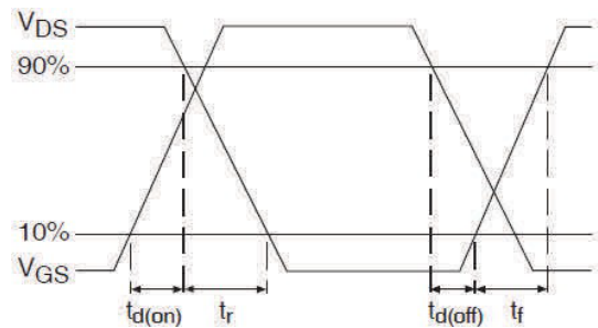
图 23b. 开关时间波形
