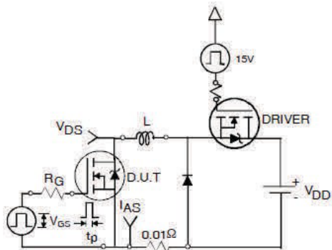
图 22a. 未钳位电感测试电路
