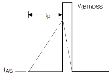
图 22b. 未钳位电感波形
