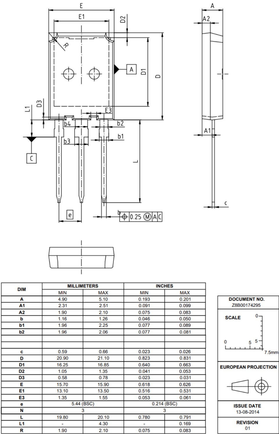
封装图 PG-TO247-3-46
