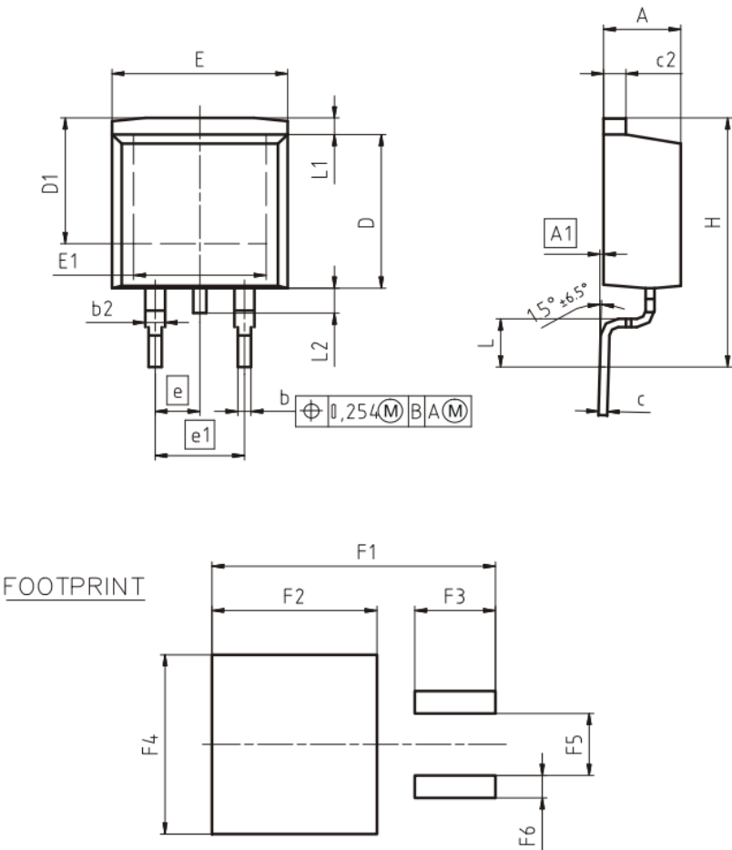
封装图 PG-T0263-3
