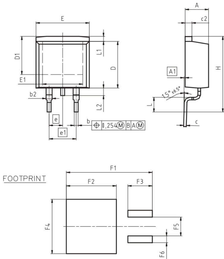
封装图 PG-T0263-3
