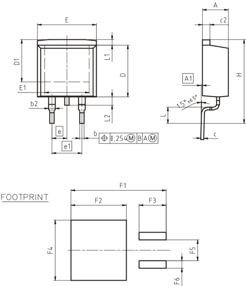
封装图 PG-T0263-3
