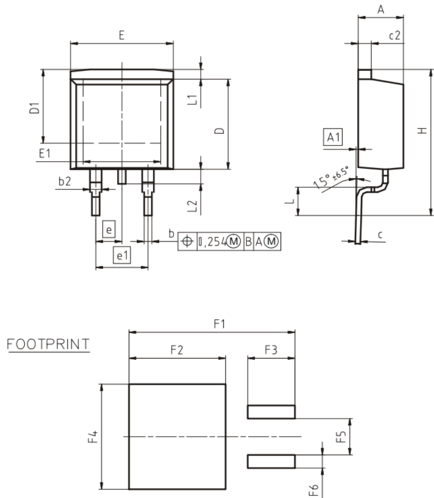
封装图 PG-T0263-3
