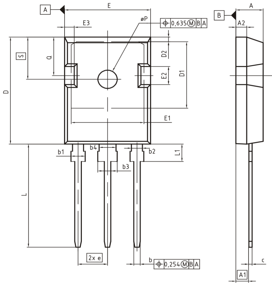
封装图 PG-TO247-3
