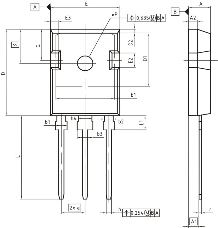
封装图 PG-T0247-3
