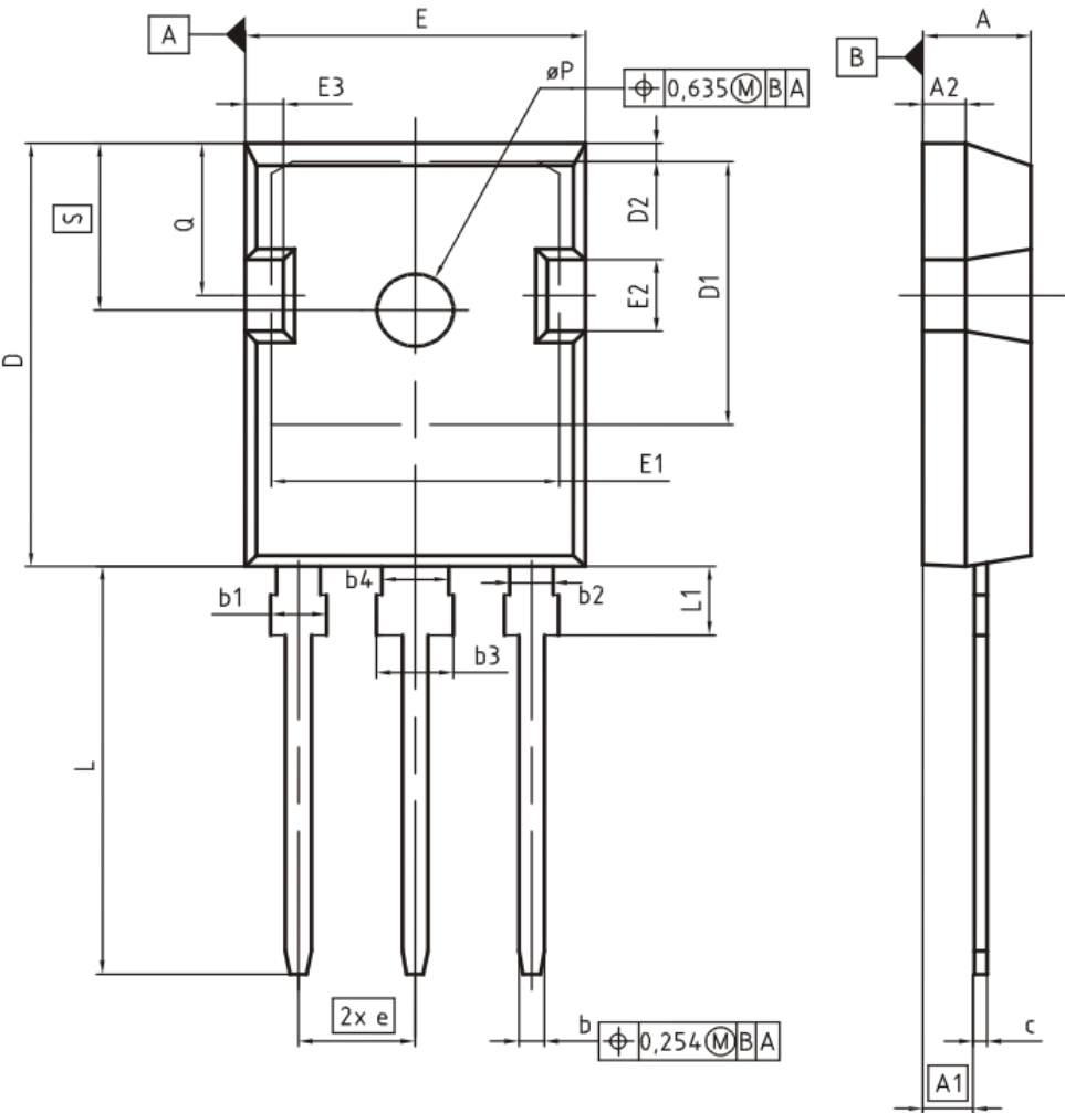
封装图 PG-T0247-3
