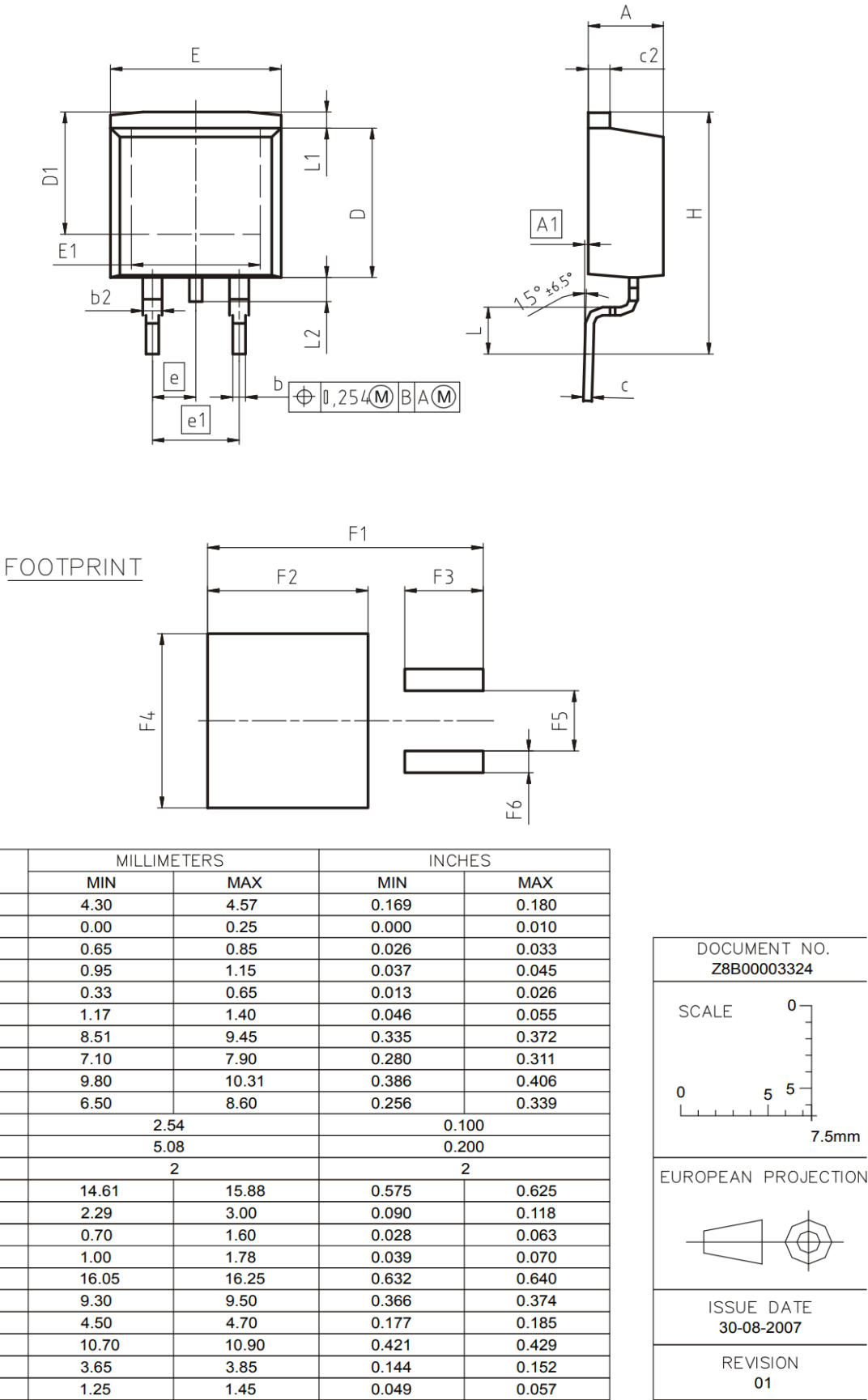
封装图 PG-T0263-3
