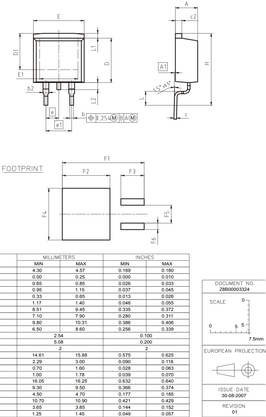
封装图 PG-T0263-3
