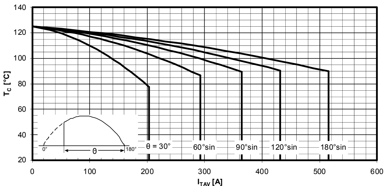
Höchstzulässige Gehäusetemperatur / Maximum allowable case temperature T_C = f(I_{TAV})
